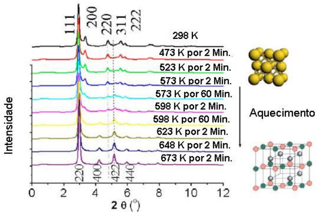
Figura 8: Retirada da ref. [39], evolução da transição de fase estrutural da liga \text{Ni}_2\text{MnGa} em função da temperatura e tempo do tratamento térmico empregado.
