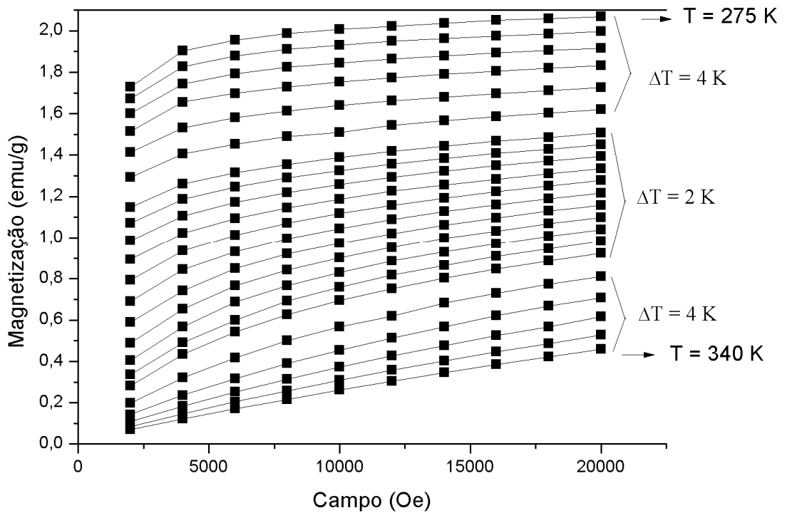
Figura 33: Magnetização em função do campo aplicado para amostras moídas durante 6 h e tratada termicamente durante 4 h a 1123 K.
