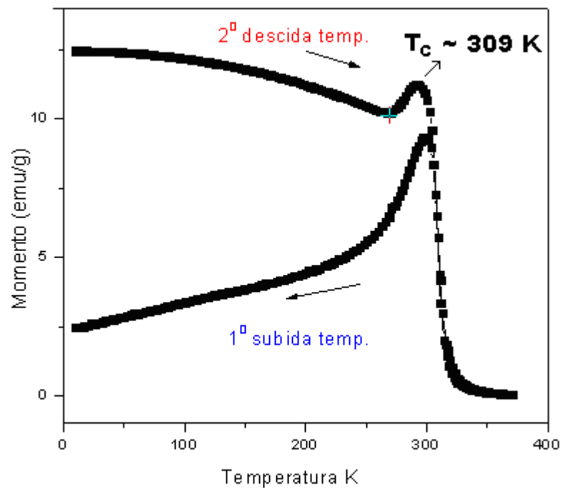
Figura 29: Curvas de magnetização em função da temperatura durante aquecimento e resfriamento para amostra moída durante 6 h e tratada termicamente a 1123 K durante 4 h.
