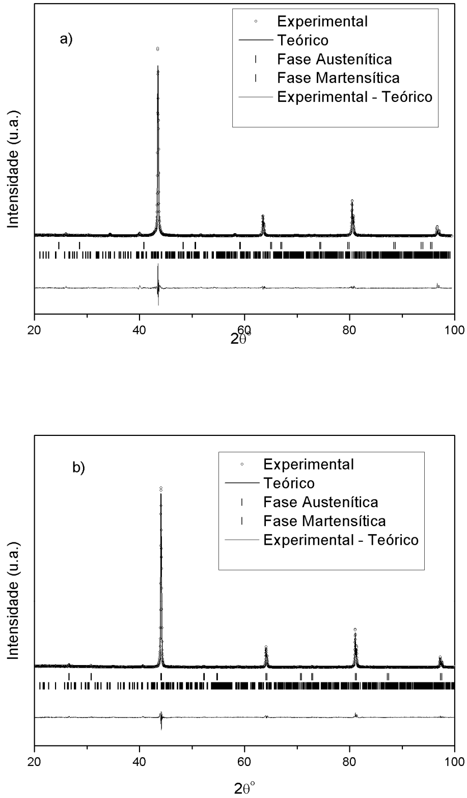
Figura 21: Análises dos difratogramas para amostras com: a) 9 h, e b) 12 h de moagem tratadas termicamente a 1123 K durante 4 h.
