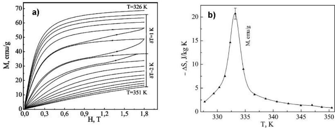
Figura 7: Retirada da ref. [08], ilustra a) magnetização em função do campo aplicado (isotermas), b) variação da entropia magnética para a liga \text{Ni}_{2,18}\text{Mn}_{0,82}\text{Ga} .
