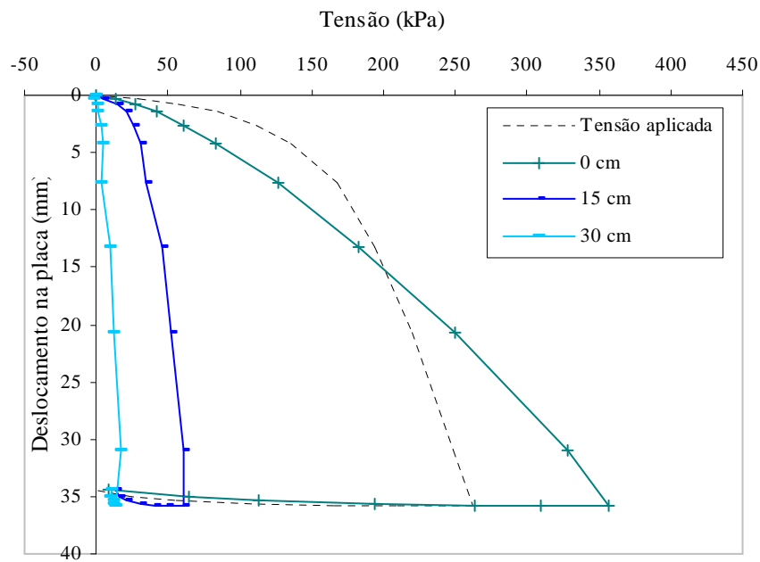
Figura 4.46: curva tensão versus deslocamento no alinhamento horizontal
