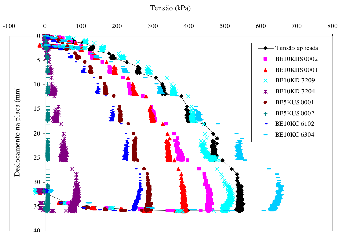
Figura 4.59: curvas tensão versus deslocamento do solo com 0,5 % de fibras
