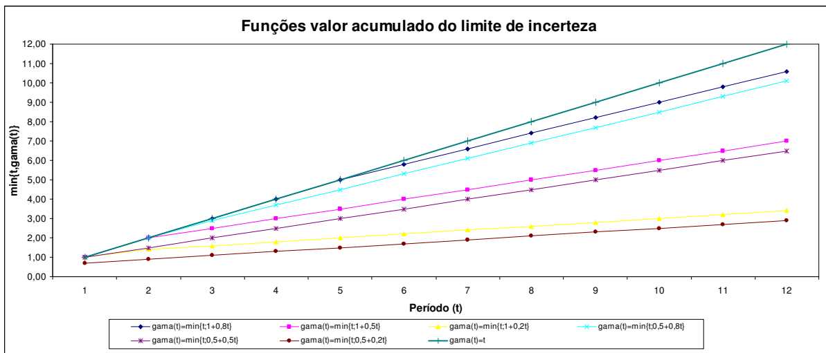
Figura 7.2: Funções lineares para computar a incerteza global para cada cenário
