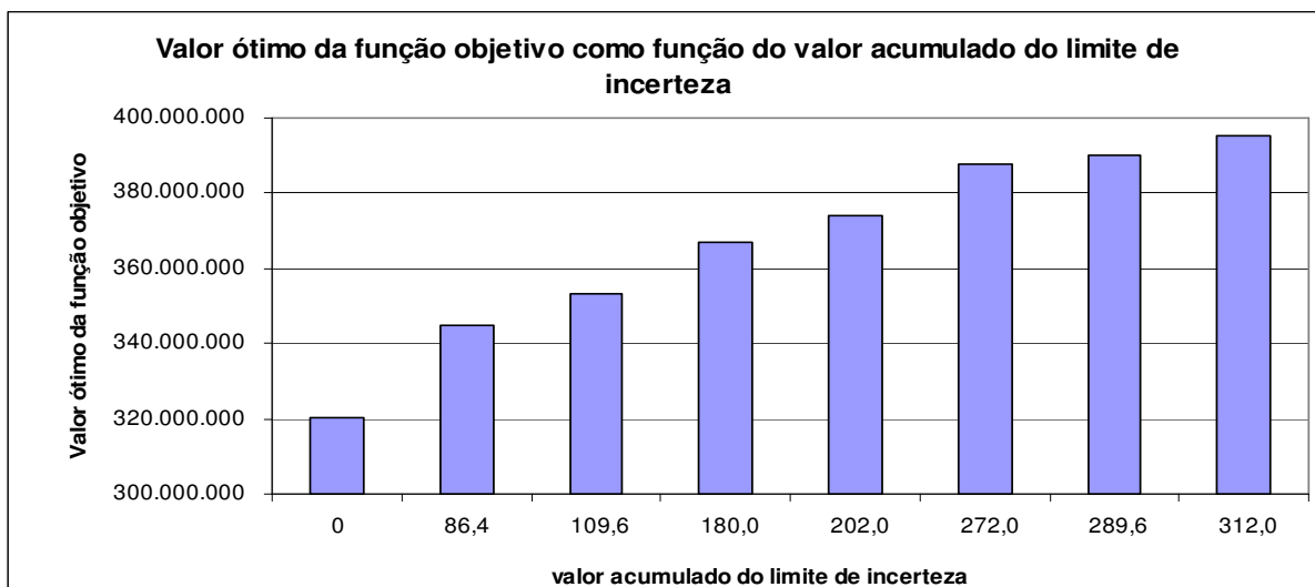
Figura 7.3: Valor ótimo da função objetivo como função do valor acumulado do limite de incerteza
