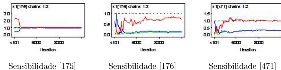
Figura 4.3.4.: Gráficos de Gelman & Rubin
