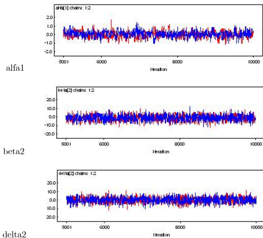
Figura 5.2.2.: Comportamento das trajetórias - 100% Variável Latente
