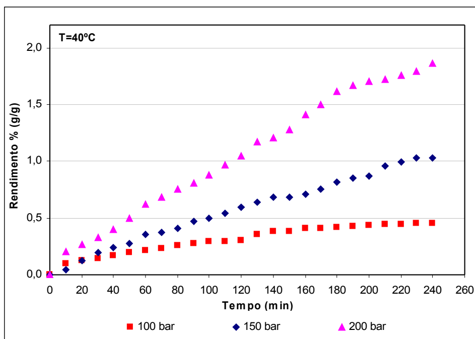
Figura 31. Curva de extração do óleo do pinhão-mansão, a 40°C nas pressões de 100, 150 e 200 bar
