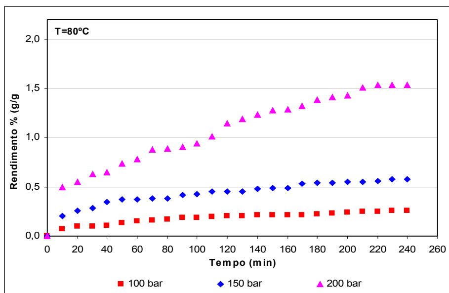
Figura 33. Curva de extração do óleo do pinhão-manso, a 80°C nas pressões de 100, 150 e 200 bar
