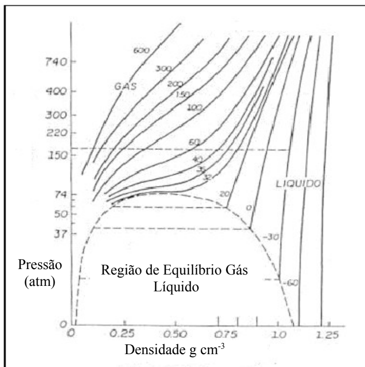
Figura 10. Dependência da densidade de CO 2 com a pressão e a temperatura (Fonte: SILVA, 2006)
