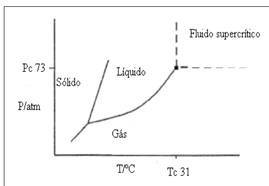
Figura 8. Diagrama pressão x temperatura e os equilíbrios entre os estados sólido, líquido e gasoso. Definição de região supercrítica para o \text{CO}_2 ; T_c : temperatura crítica; P_c : pressão crítica (Fonte: Carrilho, 2001; SILVA, 2006)
