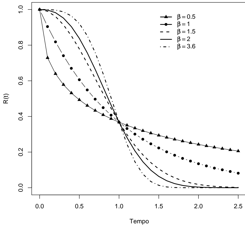
FIGURA 1.2: Função de confiabilidade do modelo Weibull ( \eta = 1 ).
