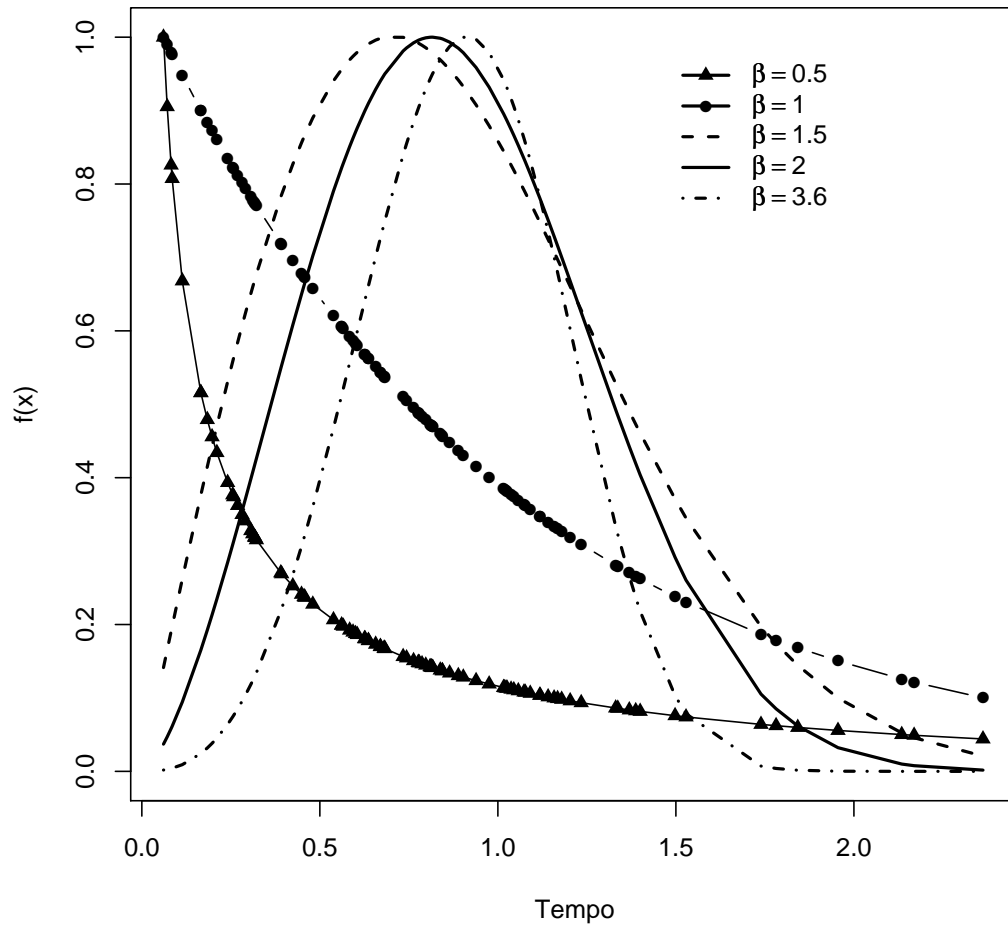
FIGURA 1.1: Função densidade do modelo Weibull ( \eta = 1 ).
