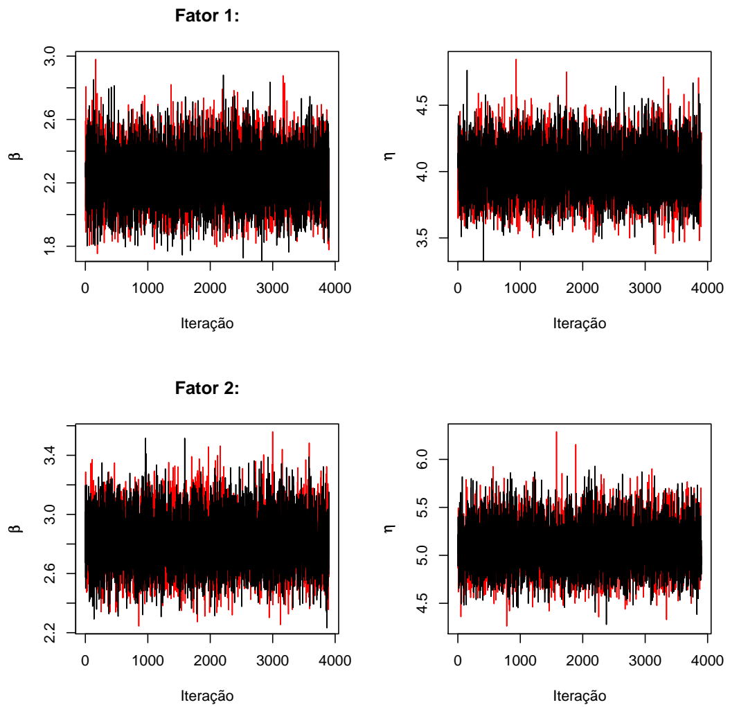
FIGURA 4.22: Traço das cadeias dos parâmetros dos fatores de risco 1 e 2.
