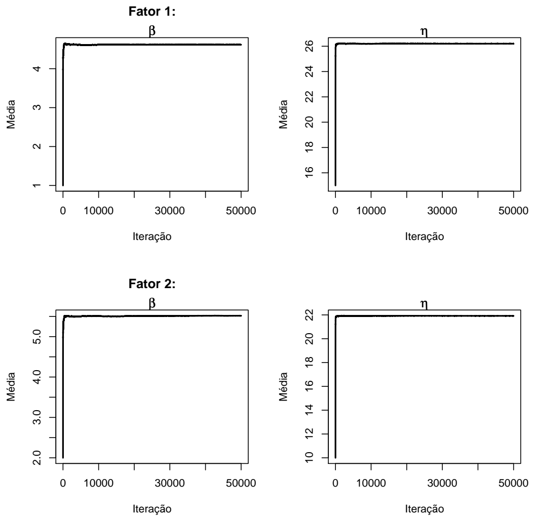
FIGURA 4.8: Médias ergódicas para os parâmetros dos fatores de risco 1 e 2 ( n = 10 ).
