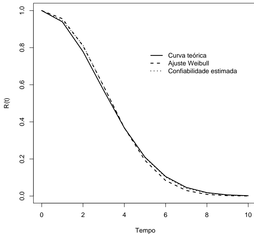
FIGURA 4.25: Ajuste da curva de confiabilidade do fator de risco 1.
