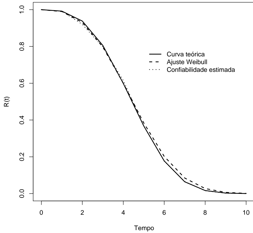
FIGURA 4.26: Ajuste da curva de confiabilidade do fator de risco 1
