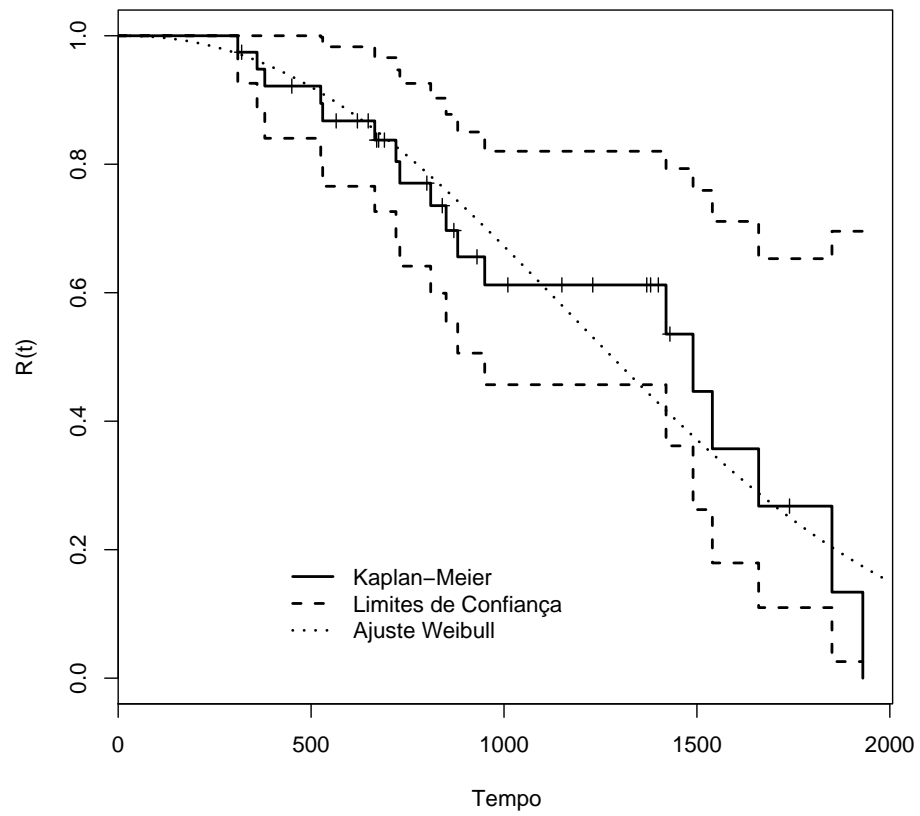
FIGURA 4.17: Ajuste da curva de confiabilidade do fator de risco B.
