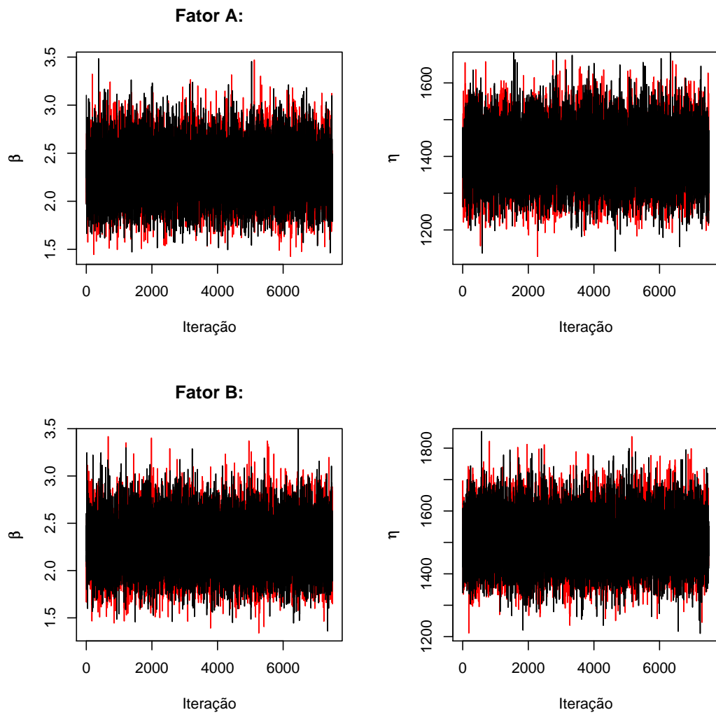
FIGURA 4.13: Traço das cadeias dos parâmetros dos fatores de risco A e B.
