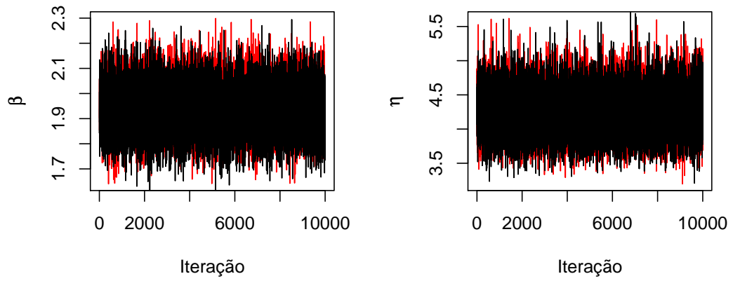
FIGURA 2.3: Traço das cadeias \beta e \eta .
