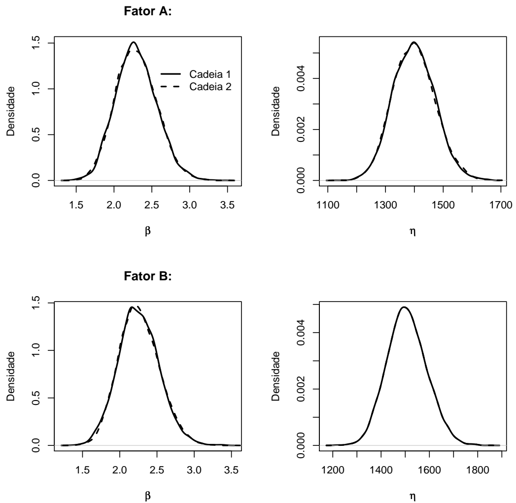
FIGURA 4.15: Funções densidade a posteriori estimadas dos parâmetros dos fatores de risco A e B.
