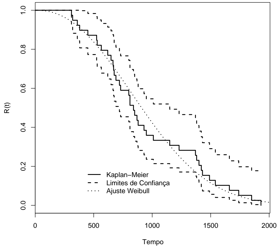
FIGURA 4.18: Ajuste da curva de confiabilidade do sistema.
