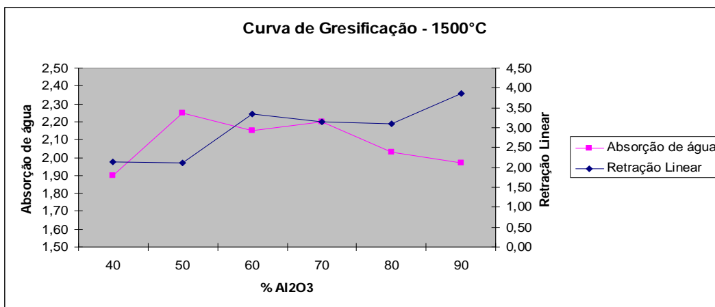
Gráfico 8 - Curva de gresificação a 1500°C.
