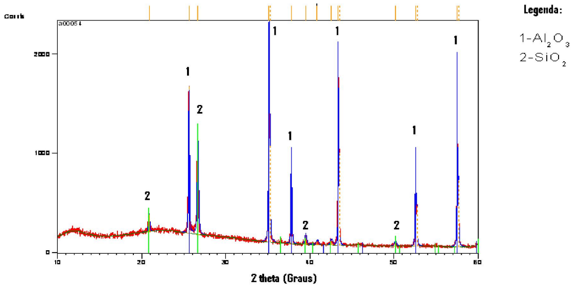
Figura 18- Difratograma de Raios X para o funil KN4.
