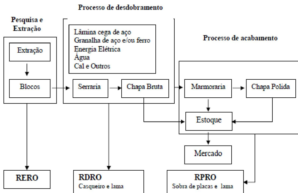
Figura 6 - Fluxograma do processo produtivo de Rochas Ornamentais. Fonte: BRAGA et al (2005).
