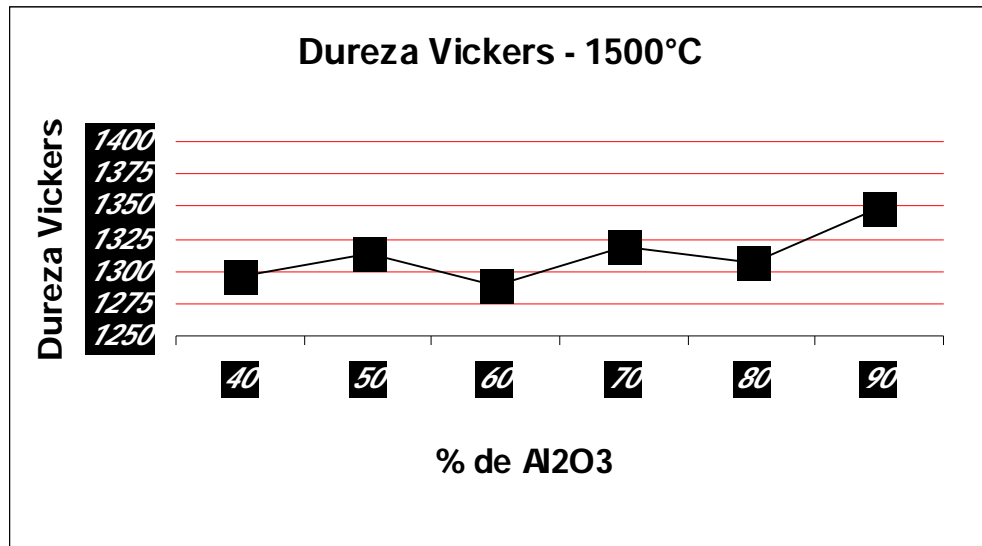
Gráfico 4 - Dureza Vickers para temperatura de sinterização a 1500°C.
