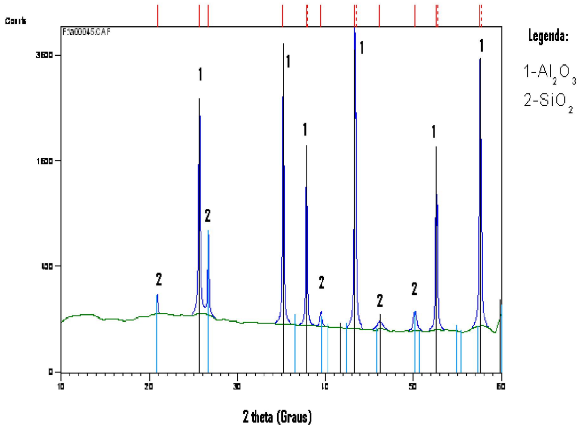
Figura 17 - Difratograma de raios X para a o funil KS K4-A.
