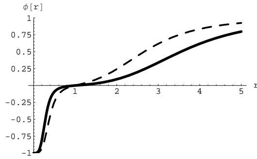
Figura 4.6: Perfil das soluções radiais para d = 2 dimensões no modelo \lambda = 4\mu , para d = 0,06249 (linha sólida contínua), e para d = 0,0624 (linha tracejada).
