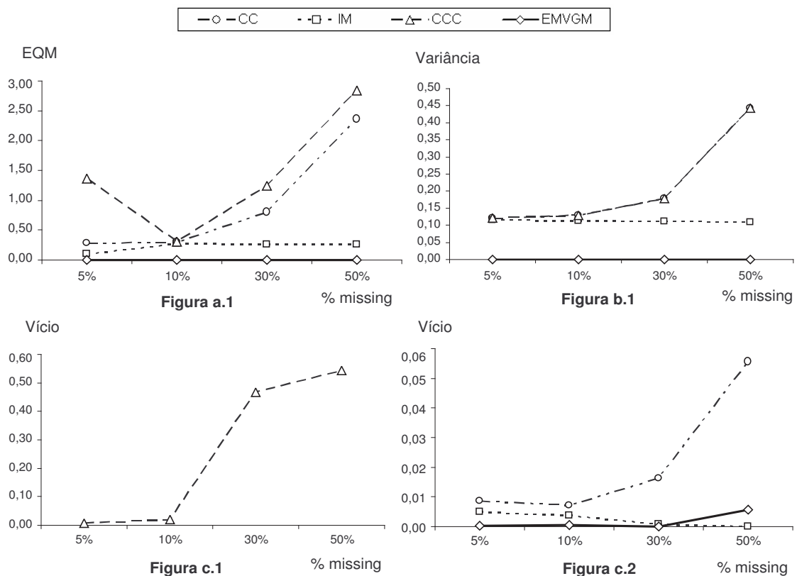
FIGURA 5.5: Erro Quadrático Médio (Figura a.1), Variância (Figura b.1) e Vício (Figura c.1 e c.2) para \hat{\beta}_1 para amostra de tamanho 500.
