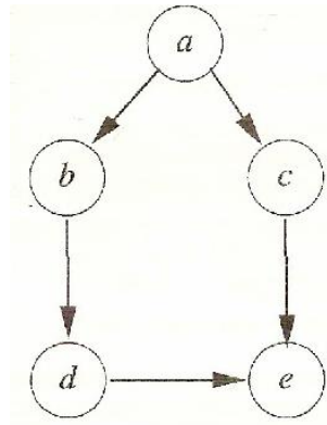
FIGURA A.1: Grafo Acíclico Orientado.
