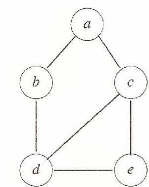
FIGURA A.2: Grafo moral correspondente a A.1.
