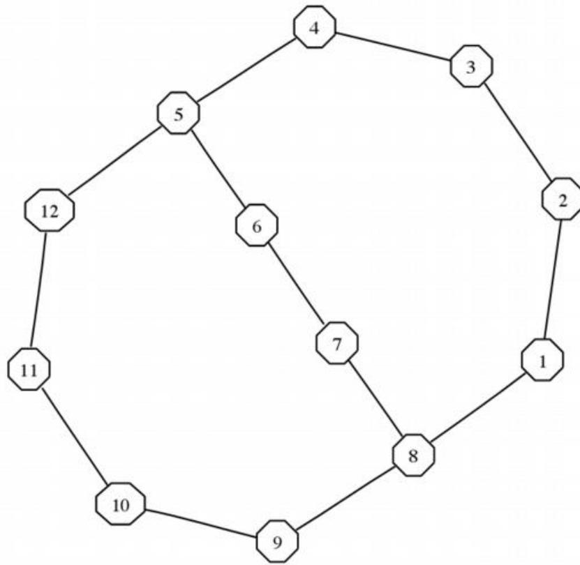
FIGURA 5.5: Grafo não-decomponível com 12 nós - segundo exemplo simulado.
