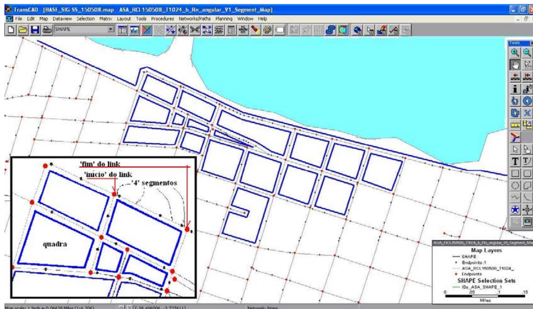
Figura 23. Base RCL's de Fortaleza, com links/arcos e nós da modelagem UTMS e ASA Fonte: o autor, obtido no software TransCAD.
