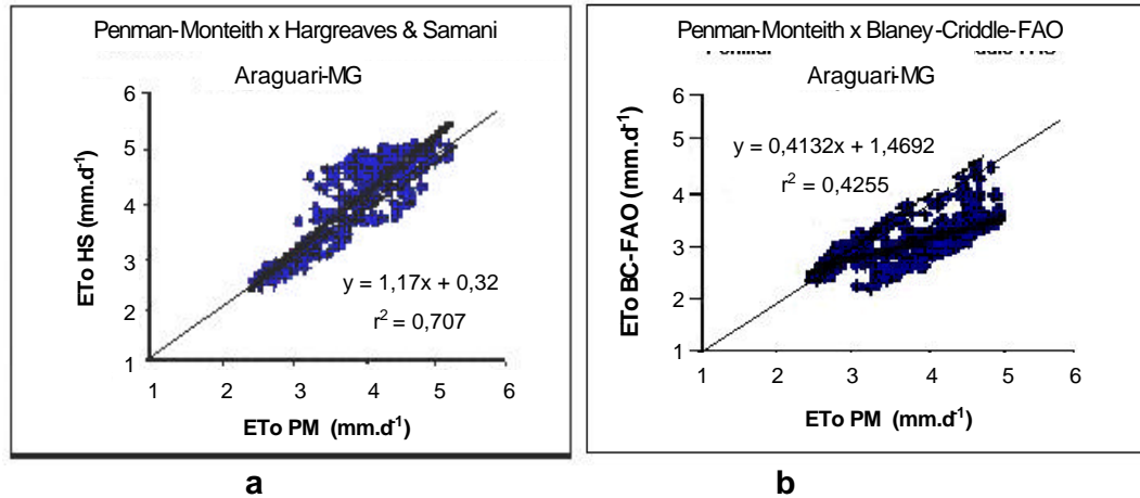
Figura 12 – Comparação entre os valores de ETo média diária estimados pelo método de Penman-Monteith (PM) e a ETo calculada pelos métodos simplificados Hargreaves & Samani (HS) e Blaney-Cridde-FAO (BC-FAO), respectivamente, para a cidade de Araguari, MG, Grupo A.
