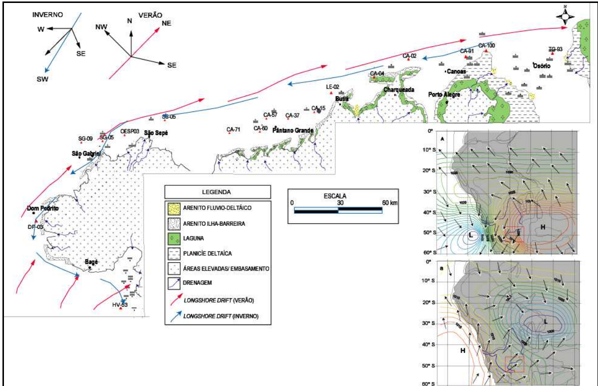
Figura 62 - Mapa paleofisiográfico e dinâmica costeira da porção sul-riograndense da Bacia do Paraná. Intervalo T3.
