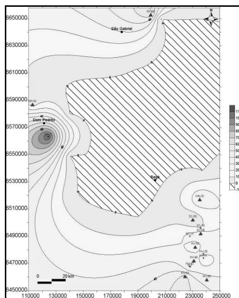
Figura 30 -Mapa de isópaca mostrando a espessura do TSMB2 na área 2. Maiores espessura a NW da área.
