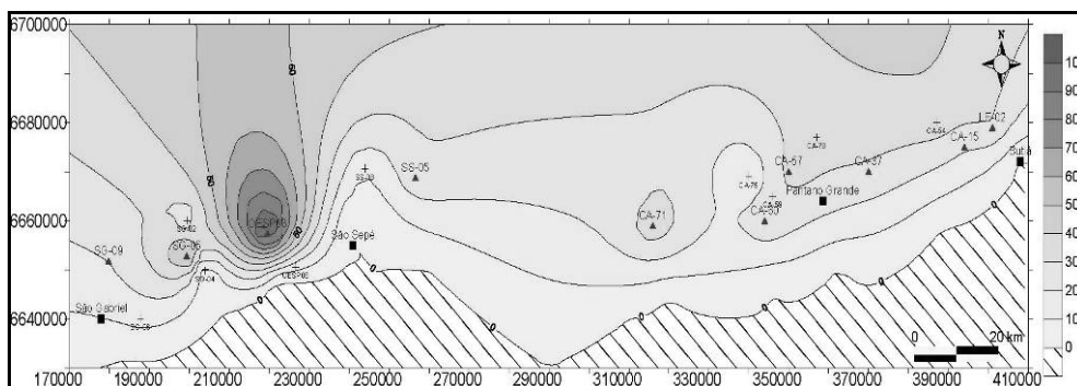
Figura 30 -Mapa de isópaca mostrando a espessura do TSMB2 na área 2. Maiores espessura a NW da área.
