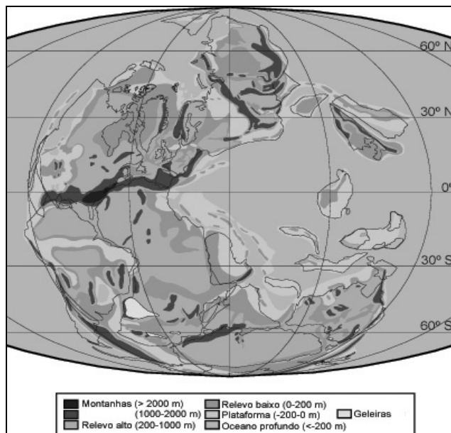
Figura 53- Reconstituição paleogeográfica para o Sakmario (Ziegler et al. , 1997).
