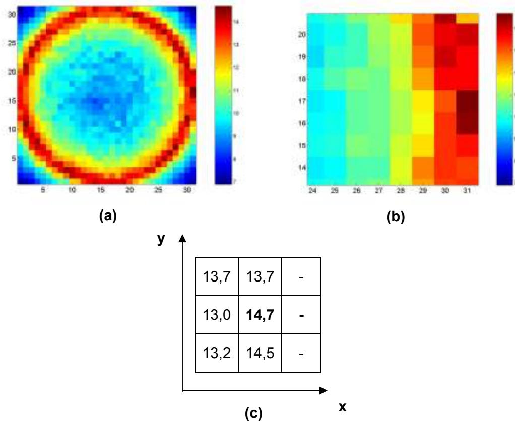
Figura 4.24: (a) Imagem bidimensional da interação de uma fonte volumétrica em anel isotrópica de 140 \text{ keV} posicionada a 0,0001 \text{ cm} de uma matriz detectora de BGO com 31 \times 31 elementos. (b) Detalhe ampliado da região da vizinhança de 8 do pico. (c) Os valores de energia depositadas F(x,y) em \text{MeV/g} em cada elemento da vizinhança do pico revelam a razão de contraste da imagem.
