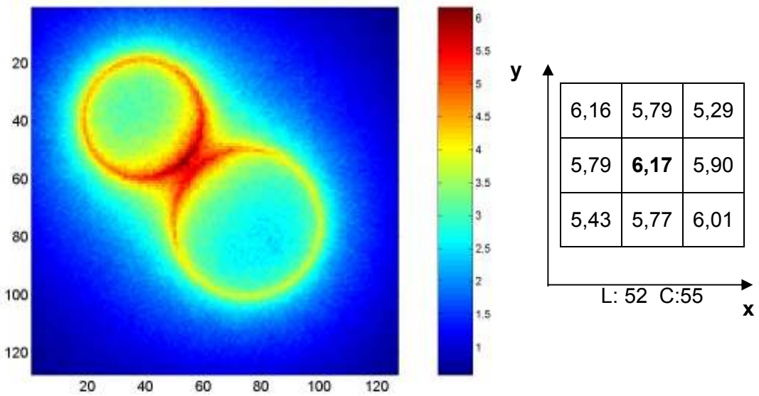
(a) \text{CdWO}_4 F(x,y) \text{ máx} = 6,169 \pm 0,130 \text{ MeV/g}
