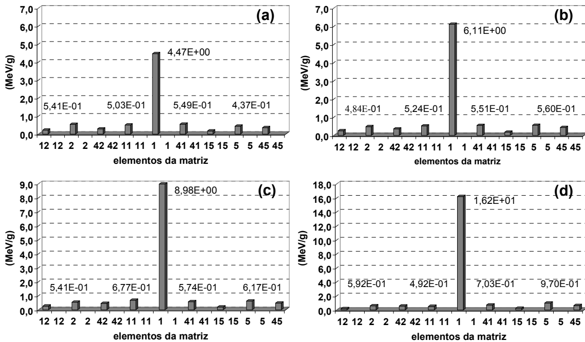
Figura 4.17: Distribuição da deposição em energia na matriz 3x3 correspondente ao elemento 1 e aos elementos da sua vizinhança de oito, com material refletor/separador de MgO com espessuras: 0,2 mm (a), 0,4 mm (b), 0,6 mm (c) e 0,8 mm (d), para a energia de 159 keV. Distância fonte-detector de 0,0016 cm. Num. Hist. = 1E+03.
