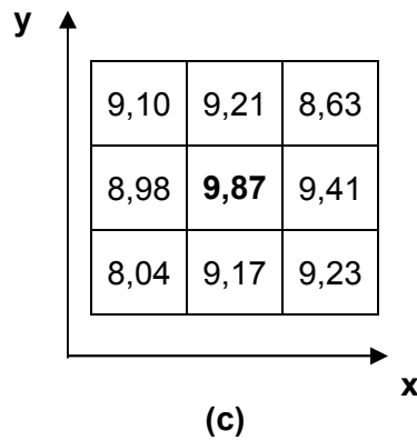
Figura 4.26: (a) Imagem bidimensional da interação de duas fontes volumétricas e isotrópicas em anel de 159 keV, com diâmetros de 420 \mu\text{m} posicionadas a 0,0001 cm de uma matriz detectora de 127 x 127 elementos de BGO. (b) Detalhe ampliado da região de aproximação dos dois folículos vizinhança de 8 do pico. (c) Os valores de energia depositadas F(x,y) em MeV/g em cada elemento da vizinhança do pico revelam a razão de contraste da imagem.
