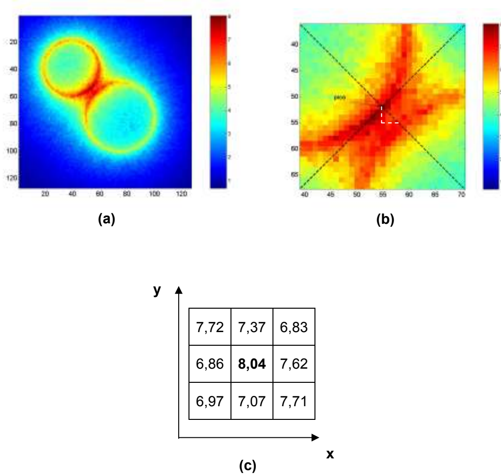
Figura 4.25: (a) Imagem bidimensional da interação de duas fontes volumétricas e isotrópicas em anel de 159 keV, com diâmetros de 420 \mu\text{m} e 520 \mu\text{m} posicionadas a 0,0001 cm de uma matriz detectora de 127 x 127 elementos de BGO. (b) Detalhe ampliado da região de aproximação dos dois folículos. (c) Os valores de energia depositadas F(x,y) em MeV/g em cada elemento da vizinhança do pico revelam a razão de contraste da imagem.
