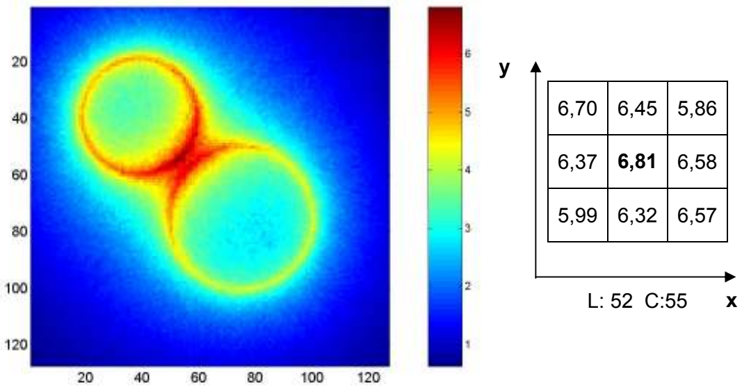
(b) LSO F(x,y) \text{ máx} = 6,807 \pm 0,141 \text{ MeV/g}
