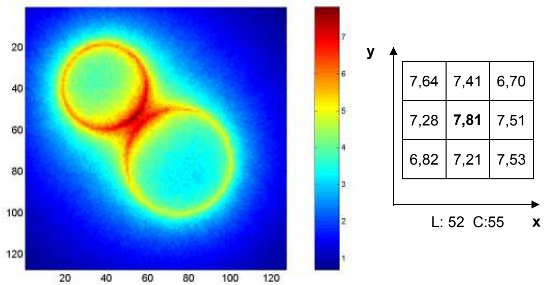
(b) BGO F(x,y) \text{ máx} = 7,814 \pm 0,103 \text{ MeV/g}
