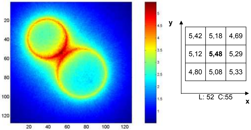
(a) GSO F(x,y) \text{ máx} = 5,478 \pm 0,113 \text{ MeV/g}
