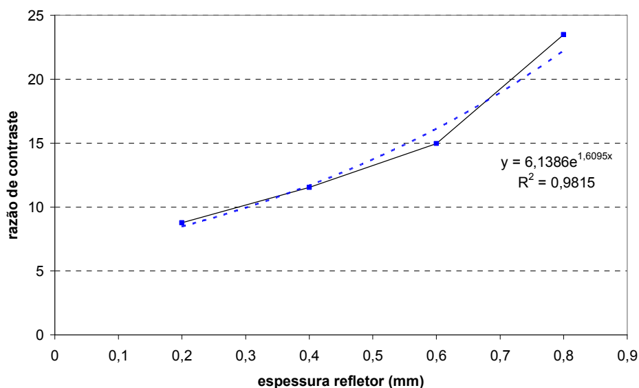
Figura 4.18: Relação entre a razão de contraste e a espessura do refletor.
