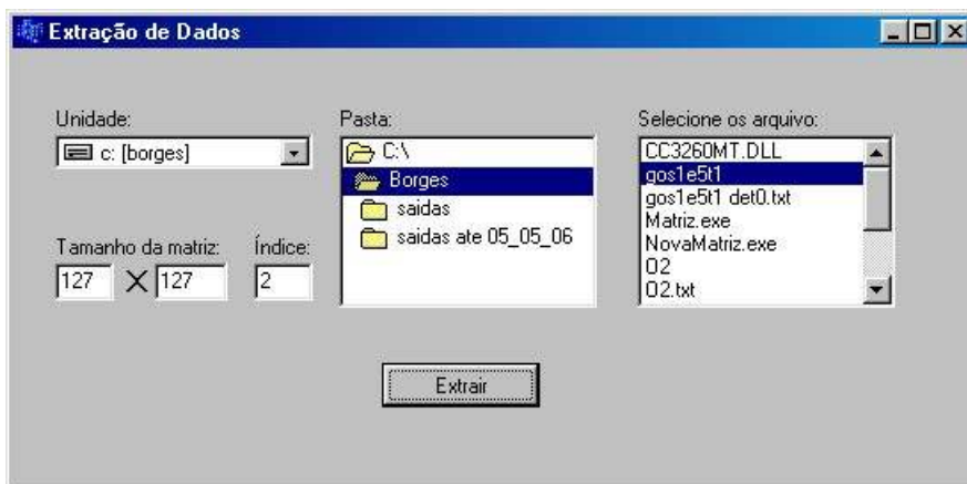
Figura 3.6: Interface gráfica do programa de extração de dados utilizado para selecionar as informações úteis geradas pelo código escrito no MCNP4B.
