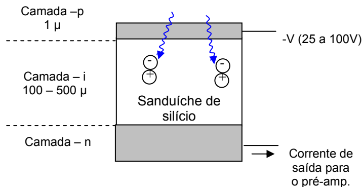
Figura 2.12: Configuração básica de um fotodiodo PIN.
