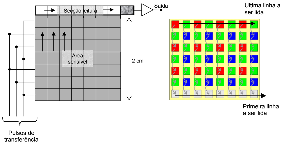
Figura 2.14: Representação esquemática da superfície de um CCD. Ao lado pode ser visto o deslocamento das cargas entre cada linha da matriz.
