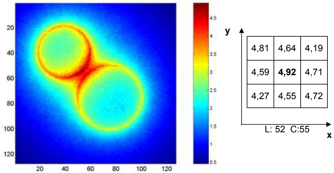
(a) CsI(Tl) F(x,y) \text{ máx} = 4,916 \pm 0,103 \text{ MeV/g}
