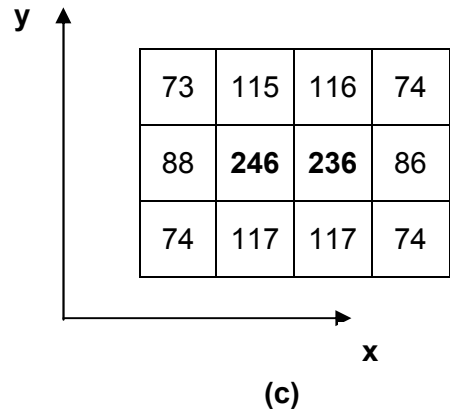
Figura 4.22: (a) Imagem bidimensional da interação de uma fonte pontual isotrópica de 159 keV posicionada a 0,0001 cm do elemento refletor 1 (pos=-0,00051) de uma matriz detectora 31 x 31 de BGO. (b) Detalhe ampliado da região da vizinhança de 8 dos elementos 1 e 51 da matriz. (c) Os valores de energia depositadas F(x,y) em MeV/g em cada elemento da vizinhança dos elementos 1 e 11 revelam a alteração na razão de contraste da imagem.
