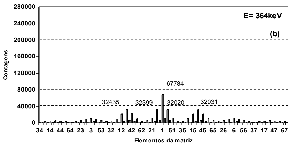
Figura 4.5: Distribuição da interação dos fótons na matriz detectora de CsI(Tl) com elementos de 1 \times 1 \times 1 \text{ cm}^3 e separador de MgO com espessura 2 mm, para fonte radioativa de 159 keV (a) e 364 keV (b), distante 0,5 cm da matriz detectora e na posição 1. Num. Hist. = 1\text{E}+06 .
