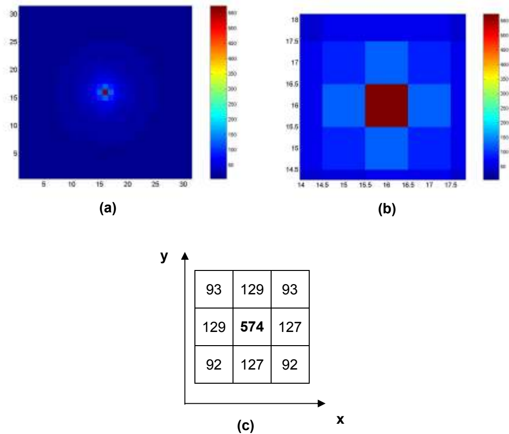
Figura 4.19: (a) Imagem bidimensional da interação de uma fonte pontual isotrópica de 159 keV posicionada a 0,0001 cm do elemento detector 1 de uma matriz detectora 31 x 31 de BGO. (b) Detalhe ampliado da região da vizinhança de 8 do elemento 1. (c) Os valores de energia depositada F(x,y) em MeV/g em cada elemento da vizinhança do elemento 1 revelam a razão de contraste da imagem.
