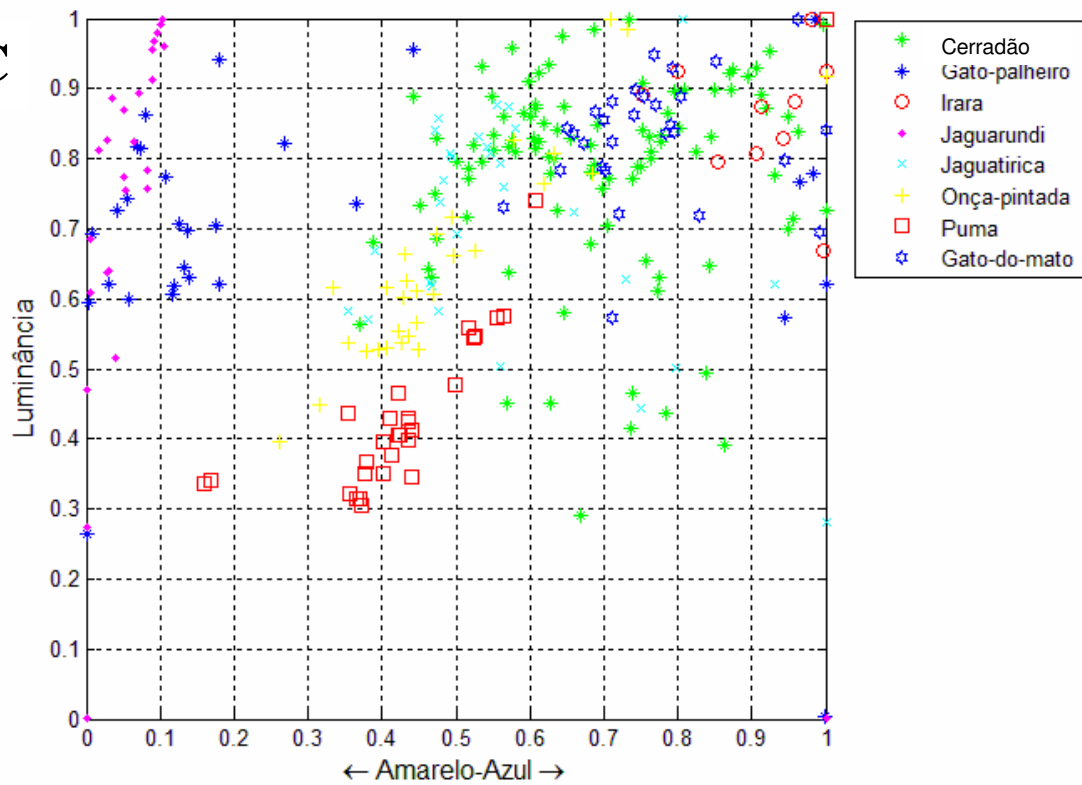
Figura 12. Diagrama de cromaticidade contrastando os potenciais predadores de C. penicillata contra o plano de fundo do cerradão para os três fenótipos dicromatas: A) 425-561, B) 425-556 e C) 425-543.
