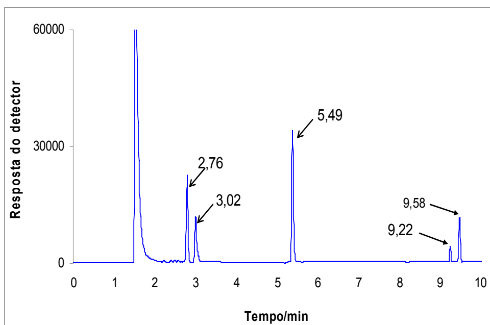
Figura 4. Cromatograma de uma solução padrão contendo os agrotóxicos clorpirifós ( 100,0 \mu\text{g L}^{-1} ), thiamethoxam ( 500,0 \mu\text{g L}^{-1} ) e deltametrina ( 100,0 \mu\text{g L}^{-1} ), e os tempos de retenção: t_R = 2,76 min. para clorpirifós; t_R = 3,02 min. para thiamethoxam; t_R = 5,49 min. para bifentrina (padrão interno) e t_R = 9,22 e 9,58 min para deltametrina.
