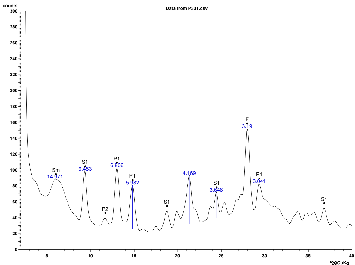
Figura 3.12 – Amostra U107 (perfil D7 da ponta Uchatka, 20-40 cm): Fração total.
