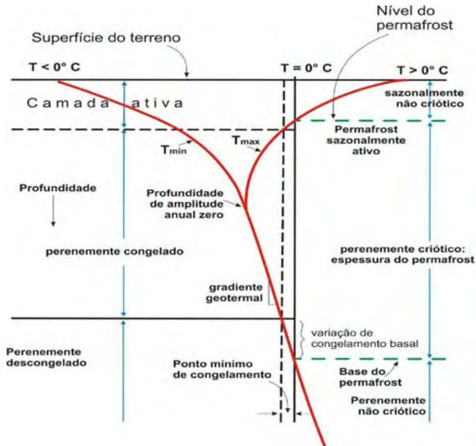
Figura 3.6 – Perfil esquemático do comportamento térmico do permafrost (adaptado de Dobinski, 2006).
