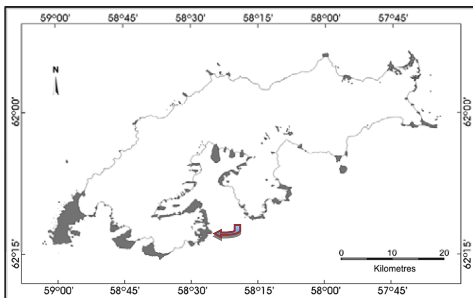
Figura 2.3. Mapa da ilha Rei George apresentando as áreas livres de gelo (em cinza escuro), basicamente restritas a pontas e pequenas penínsulas, em sua maioria no seu setor meridional. A seta indica a área livre de gelo da borda leste da península Warszawa. (modificado de Simões et al. , 2004).
