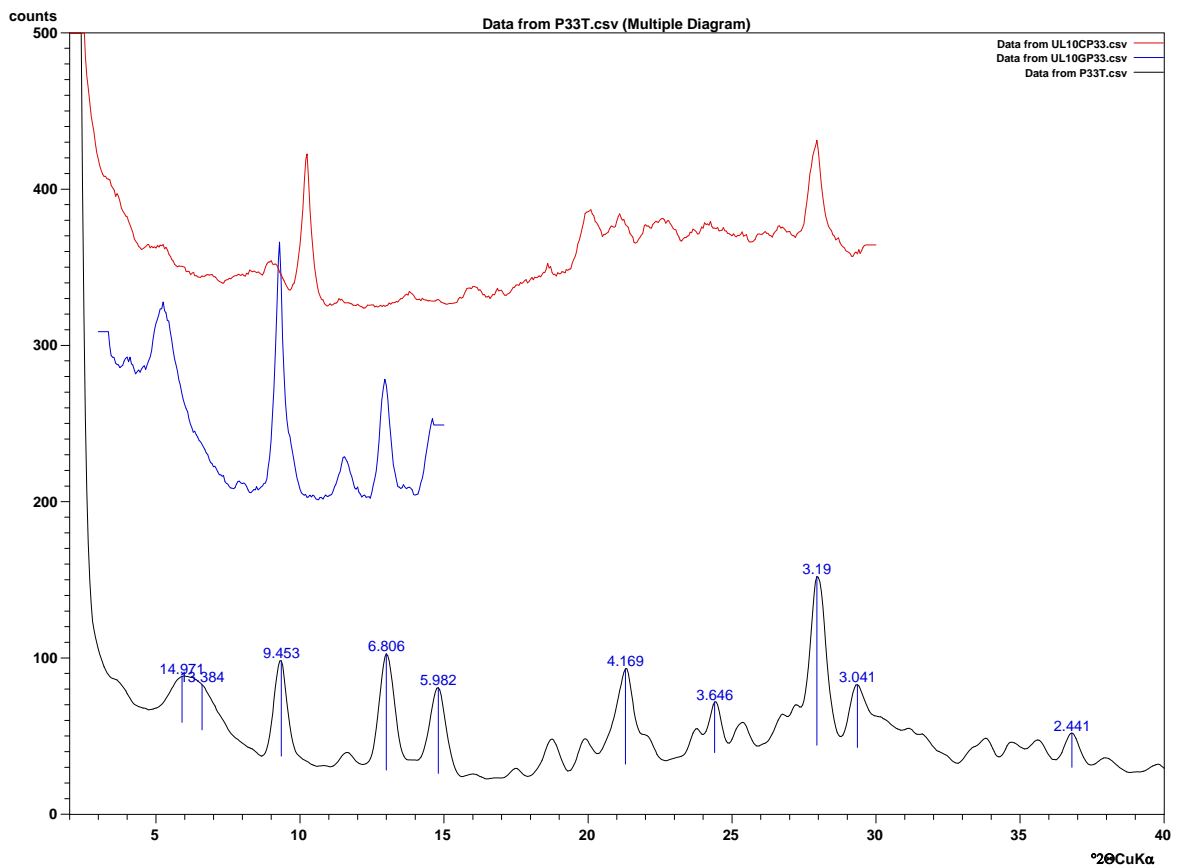
Figura 3.13 – Amostra U107. Fração total (traço preto), fração menor que 10 \mu\text{m} , orientada e glicolada (traço azul), fração menor que 10 \mu\text{m} , orientada e calcinada (traço vermelho).
