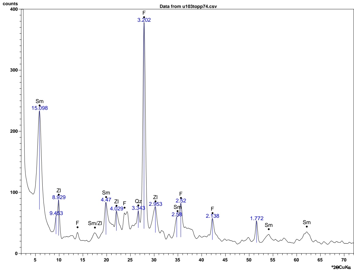
Figura 3.9 – Amostra U103, fração total.
