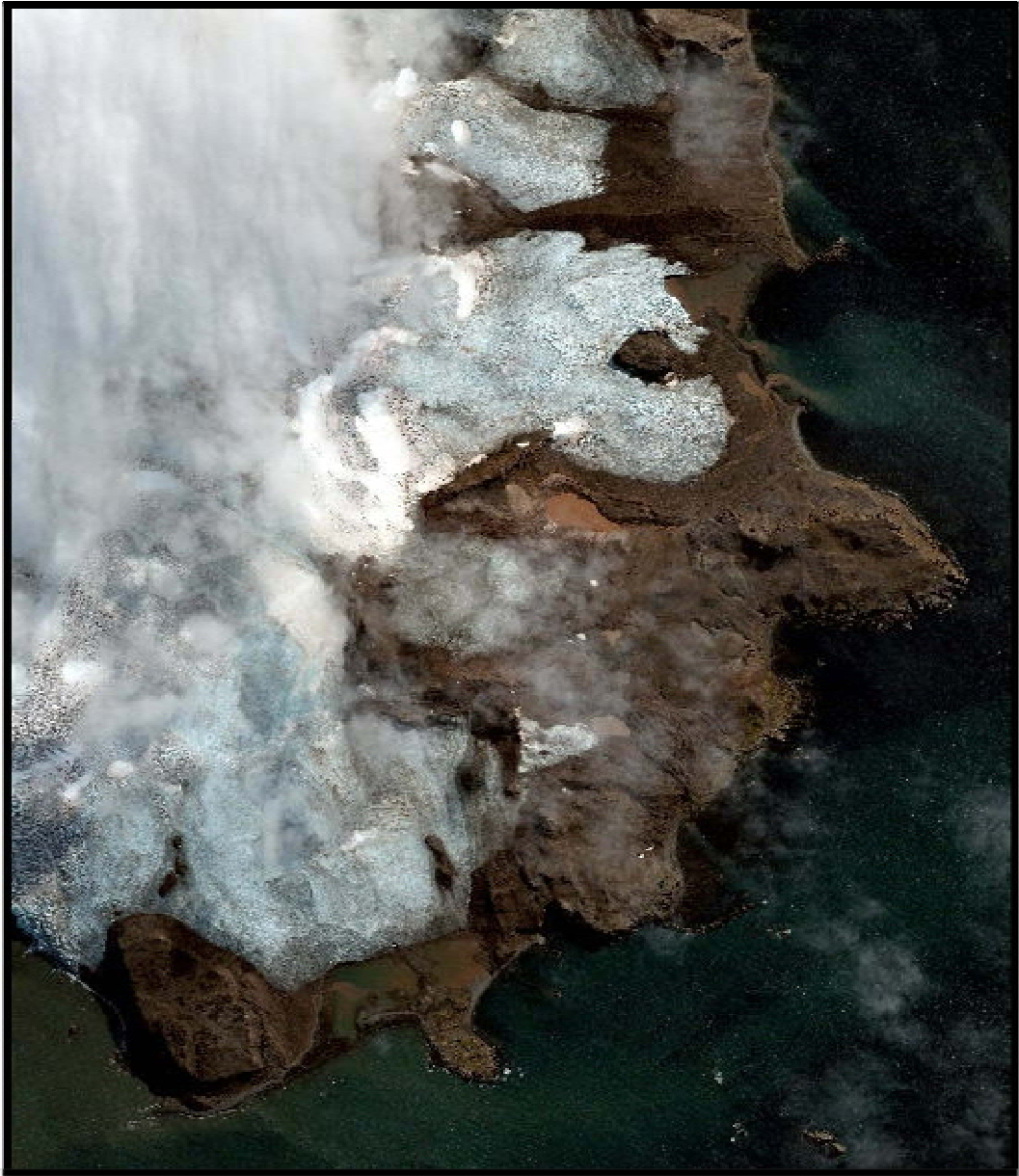
Figura 2.8 – Imagem orbital Quickbird , da qual os 2/3 meridionais foram utilizados para o mapeamento geomorfológico.
