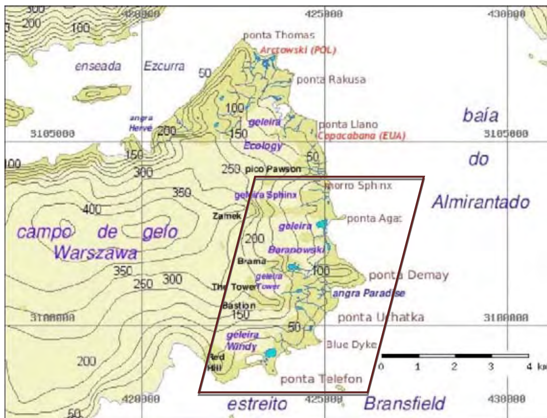
Figura 1.2 – Localização da área de estudo na borda leste da península Warszawa e margem oeste da baía do Almirantado, na ilha Rei George. A altimetria, os limites e as coordenadas geográficas foram obtidas do sistema de informações geográficas da ilha Rei George, KGIS (modificado de SCAR, 2007).
