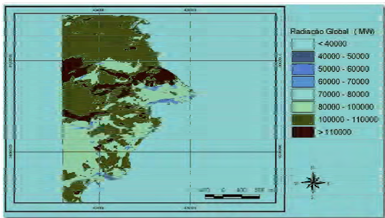
Figura 4.9 – Radiao global na rea de estudo no vero 2005-2006.
