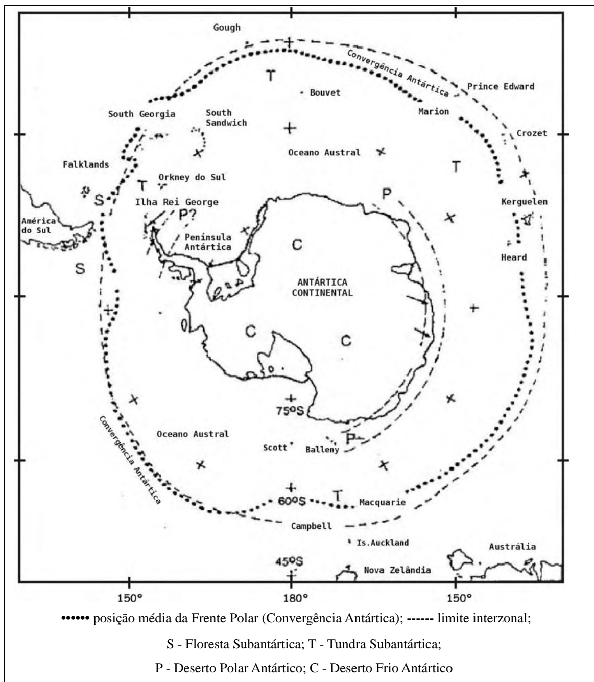
Figura 3.1. Zonas pedológicas na região circumpolar meridional (modificado de Bockheim & Ugolini, 1990).
