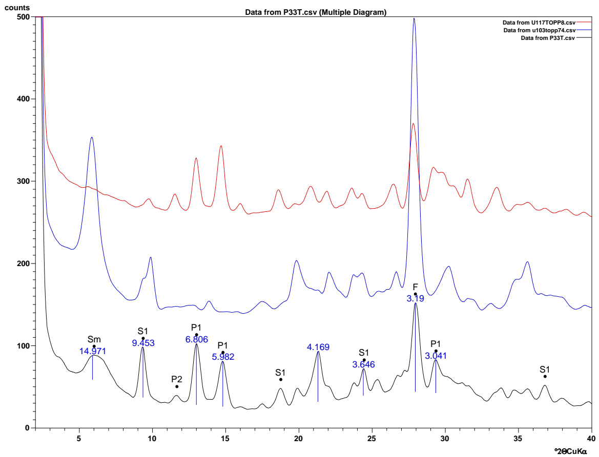
Figura 3.14–Amostra U107 (traço preto), amostra U103 (traço azul) e U117 (traço vermelho).
