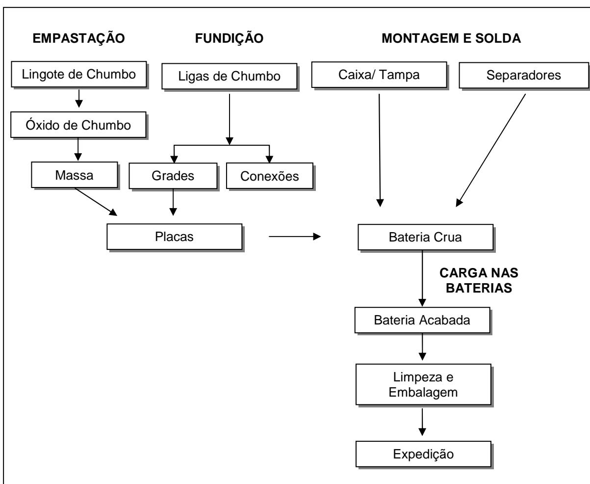
Figura 11 – Quadro com os principais processos de industrialização de baterias automotivas
