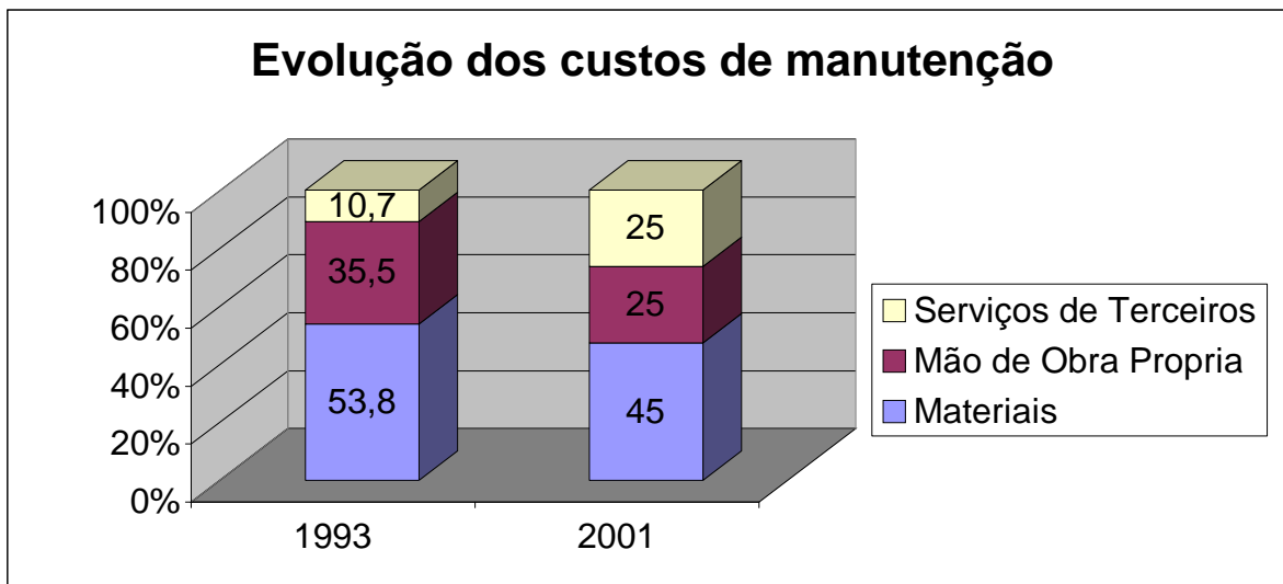
Gráfico 1 Evolução da composição dos custos de manutenção na indústria de cimento
