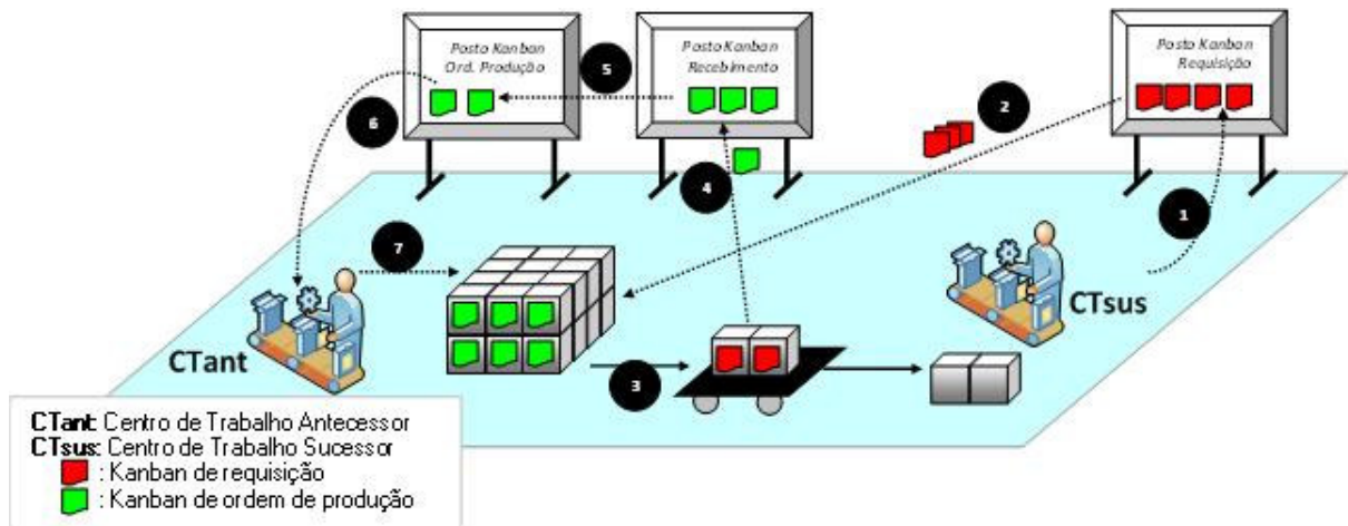
Figura 3.4. Sistema Kanban-CNE de CARTÃO DUPLO. Fonte: adaptado de Monden (1984).
