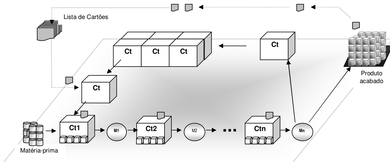
Figura 3.2. Sistema CONWIP CNE. Fonte: Fernandes (2003).
