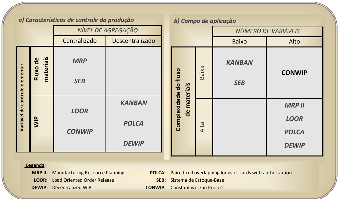
Figura 3.16. Classificação dos sistemas de controle da produção Fonte: Lööding et al , 2003.
