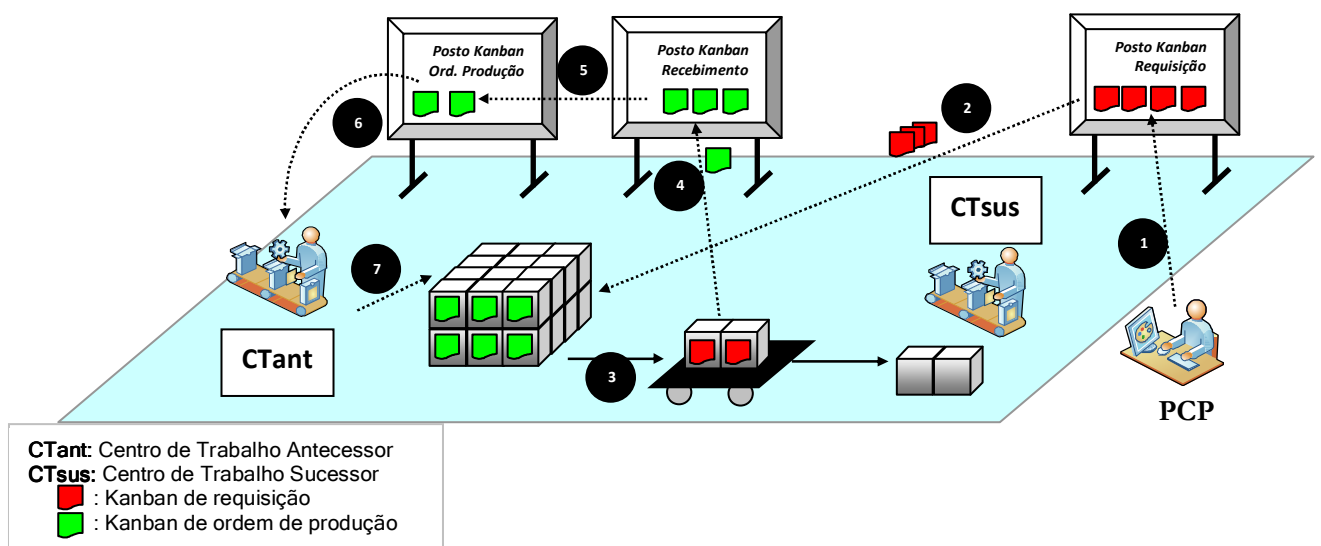
Figura 3.10. Kanban-H de Produção de duplo cartão. Fonte: elaborada pelo autor.
