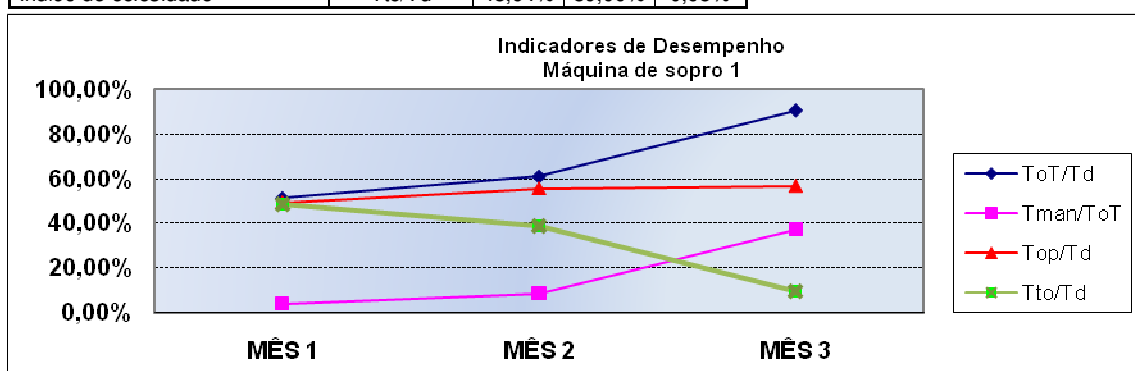
Figura 5.27. Gráficos de monitoramento das máquinas de sopro do Processo-Chave.
