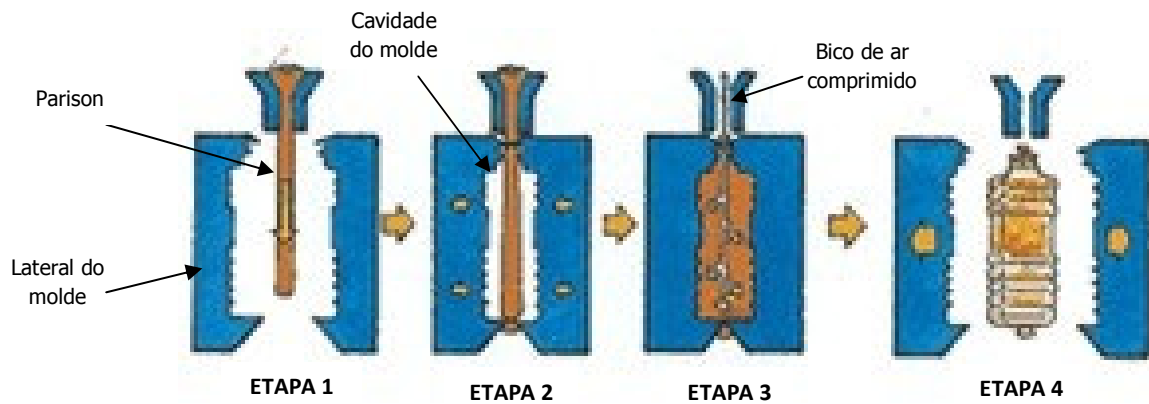
Figura 5.2. Fases do processo de moldagem por sopro.
