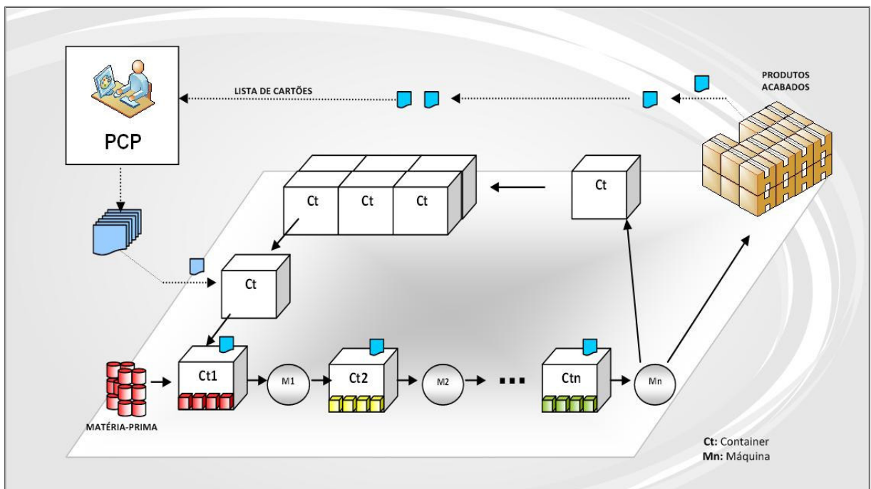
Figura 3.7. Sistema CONWIP H. Fonte: Fernandes (2003).
