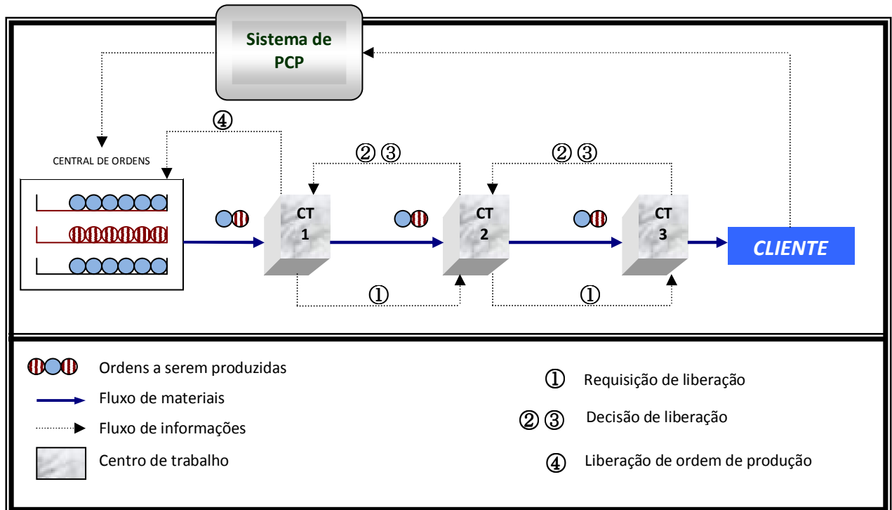
Figura 3.15. Diagrama esquemático de funcionamento do sistema DEWIP.
