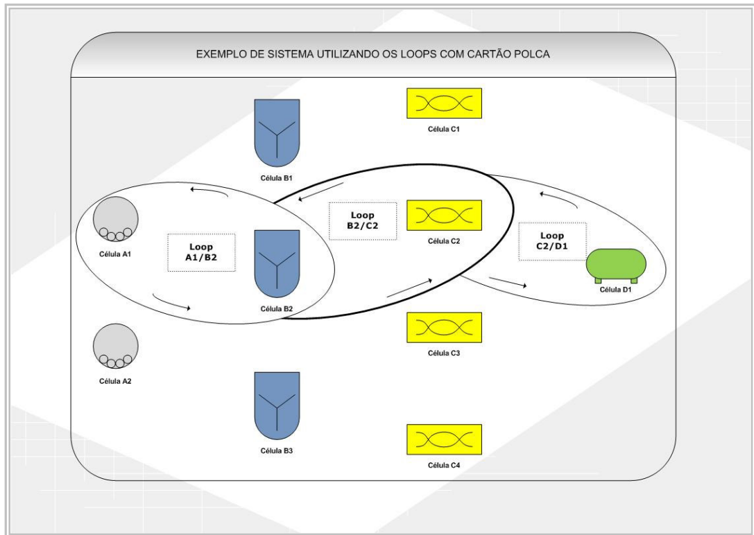
Figura 3.12. Esquema ilustrativo de um sistema POLCA. Fonte: Suri (1998a).
