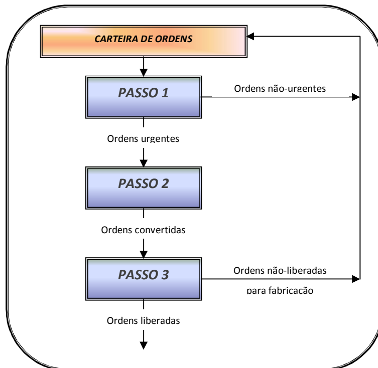
Figura 3.14. Passos de funcionamento do LOOR (WIENDAHL, 1995).
