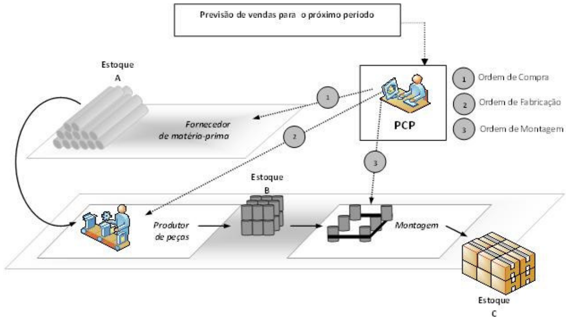
Figura 3.5. Esquema do Sistema de Estoque-base Fonte: elaborada pelo autor.
