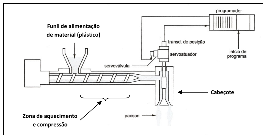
Figura 5.3. Diagrama esquemático do processo de moldagem por sopro.
