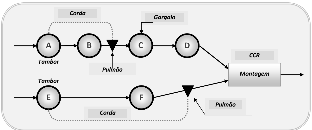
Figura 3.11. Esquema de um processo DBR.
