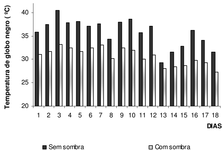
Figura 13 – Perfil da temperatura de globo negro média com e sem sombra
