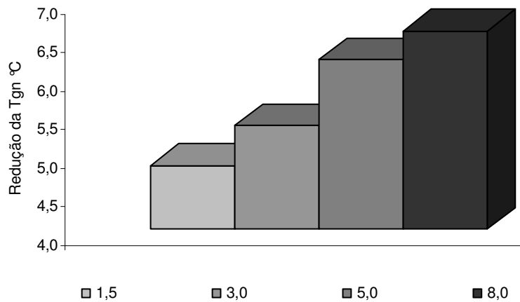
Figura 14 - Redução de temperatura de globo de acordo com o aumento da área de sombra
