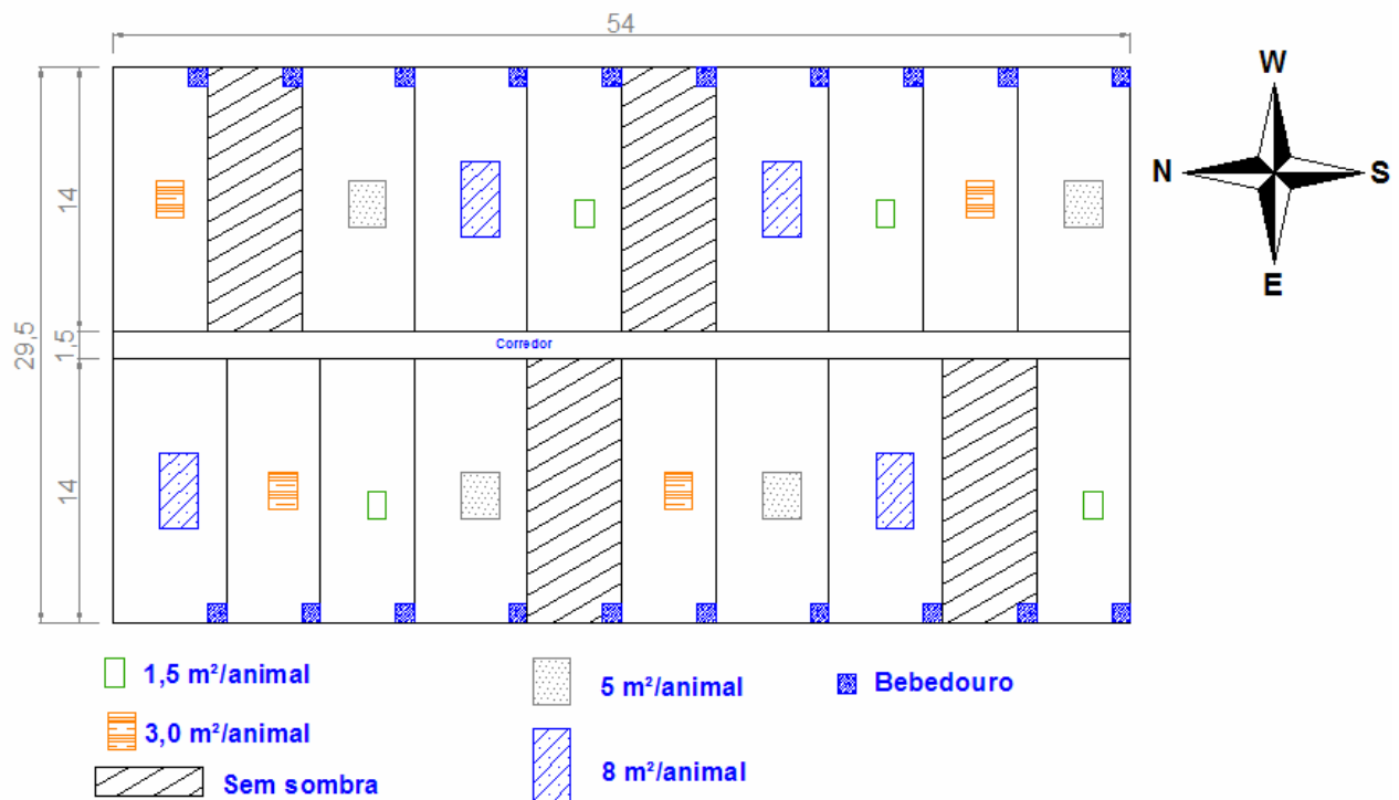
Figura 5 – Planta baixa do campo experimental
