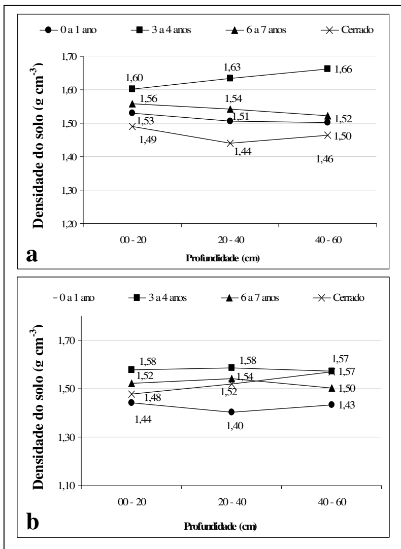
Figura 16: Distribuição da densidade do solo ao longo do perfil no inverno (a) e verão (b).
