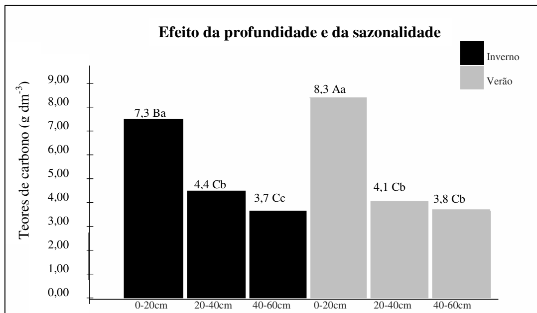
Figura 15: Teores de carbono orgânico no solo em função da interação entre profundidade e sazonalidade. (Letras iguais minúsculas dentro do tratamento e maiúsculas entre os tratamentos não diferem entre si a 5% de probabilidade).
