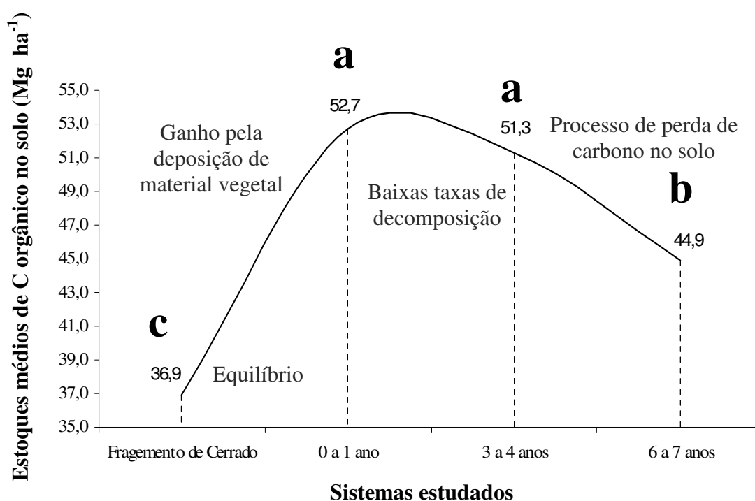
Figura 23: Curva de distribuição dos estoques totais de carbono de 0 a 60 cm de profundidade entre os plantios puros e o fragmento de Cerrado.
