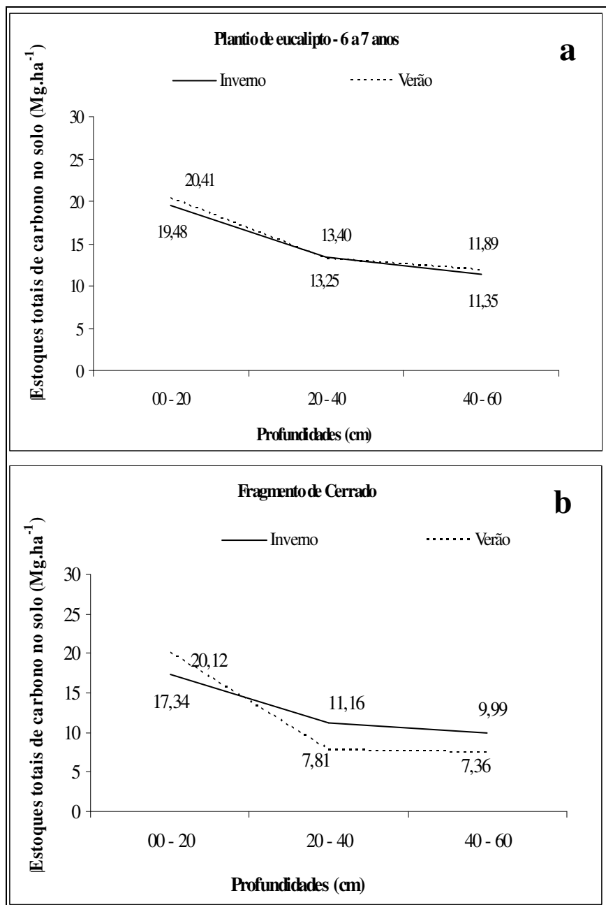
Figura 20: Estoques totais de carbono orgânico no solo ao longo do perfil para: a) plantio de eucalipto de 6 a 7 anos de idade; b) fragmento de Cerrado.
