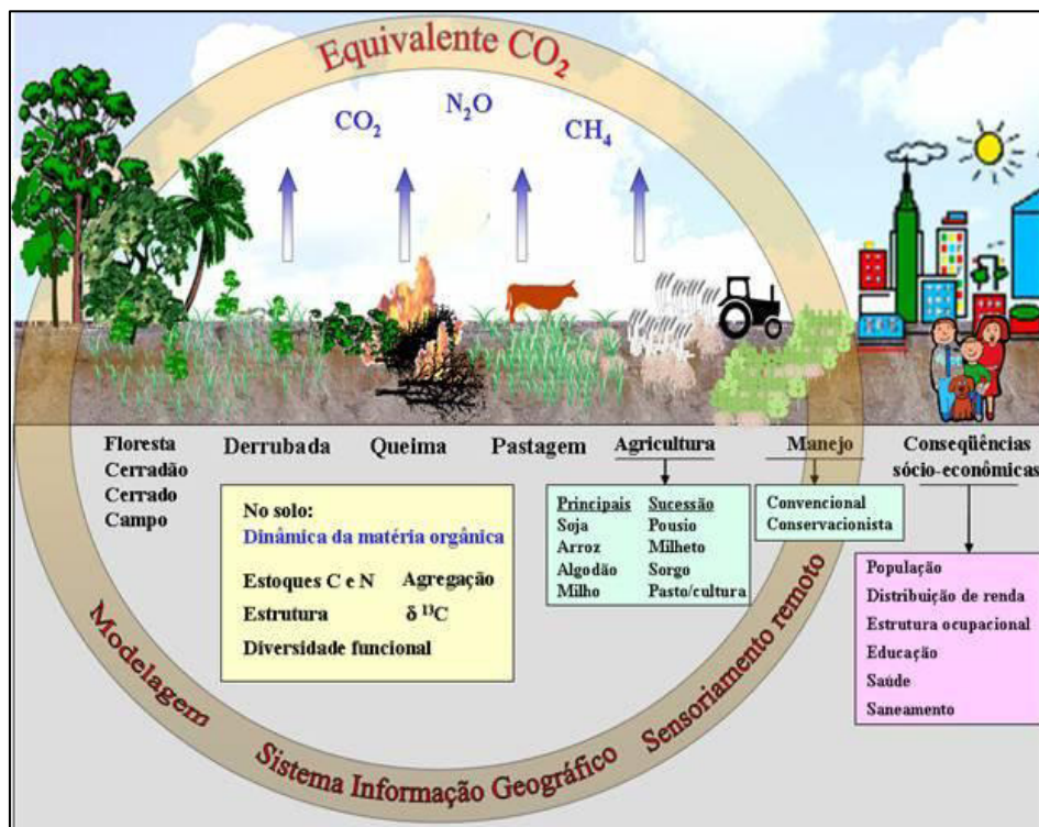
Figura 1: Estoques globais de carbono nos ecossistemas terrestres (CERRI & CERRI, 2007).
