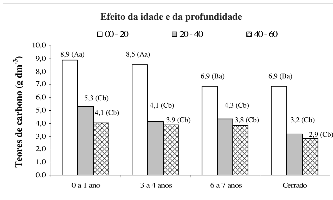
Figura 14: Teores de carbono no solo ao longo do perfil. (Letras iguais minúsculas dentro do tratamento e maiúsculas entre os tratamentos não diferem entre si a 5% de probabilidade).
