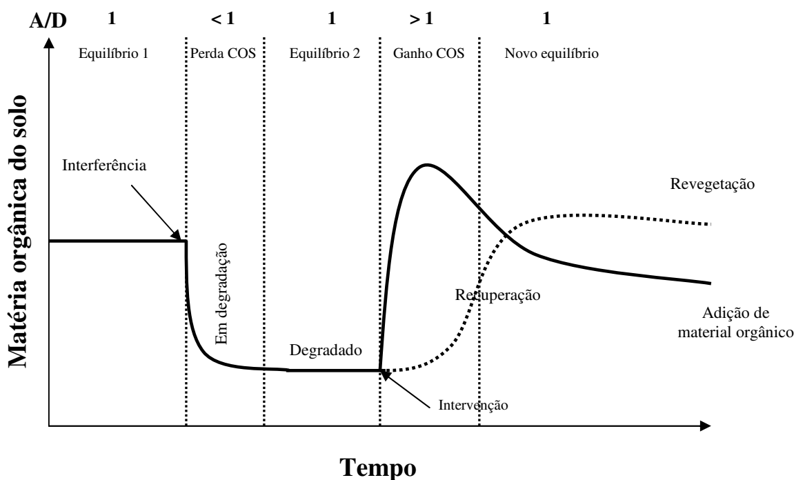
Figura 2: Modelo conceitual da decomposição/acúmulo de carbono orgânico do solo em áreas degradadas e após intervenção visando a recuperação da MOS pela adição de material orgânico ou pela revegetação. A/D = razão entre a adição e a decomposição de carbono (desenvolvido a partir de Batjes, 2001 e Siqueira et al., 2008).
