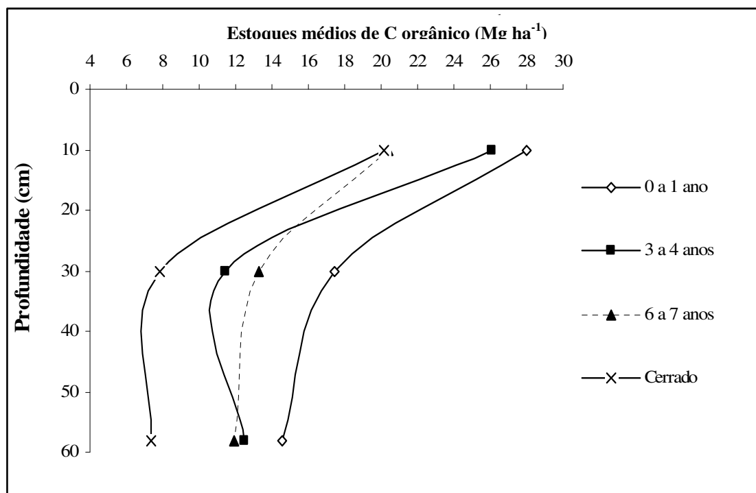
Figura 18: Acúmulo de C orgânico ( \text{Mg ha}^{-1} ) sob plantios de Eucalyptus grandis e de um fragmento de Cerrado no verão.
