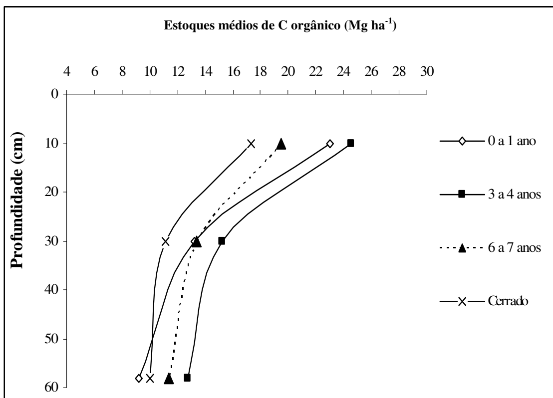
Figura 17: Acúmulo de C orgânico (Mg ha -1 ) sob plantios de Eucalyptus grandis e de um fragmento de Cerrado no inverno.
