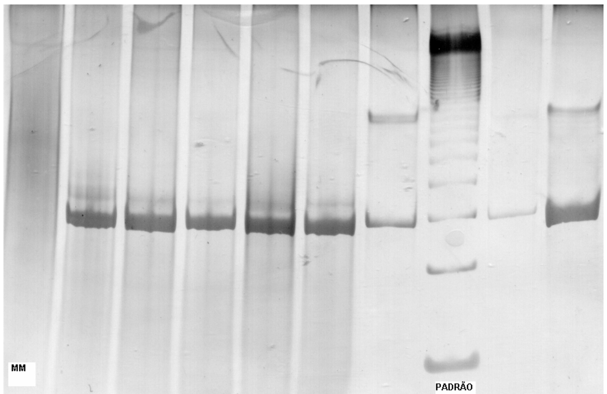
Figura 8: gel de poliacrilamida com produtos de PCR do exon 11 da TPH2.
