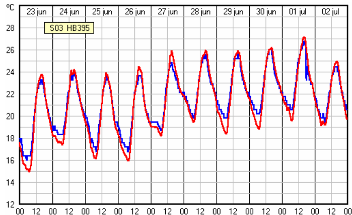
Gráfico 5.1: Comparação entre as temperaturas registradas no ponto de referencia (9) e no ponto 8, nos 10 dias monitorados.
