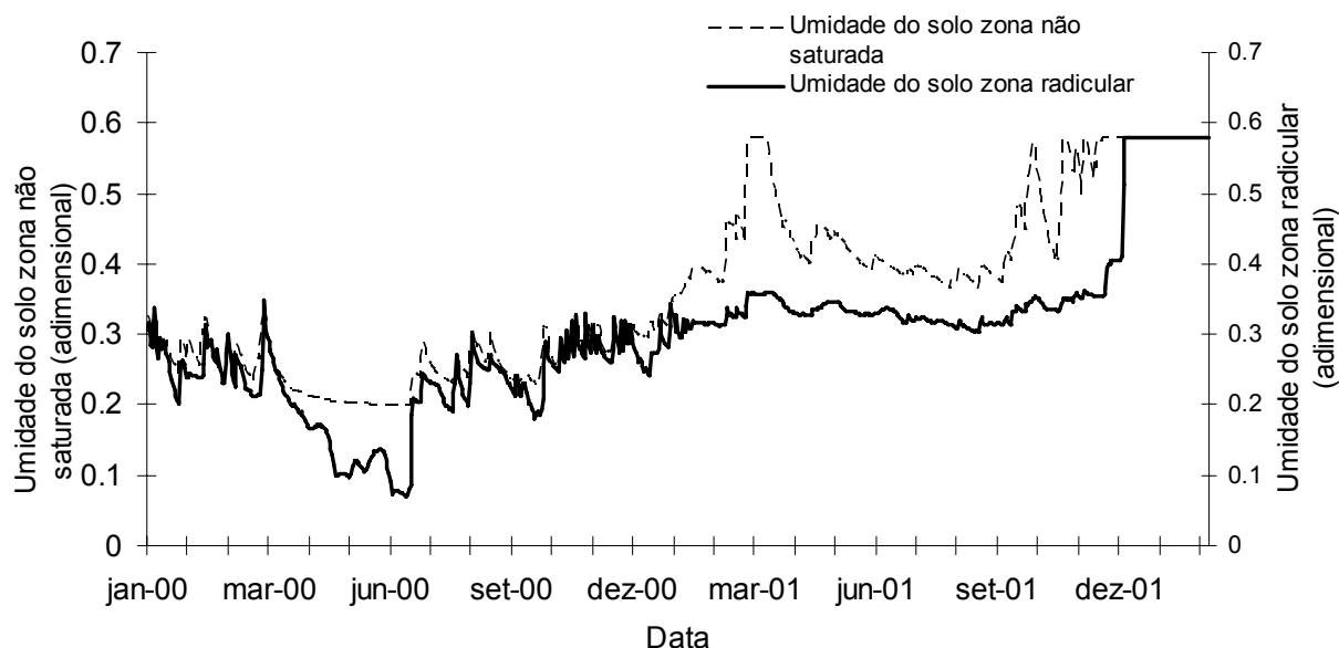
Figura 45 – Variação temporal da umidade do solo período de simulação
