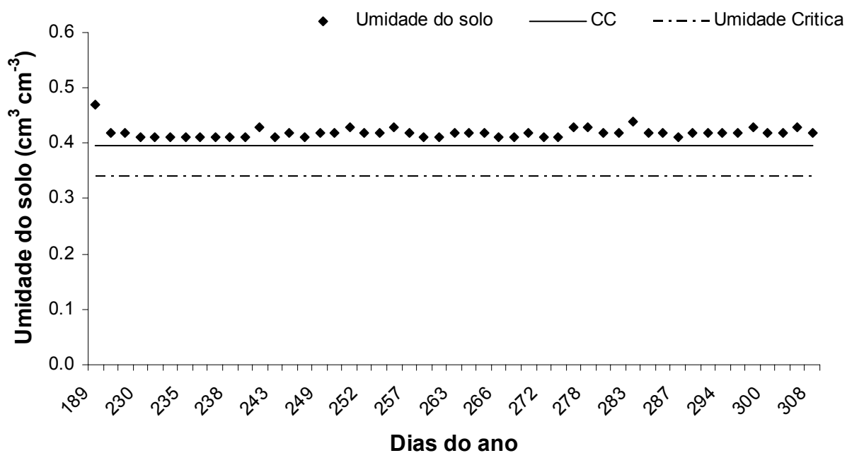
Figura 36 – Umidade do solo na área de estudo irrigada da propriedade 1, profundidade de 20-40 cm
