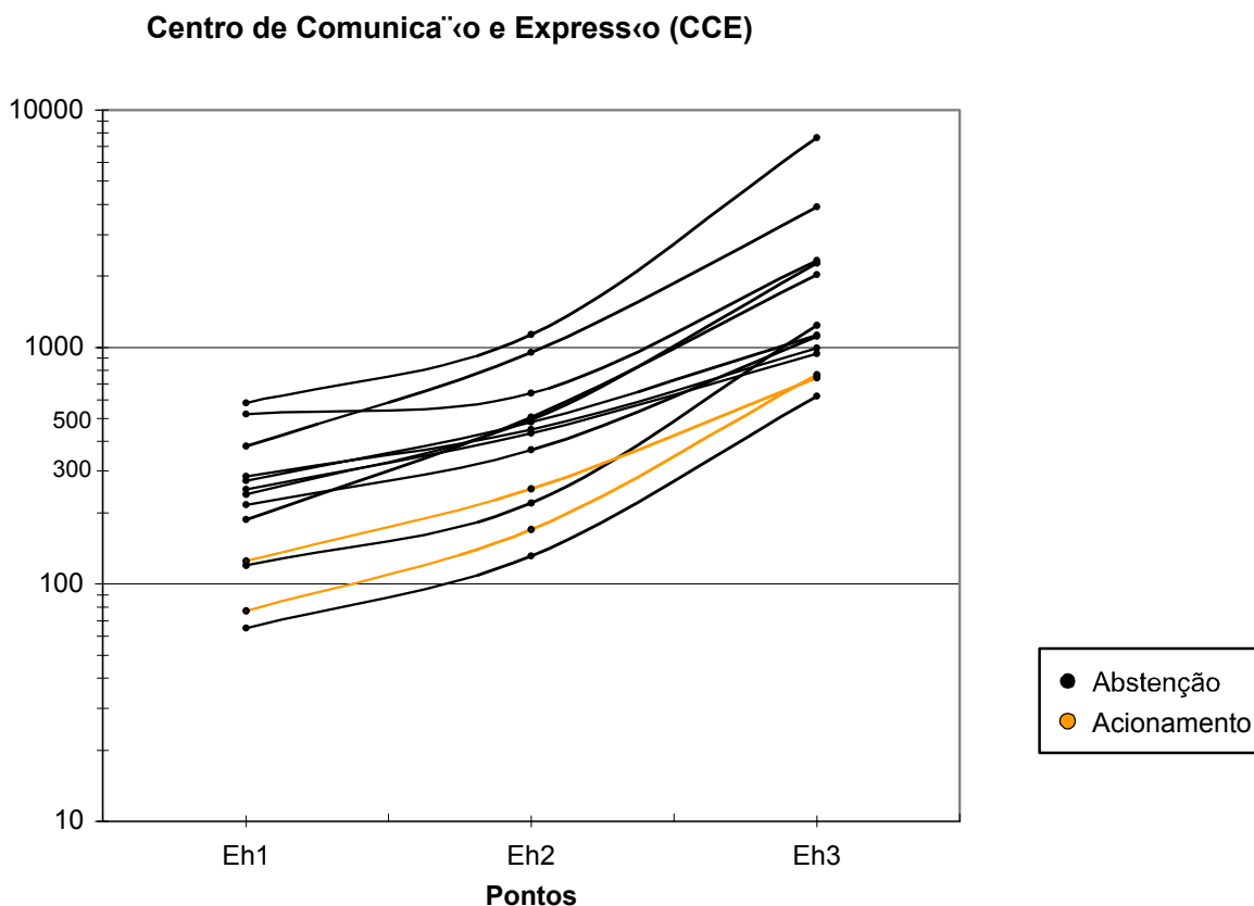
Figura 4-06. Distribuição das iluminâncias horizontais no Centro de Comunicação e Expressão.
