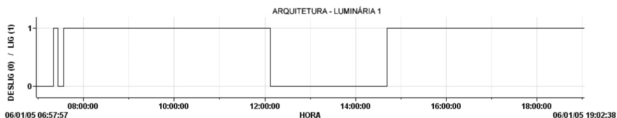
Figura 3-12. Saída de dados do sensor Hobo: acionamento e desligamento das lâmpadas.
