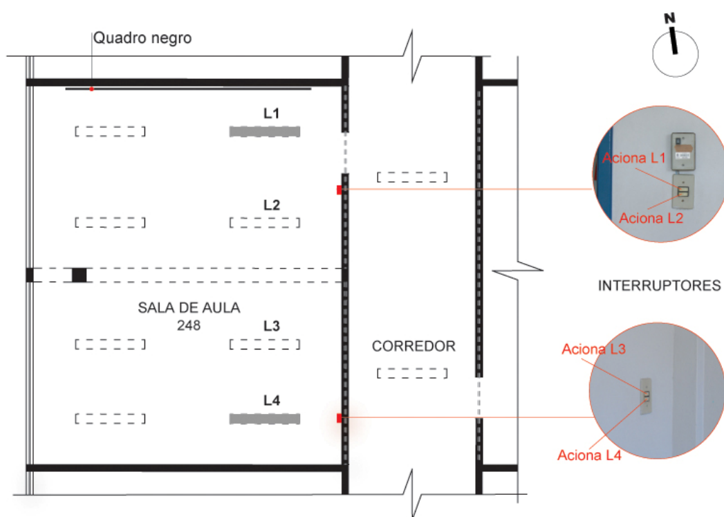
Figura 3-16. Medições na sala 248 no Centro de Comunicação e Expressão e a indicação onde foram instalados os aparelhos Hobo, em cinza.
