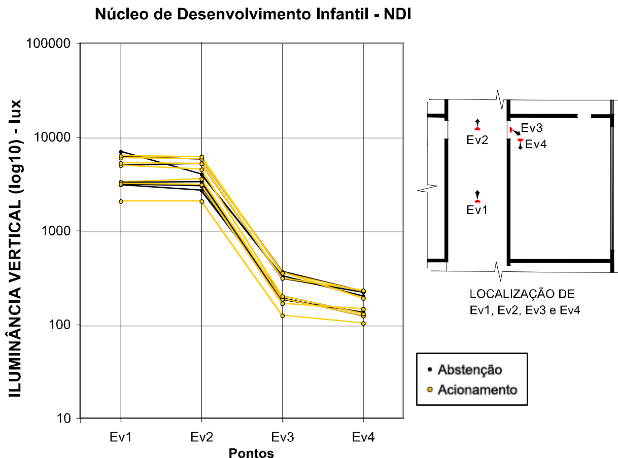
Figura 4-09. Gráfico das iluminâncias verticais - Núcleo de Desenvolvimento Infantil.
