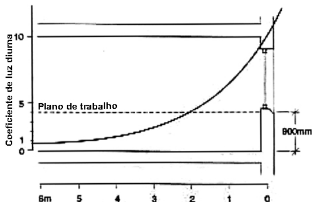
Figura 2-10. Distribuição da luz realizada por abertura lateral. Fonte: Baker e Steemers (2002).
