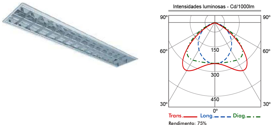
Figura 2-15. Luminária - curvas de distribuição luminosa e rendimento. Fonte: Catálogo Itaim (2000).
