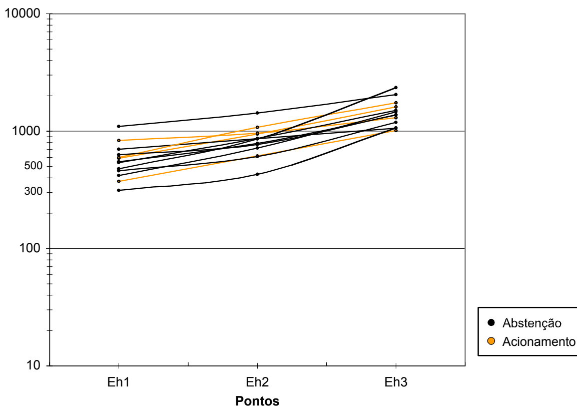
Figura 4-03. Distribuição das iluminâncias horizontais - período vespertino.
