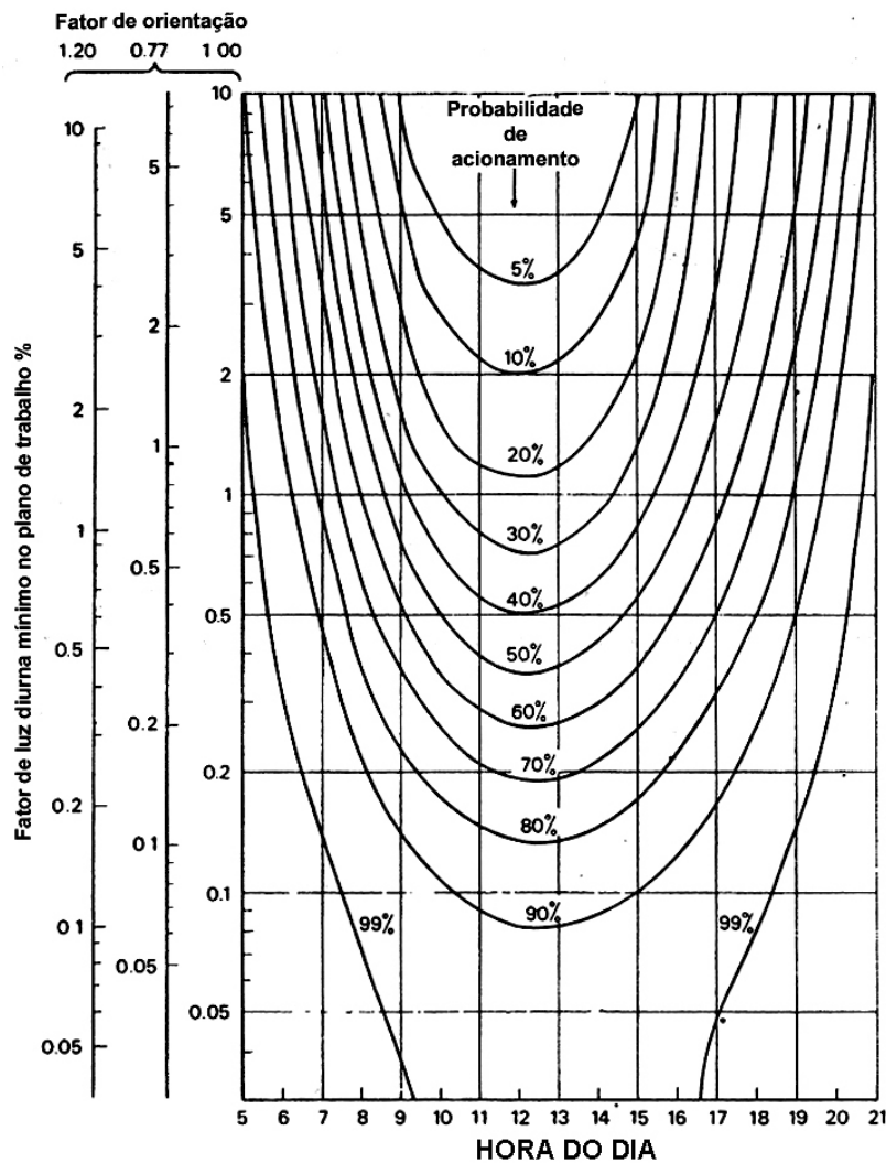
Figura 2-21. Curva de probabilidade de acionamento. Fonte: Hunt (1980).
