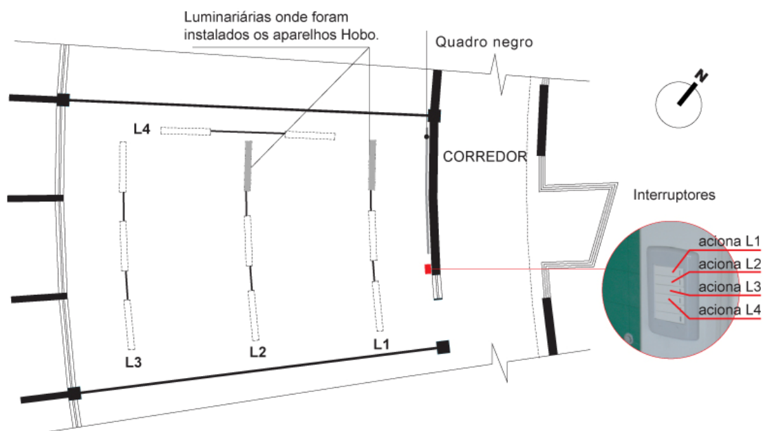
Figura 3-14. Medições na Sala ARQ-07 na Arquitetura e Urbanismo: as luminárias destacadas em cinza indicam onde foram instalados os aparelhos Hobo light on/off.
