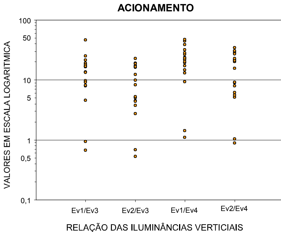
Figura 4-12. Gráfico das relações das iluminâncias verticais e acionamento.
