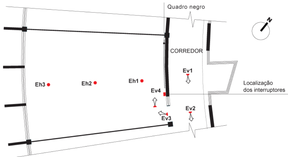
Figura 3-20. Indicação dos pontos na Arquitetura e Urbanismo – sala ARQ-07 e corredor.
