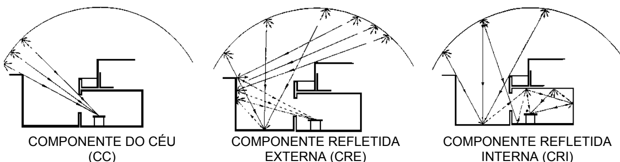
Figura 2-08. Os componentes da iluminação natural. Fonte: NBR15215-3 (2004, p. 4).
