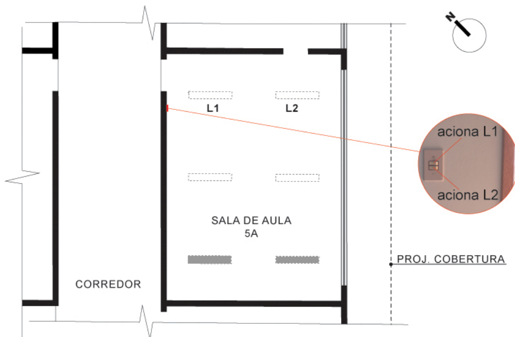
Figura 3-17. Localização dos sensores hobo light on/off na sala 5A do Núcleo de Desenvolvimento Infantil.
