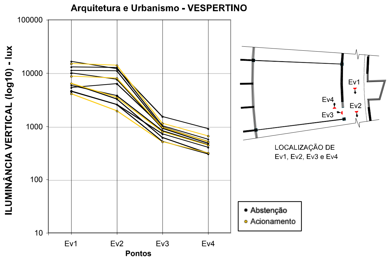
Figura 4-05. Gráfico das Iluminâncias verticais - período vespertino da Arquitetura e Urbanismo.
