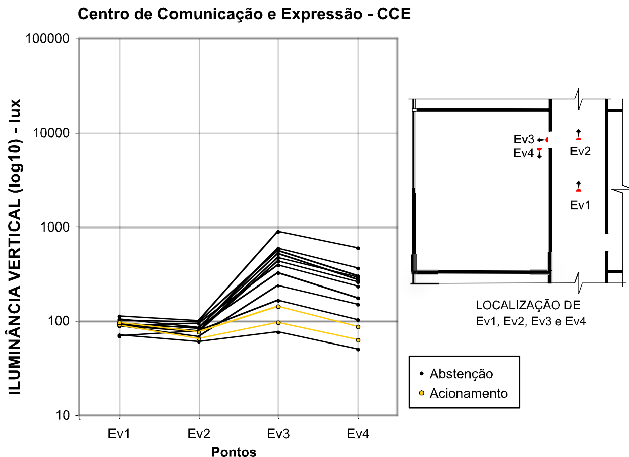
Figura 4-07. Gráfico das Iluminâncias verticais - Centro de Comunicação e Expressão.
