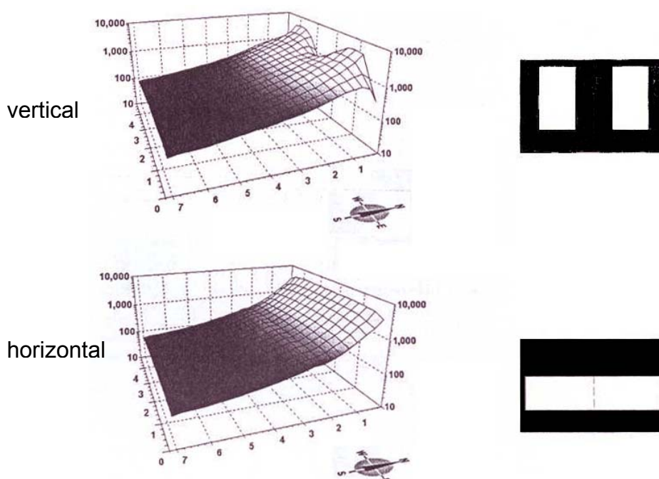
Figura 2-11. Distribuição da luz segundo a forma da janela: vertical e horizontal. (Simulação no programa computacional SUPERLITE. Modificado de Baker e Steemers (2002).
