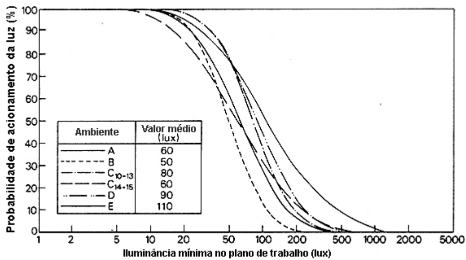
Figura 2-17. Probabilidade de acionamento por iluminância mínima no plano de trabalho para os ambientes monitorados. Fonte: Hunt (1979).
