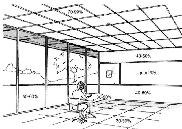
Figura 2-16. Recomendações de refletâncias para as superfícies internas de uma sala de aula. Fonte: IESNA (2000).
