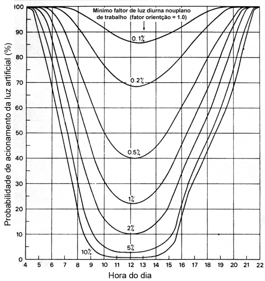
Figura 2-20. Curva de fator de luz de diurna para fator de orientação de 1.0. Fonte: Hunt (1980).
