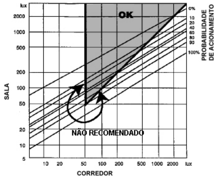
Figura 2-23. Limites para a probabilidade de acionamento calculado em função da iluminância média na sala e no corredor e os limites para um bom projeto de iluminação. Fonte: Modificado de Lynes, Littlefair e Slater (1997).
