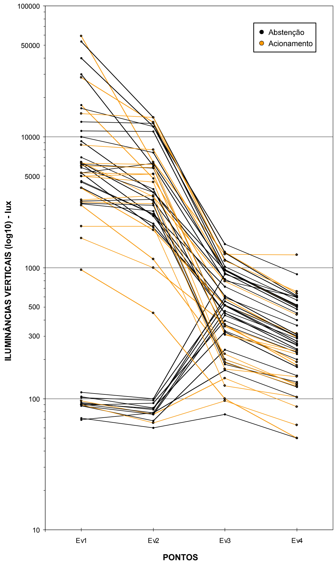
Figura 4-10. Iluminância vertical em todos os ambientes.
