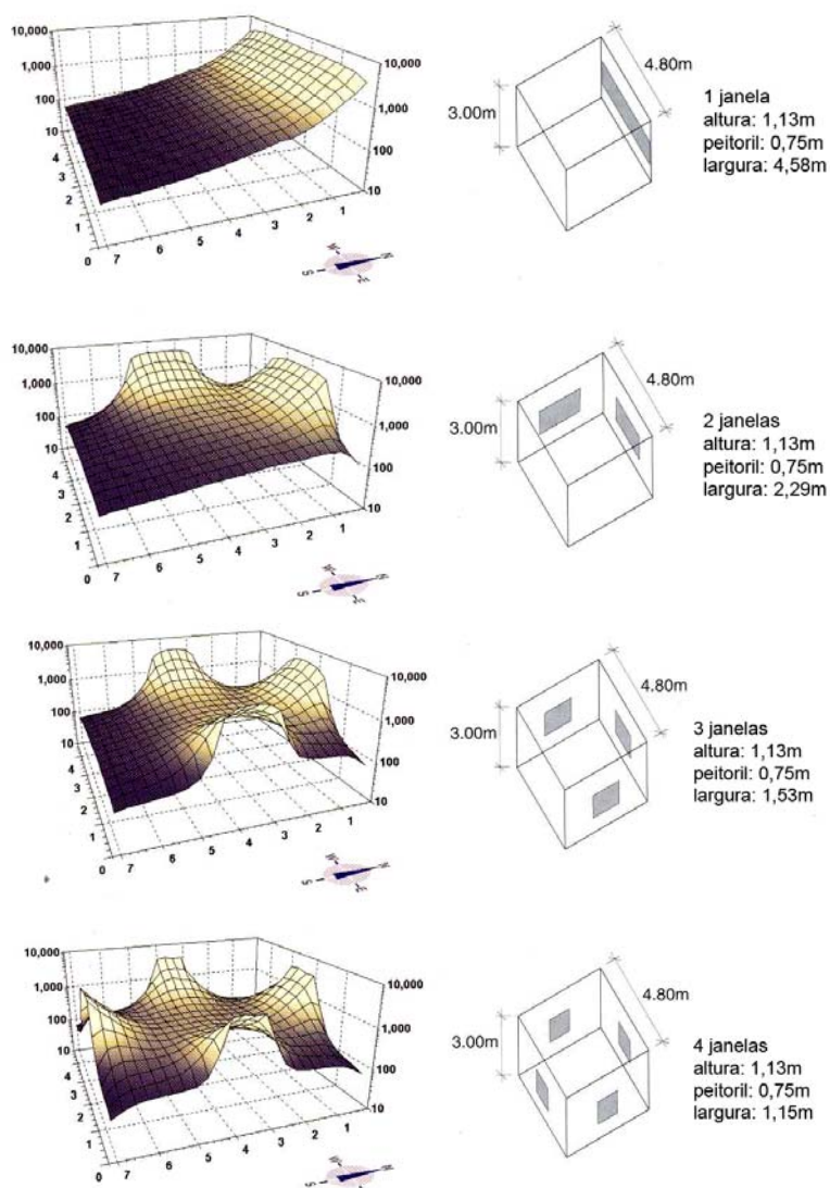
Figura 2-12. Simulação da distribuição da luz natural no programa computacional SUPERLITE. Modificado de Baker e Steemers (2002).
