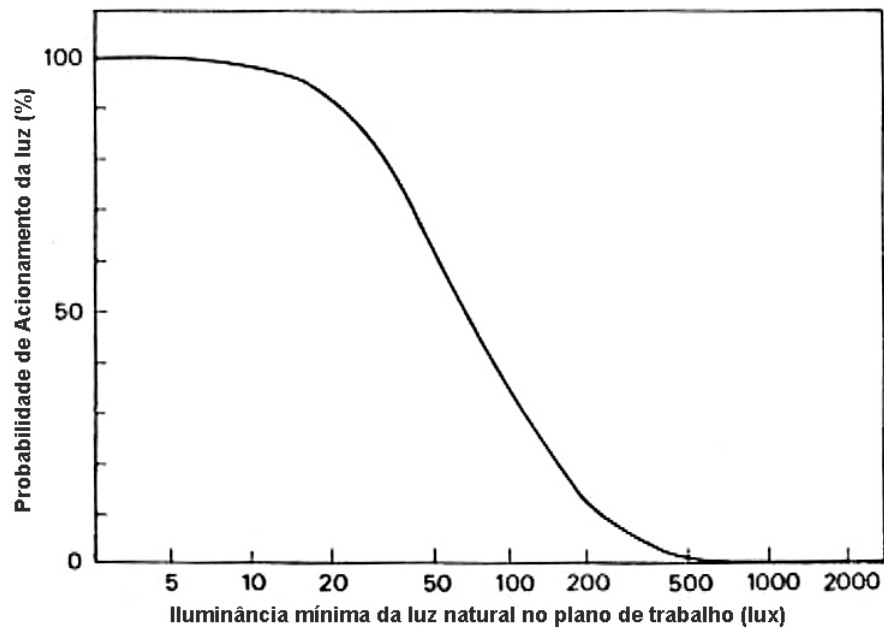
Figura 2-18. Curva representativa ajustada segundo um coeficiente de correlação. Fonte: Hunt (1980).
