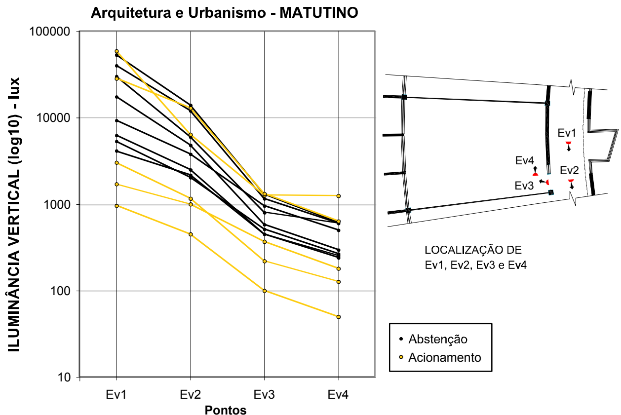
Figura 4-02. Gráfico das Iluminâncias verticais no período matutino da Arquitetura e Urbanismo.
