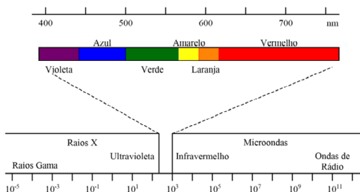
Figura 1-01. Espectro eletromagnético (comprimentos de onda em nanômetros). Fonte: Pereira e Souza, 2000.
