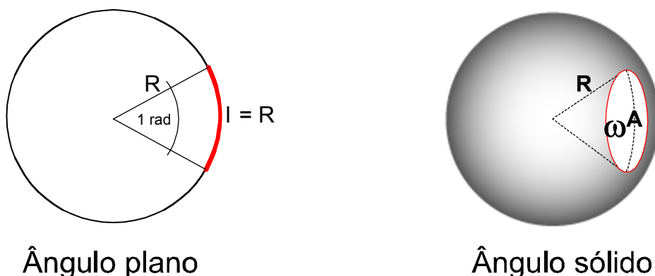
Figura 2-01. Ângulo sólido.
