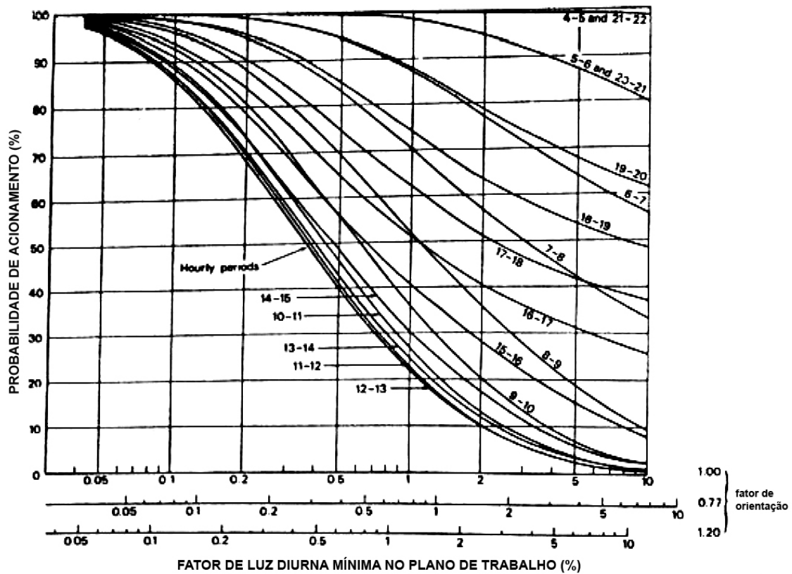
Figura 3-19. Curva Horária, probabilidade de acionamento para os 365 dias do ano. Fonte: Hunt (1980).
