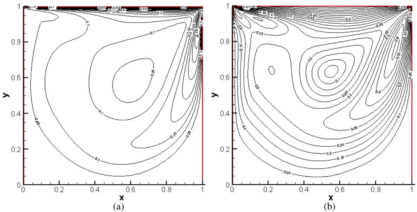
Figura 6.15: Isolinhas de Velocidade: (a) n = 0,5 , (b) n = 1,5 _ Re=500 .
