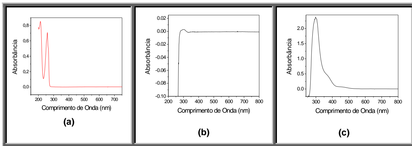
Figura 24 - Espectros de absorção na região do UV-Vis de soluções aquosas de (a) SiPy + Cl - 1 mmol.L -1 ; (b) ácido fórmico 0,5 mol.L -1 ; (c) H 2 PtCl 6 3 mmol.L -1 .
