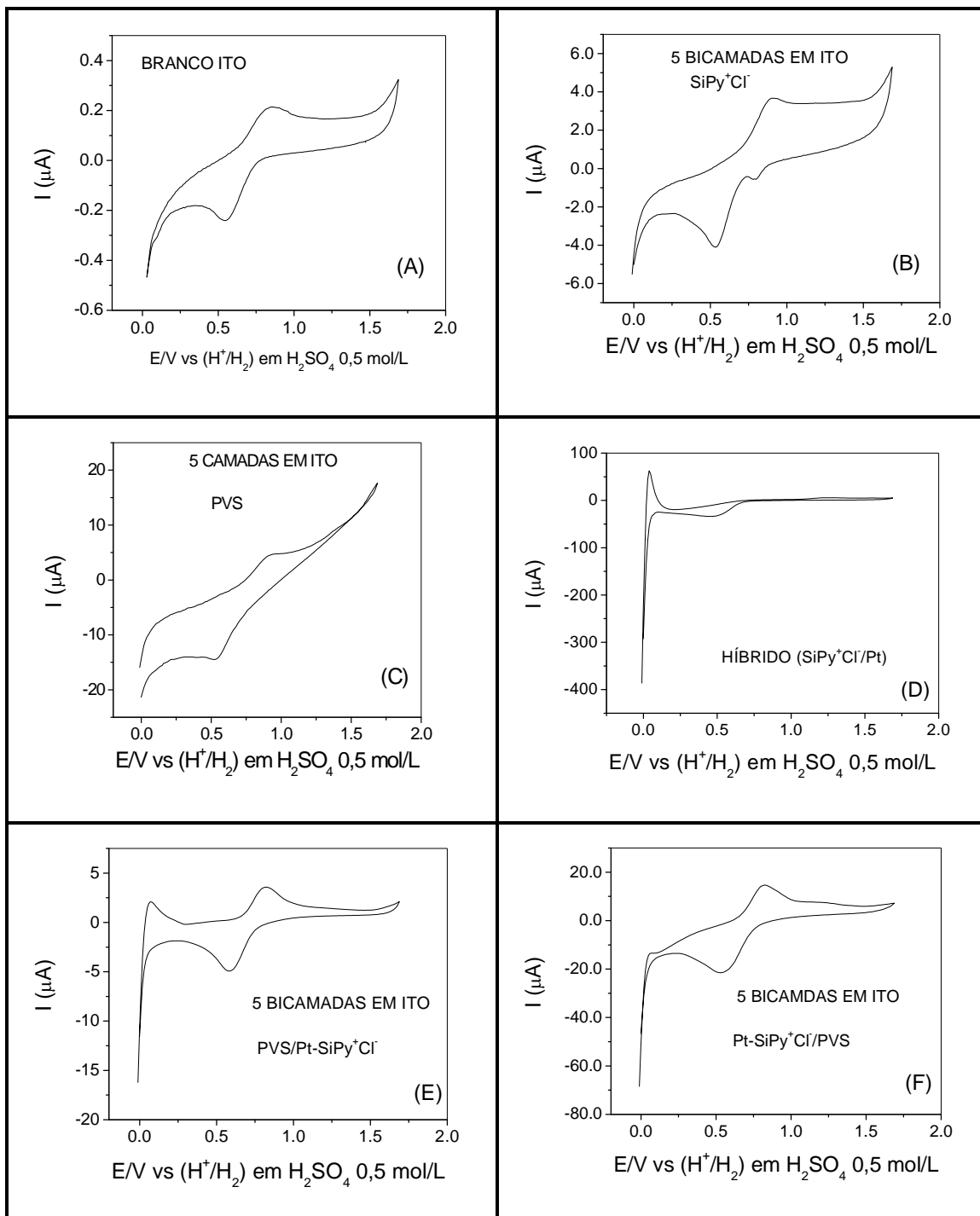
Figura 35 – Voltamogramas cíclicos dos filmes sobre substrato de ITO realizados com velocidade de varredura de 10mV.s^{-1} em solução de H_2SO_4 0,5 mol L^{-1} vs H^+/H_2 (ERH) de: (A) branco (ITO); (B) filme LbL contendo 5 camadas de SiPy^+Cl^- ; (C) filme LbL contendo 5 camadas de PVS; (D) filme LbL contendo 5 camadas do híbrido Pt/SiPy^+Cl^- ; (E) filme LbL contendo 5 bicamadas do composto PVS/SiPy^+Cl^-/Pt ; (F) filme LbL contendo 5 camadas do composto Pt/SiPy^+Cl^-/PVS .
