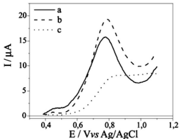
Figura 18 – Voltamograma de onda quadrada do 4-clorofenol ( 1,5 \cdot 10^{-5} mol/L, 0,1 \text{ mol} \cdot \text{L}^{-1} de tampão com pH 6, f = 100 \text{ s}^{-1} , a = 50 \text{ mV} , \Delta E_s = 2 \text{ mV} ). A) corrente resultante; b) corrente direta; c) corrente reversa [77].
