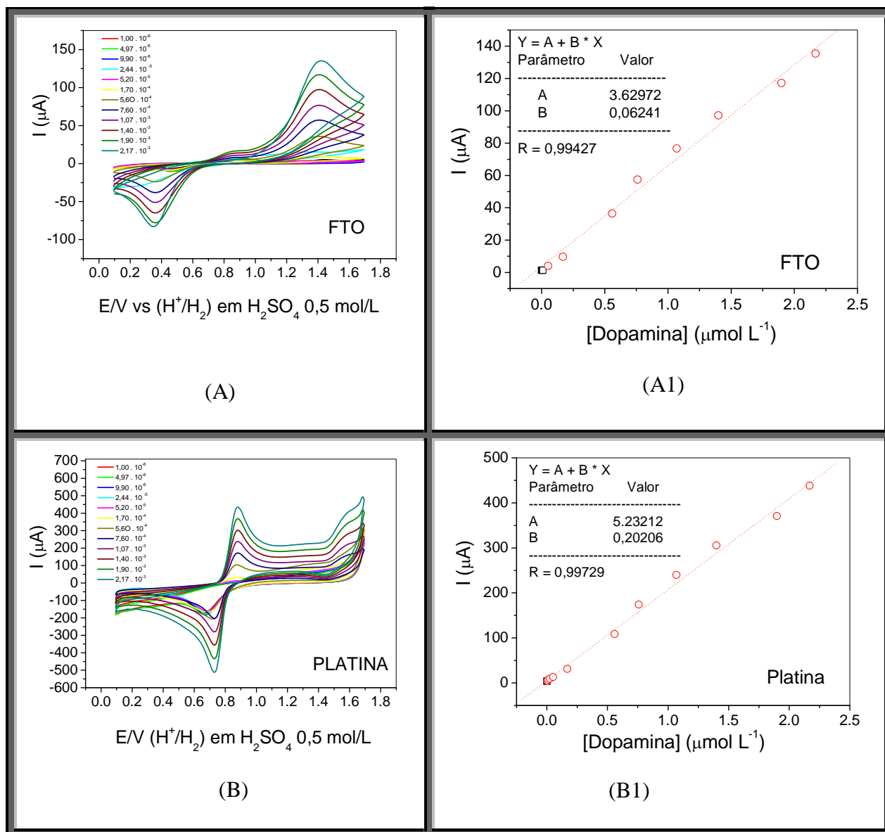
Figura 44- Voltamogramas cíclicos dos eletrodos FTO (A) e Platina (B) em diferentes concentrações de dopamina ( 1,0 \times 10^{-6} mol.L ^{-1} a 2,17 \times 10^{-3} mol.L ^{-1} ) no eletrólito de H _2 SO _4 0,5 mol.L ^{-1} estudado na velocidade de varredura de 30 mV/s. Curvas analíticas para dopamina obtida para os eletrodos FTO (A1) e Platina (B1).
