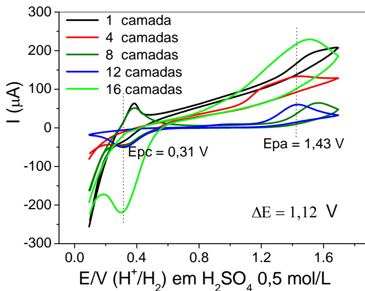
Figura 40 - Voltamogramas Cíclicos do filme de Pt-SiPy + Cl - com 1, 4, 8, 12 e 16 camadas sobrepostos na presença de DA 3,57 \cdot 10^{-4} \text{ mol.L}^{-1} utilizando \text{H}_2\text{SO}_4 0,5 \text{ mol.L}^{-1} como eletrólito suporte e velocidade de varredura de 30 mV/s.
