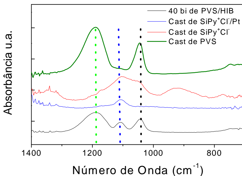
Figura 32 - Espectros de FTIR para filme automontado contendo 40 bicamadas PVS/Pt- \text{SiPy}^+\text{Cl}^- , filme cast de Pt- \text{SiPy}^+\text{Cl}^- , filme cast de \text{SiPy}^+\text{Cl}^- e filme cast de PVS
