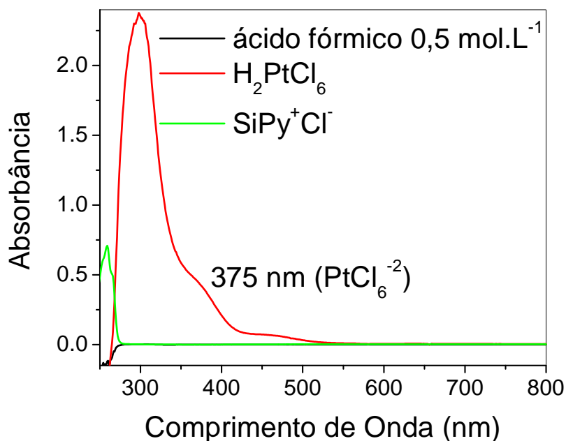
Figura 25 - Sobreposição dos espectros de UV-vis de SiPy + Cl - 1 mmol.L -1 , ácido fórmico 0,5 mol.L -1 e H 2 PtCl 6 3 mmol.L -1 .
