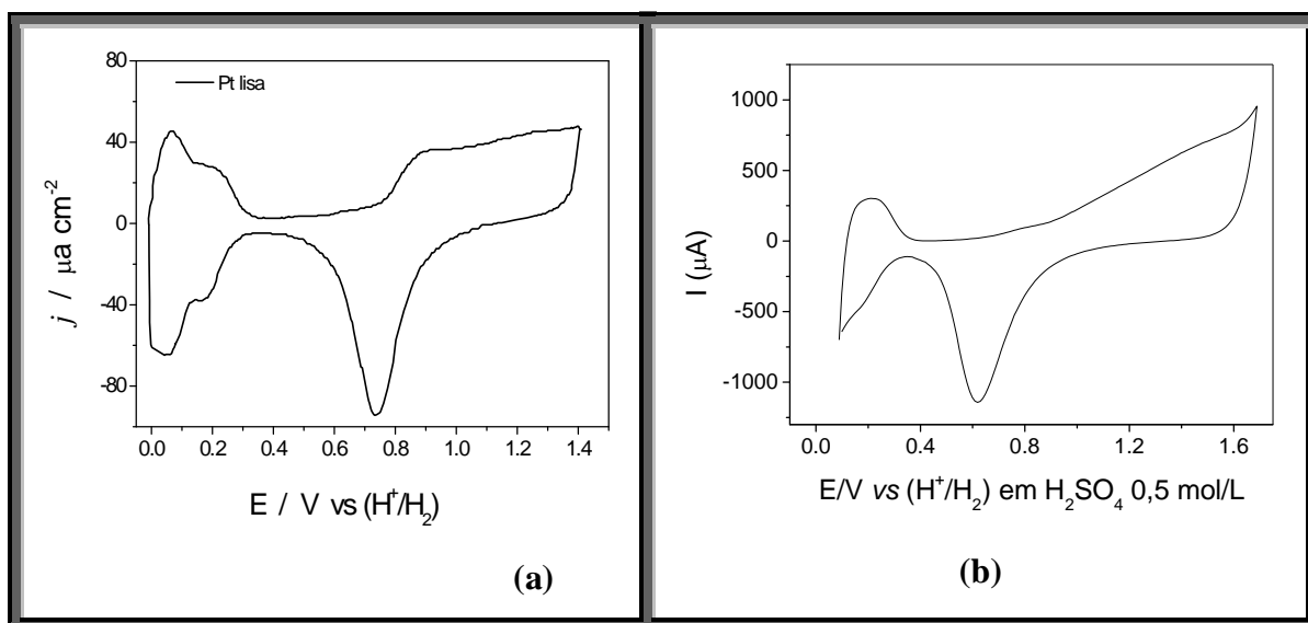
Figura 37 - Voltamogramas Cíclicos em H 2 SO 4 0,5 mol.L -1 (a) Platina pura (v = 30 mV/s e (b) filme LbL contendo 5 camadas de Híbrido (Pt-SiPy + Cl - ) sobre substrato ITO (v = 100 mV/s).
