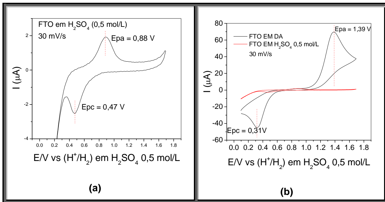
Figura 38- Voltamogramas Cíclicos de (a) FTO na presença de \text{H}_2\text{SO}_4 0,5 \text{ mol.L}^{-1} e (b) FTO na presença de \text{H}_2\text{SO}_4 0,5 \text{ mol.L}^{-1} sobreposto ao FTO na presença de DA 2,17 \cdot 10^{-3} \text{ mol.L}^{-1} utilizando \text{H}_2\text{SO}_4 0,5 \text{ mol.L}^{-1} como eletrólito suporte e velocidade de varredura de 30 \text{ mV/s} .
