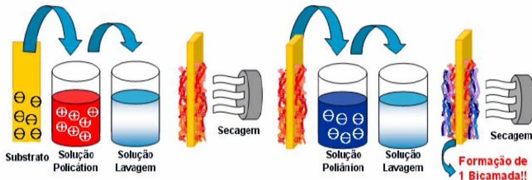
Figura 4 - Representação esquemática do processo de fabricação de filmes finos pela técnica de automontagem [4].
