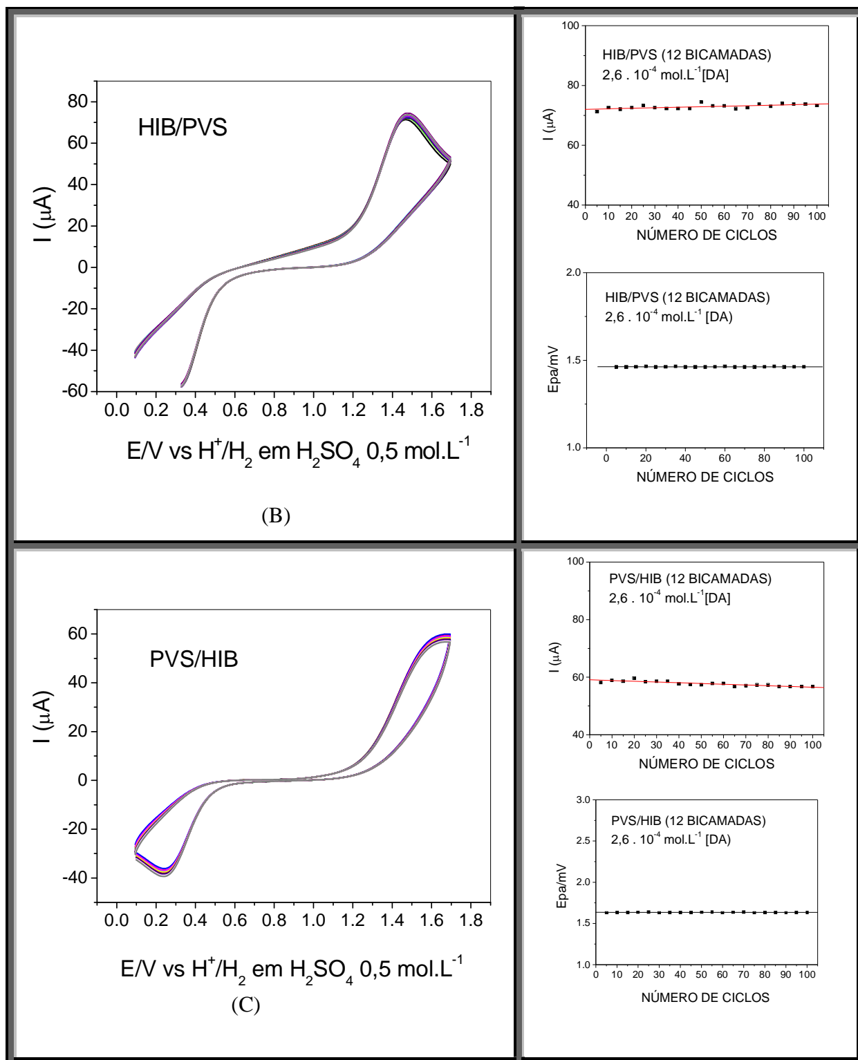
Figura 50 – Voltamogramas cíclicos de (A) Híbrido, (B) HIB/PVS e (C) PVS/HIB, em 2,6 \times 10^{-4} \text{ mol.L}^{-1} de dopamina, no eletrólito de \text{H}_2\text{SO}_4 0,5 \text{ mol.L}^{-1} , velocidade de varredura 50 \text{ mV/s} . Gráficos à direita: correlação entre a corrente de pico anódica e o número de ciclos, e potencial de pico anódico e número de ciclos para os eletrodos de Filmes LbL de Híbrido, HIB/PVS e PVS/HIB.
