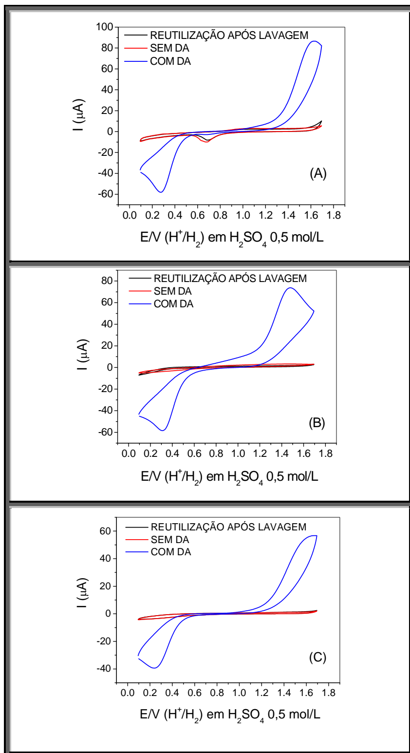
Figura 49- Voltamogramas Cíclicos de (A) Híbrido, (B) HIB/PVS e (C) PVS/HIB, sem DA, com DA 2,6 \cdot 10^{-4} \text{ mol.L}^{-1} e após lavagem. Eletrólito suporte \text{H}_2\text{SO}_4 0,5 mol.L ^{-1} e v = 50 \text{ mV s}^{-1} .
