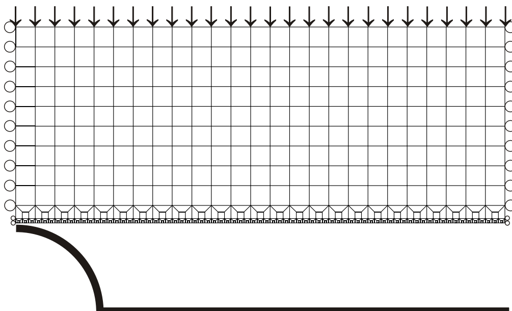
Figura 56: Modelo para análise com elemento finito
