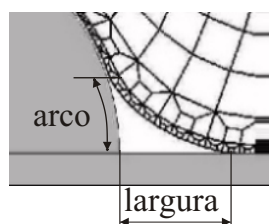
Figura 58: Geometria da zona de não-aderência
