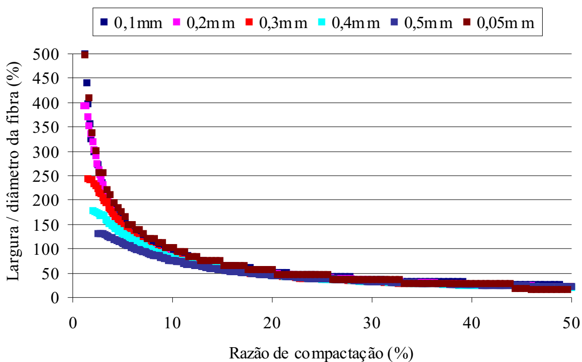
Figura 61: Razão da largura do defeito pelo diâmetro da fibra em função da razão de compactação
