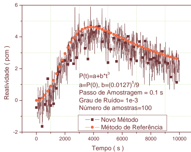
Figura 6.18 Variação de reatividade necessária para reproduzir a variação da potência nuclear, na forma P(t) = P(0) + b * t^3 , passo de amostragem igual a 0.1 s, número de amostras de 100 e com um grau de ruído de \sigma=0.001 .
