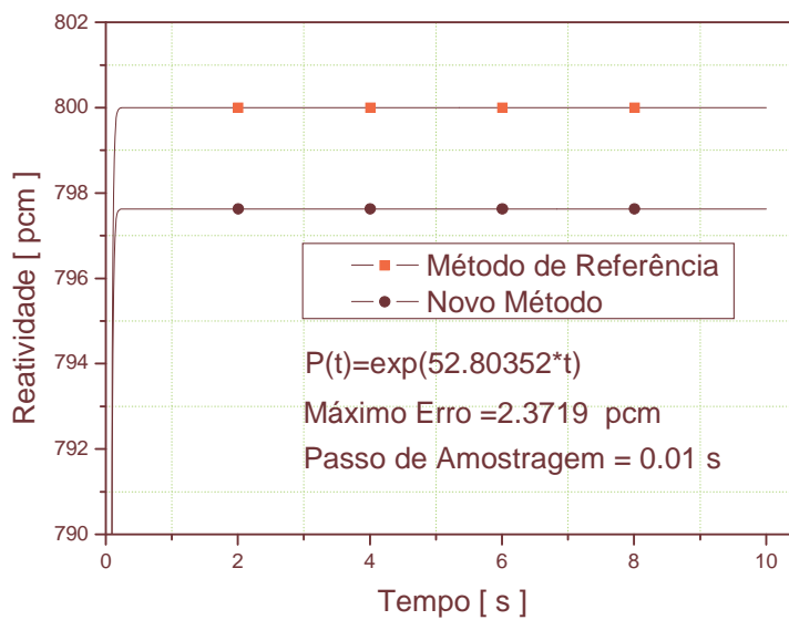
Figura 6.13 Variação de reatividade necessária para reproduzir a variação da potência nuclear, na forma P(t)=\exp(\omega \cdot t) , com \omega igual 52.80352. Passo de amostragem igual a 0.01 s
