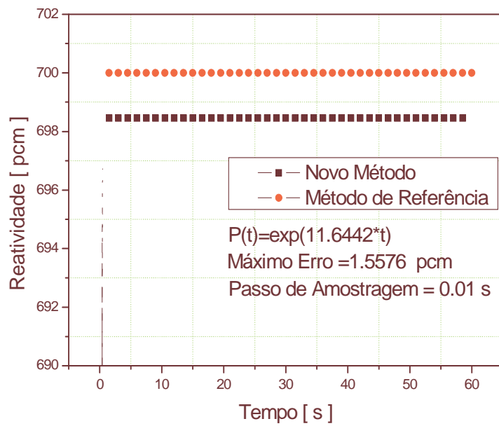
Figura 6.12 Variação de reatividade necessária para reproduzir a variação da potência nuclear, na forma P(t)=\exp(\omega \cdot t) , com \omega igual 11.6442. Passo de amostragem igual a 0.01 s.
