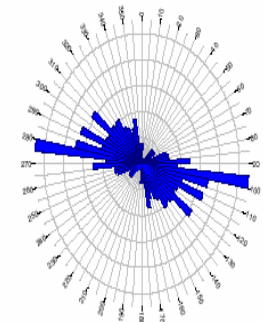
Figura 14 - Diagrama de rosea p/ lineamentos obtidos a partir da CC 1(R)3(G)4(B). Total (N) = 64
