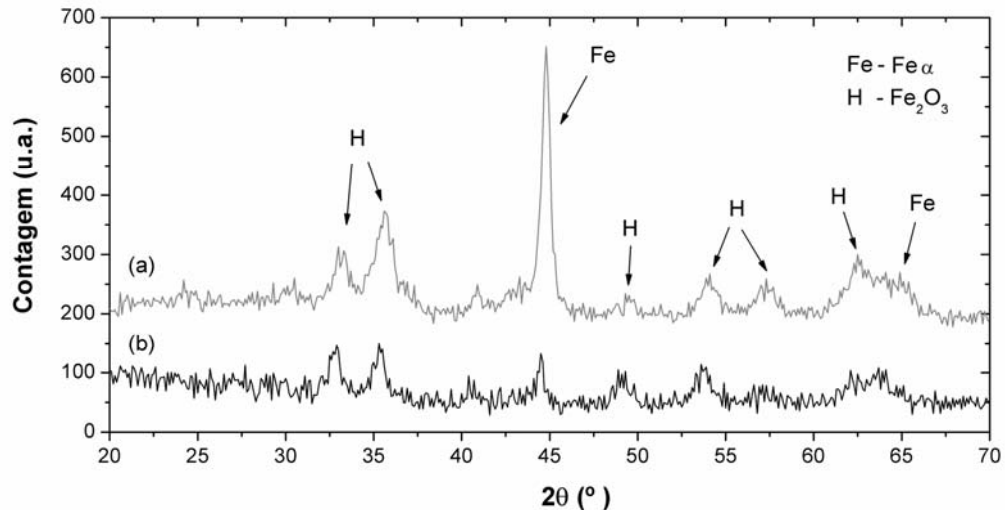
Figura 5.22 – Espectros de difração de raios X dos fragmentos da amostra que apresentou elevado (a) e baixo (b) valor de desgaste relativo.
