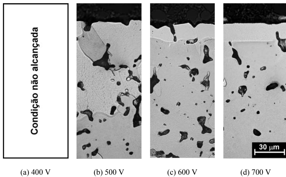
Figura 4.27 – Micrografias das amostras sinterizadas a 1150°C com t_{on} de 100 \mu s e tensões negativas de pico de 500 V (b), 600 V (c) e 700 V (d). A condição de 400 V (a) não foi alcançada.
