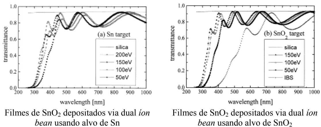
Figura 6.3 – Transmitância de diversos filmes de SnO 2 (Chung, 1999).
