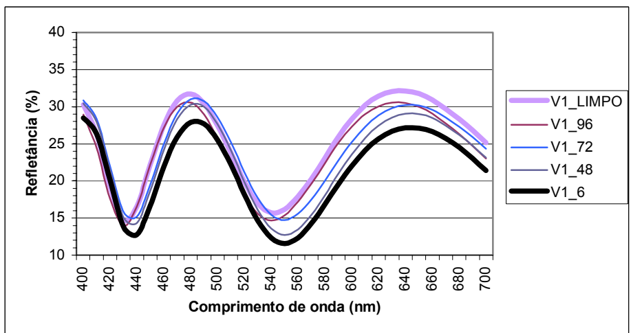
Figura 7.40 – Refletância de placas de vidro versus tempo de exposição à luz ultravioleta para visualizar a degradação do azul de metileno sobre vidro com filme de TiO 2 depositado durante 15 minutos.
