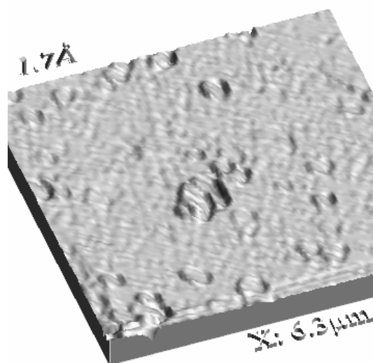
(b) Imagem 3D da superfície do vidro com uma área de 6,3 \mu\text{m} por 6,3 \mu\text{m} . Rugosidade na ordem de unidade de Ångström.
