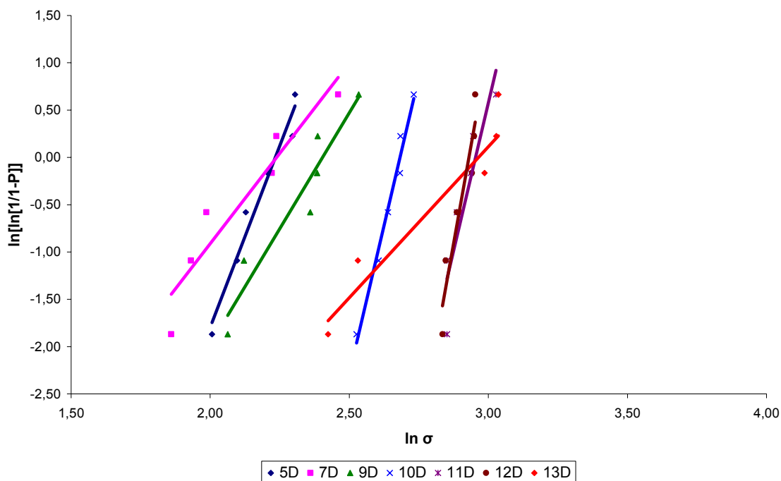
FIGURA 11 – GRÁFICO DE WEIBULL DAS 7 COMPOSIÇÕES – 7 DIAS.
