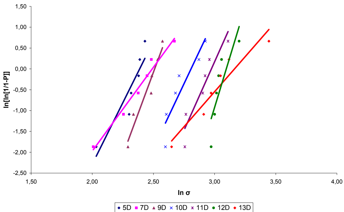
FIGURA 13 – GRÁFICO DE WEIBULL DAS 7 COMPOSIÇÕES – 28 DIAS.
