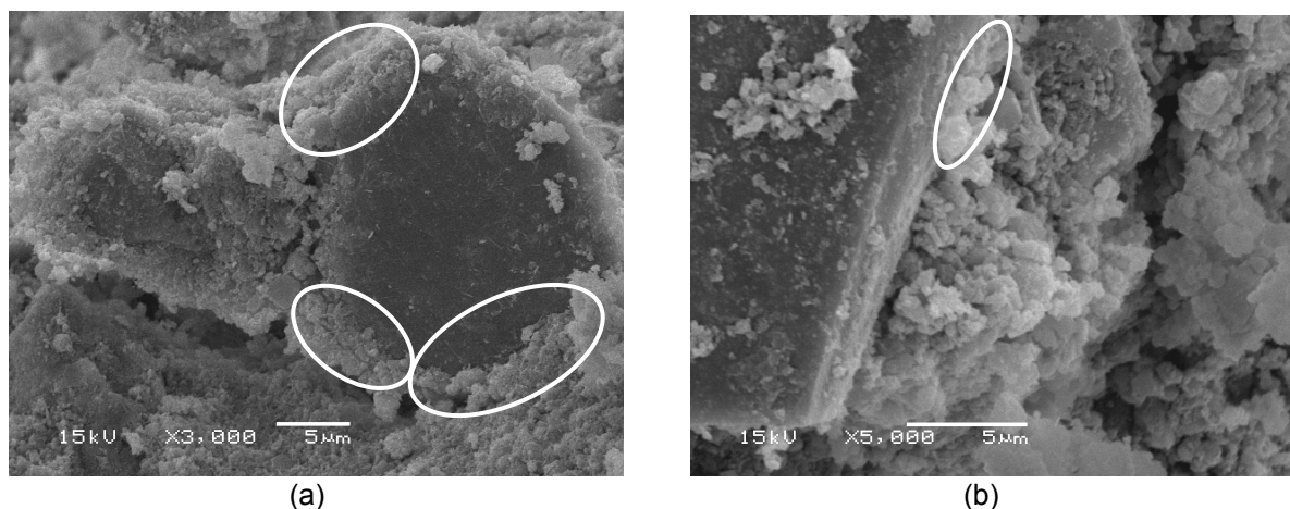
FIGURA 32 – MICROGRAFIAS DA COMPOSIÇÃO 11D 3 DIAS – 3.000x(a) e 5.000x(b).
