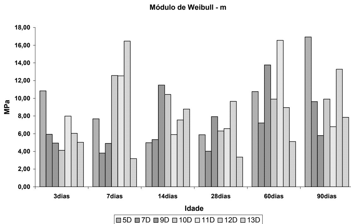
FIGURA 18 – MÓDULO DE WEIBULL - RESISTÊNCIA x IDADE.
