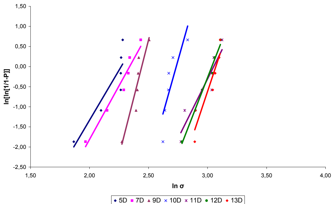
FIGURA 12 – GRÁFICO DE WEIBULL DAS 7 COMPOSIÇÕES – 14 DIAS.
