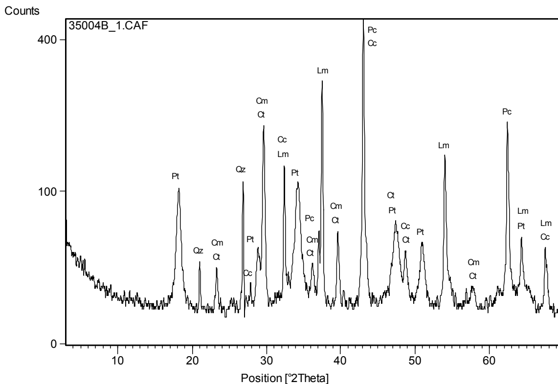
FIGURA 21 - DIFRATOGRAMA DE RAIOS X DO RESÍDUO DE PRODUÇÃO DE CAL
