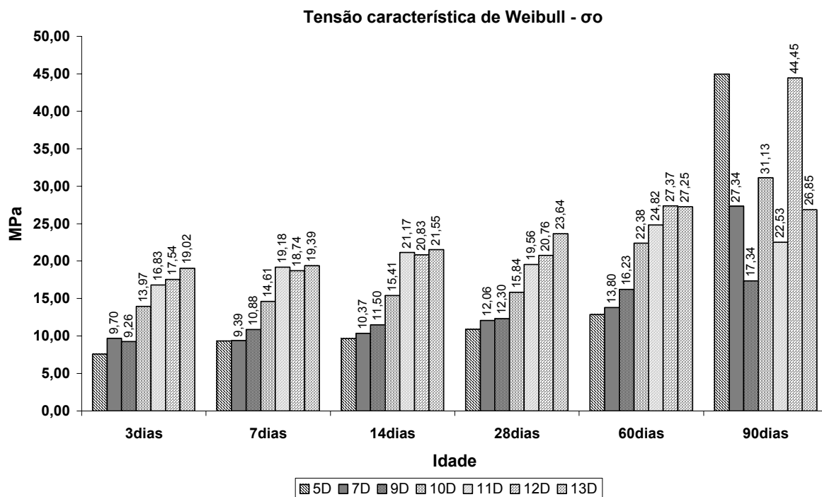
FIGURA 17 – TENSÃO CARACTERÍSTICA DE WEIBULL – RESISTÊNCIA x IDADE.
