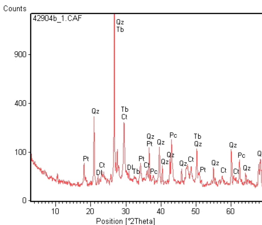
FIGURA 24 – DIFRATOGRAMA DE RAIOS X DA COMPOSIÇÃO 11D – 28 DIAS.
