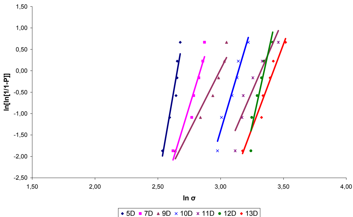
FIGURA 15 – GRÁFICO DE WEIBULL DAS 7 COMPOSIÇÕES – 90 DIAS.
