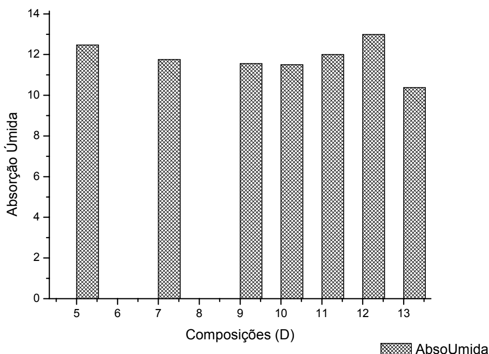
FIGURA 19 – GRÁFICO ABSORÇÃO x COMPOSIÇÃO.
