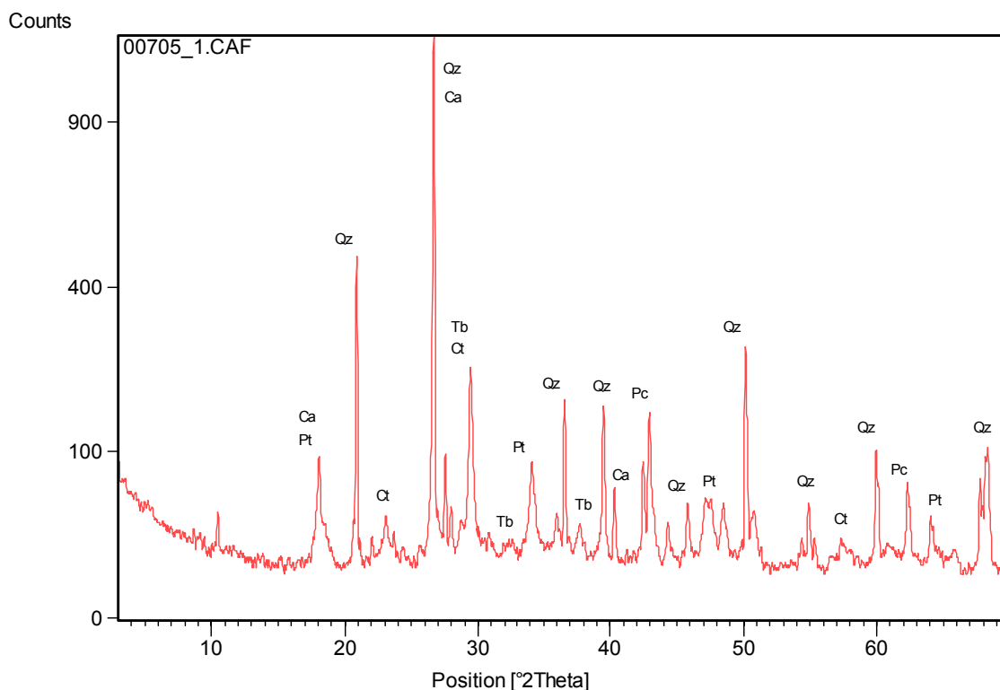
FIGURA 25 – DIFRATOGRAMA DE RAIOS DA COMPOSIÇÃO 11D – 90 DIAS.
