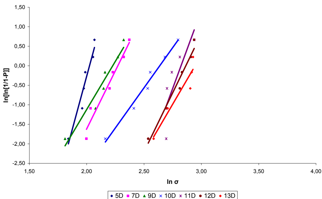
FIGURA 10 – GRÁFICO DE WEIBULL DAS 7 COMPOSIÇÕES – 3 DIAS.
