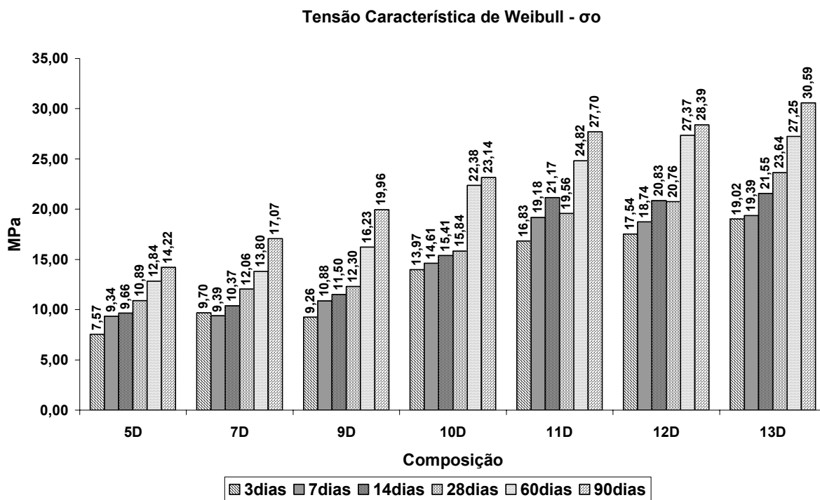
FIGURA 16 – TENSÃO CARACTERÍSTICA DE WEIBULL – RESISTÊNCIA x COMPOSIÇÃO.
