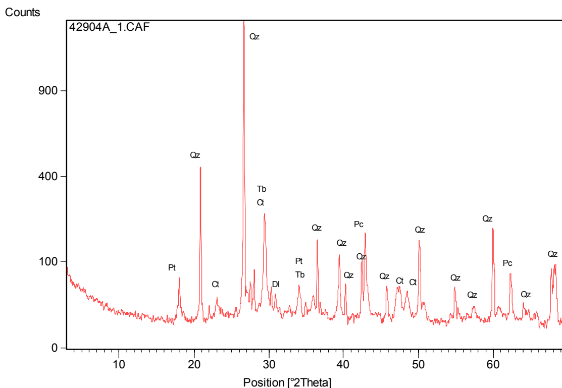
FIGURA 23 – DIFRATOGRAMA DE RAIOS X DA COMPOSIÇÃO 11D – 3 DIAS.
