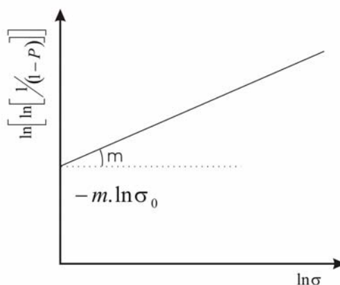
FIGURA 9 – MODELO ESQUEMÁTICO DO DIAGRAMA DE WEIBULL.
