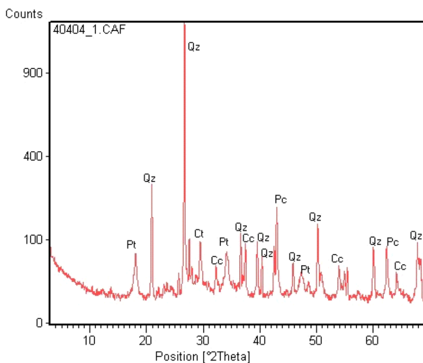
FIGURA 22 – DIFRATOGRAMA DE RAIOS X DA COMPOSIÇÃO 11D SECA.
