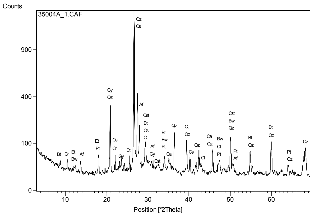
FIGURA 20 – DIFRATOGRAMA DE RAIOS X DO RESÍDUO DE CONCRETO.
