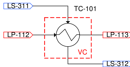
FIGURA 18. VOLUME DE CONTROLE DO TROCADO DE CALOR TC-101.
