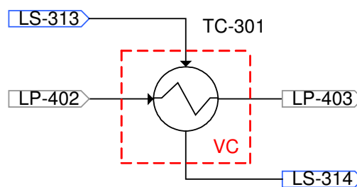
FIGURA 19. VOLUME DE CONTROLE DO TROCADO DE CALOR TC301.
