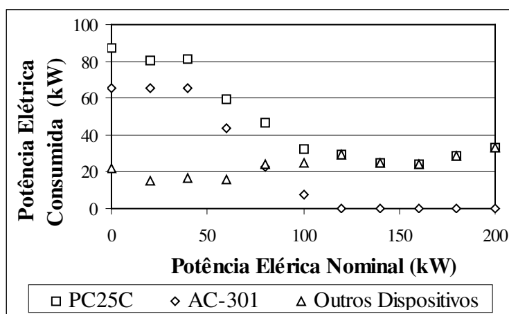
FIGURA 25. POTÊNCIA ELÉTRICA CONSUMIDA.
