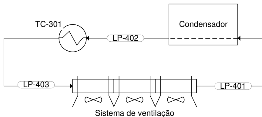
FIGURA 20. SISTEMA DE REFRIGERAÇÃO.
