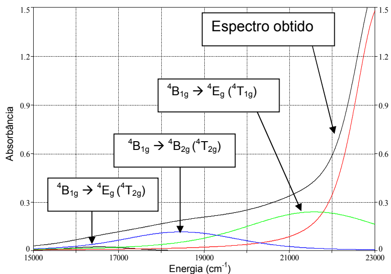
FIGURA C.1. Análise por deconvolução para o complexo Cr(3,5-Clsalen) 1 \times 10^{-3} \text{ mol L}^{-1} para o espectro eletrônico em DMSO.
