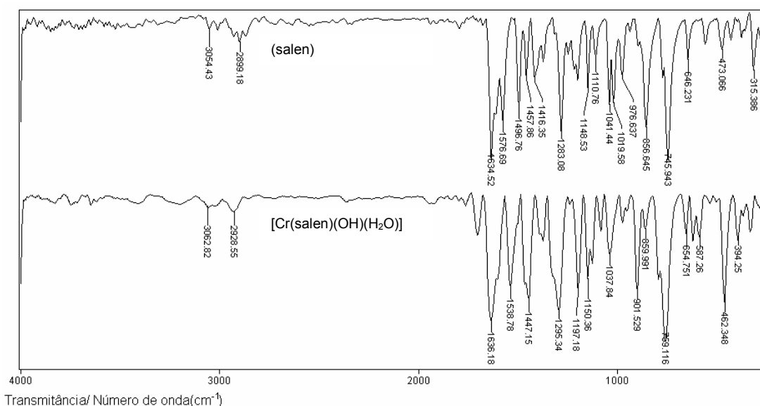
FIGURA A.1. Espectro na região do infravermelho do ligante (salen) e do complexo [Cr(salen)(OH)(H 2 O)], na região compreendida entre 4000 e 250 cm -1 , com resolução 4 cm -1 utilizando pastilhas de KBr (1 mg do composto para 100 mg de KBr) com as amostras do ligante e do complexo.
