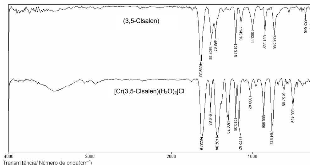
FIGURA 4.2. Espectro na região do infravermelho do ligante (3,5-Clsalen) e do complexo [Cr(3,5-Clsalen)(H 2 O) 2 ]Cl, na região compreendida entre 4000 e 250 cm -1 , com resolução 4 cm -1 utilizando pastilhas de KBr (1 mg do composto para 100 mg de KBr) com as amostras do ligante e do complexo.
