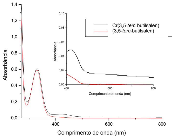
FIGURA B.7. Espectros eletrônicos na região do ultravioleta-visível para o ligante (3,5-terc-butilsalen) e complexo Cr(3,5-terc-butilsalen) em solvente DMSO concentração 1 \times 10^{-4} \text{ mol L}^{-1} , com expansão na região acima de 400 nm.
