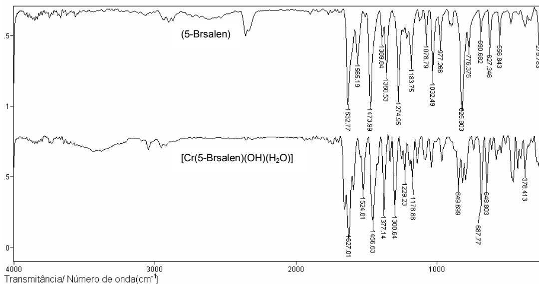
FIGURA A.2. Espectro na região do infravermelho do ligante (5-Brsalen) e do complexo [Cr(5-Brsalen)(OH)(H 2 O)], na região compreendida entre 4000 e 250 cm -1 , com resolução 4 cm -1 utilizando pastilhas de KBr (1 mg do composto para 100 mg de KBr) com as amostras do ligante e do complexo.
