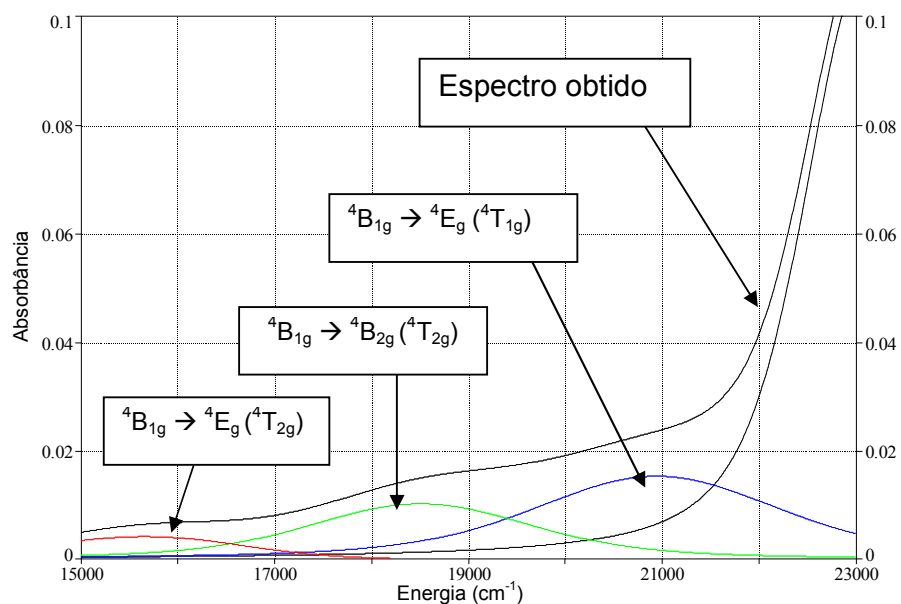
FIGURA C.4. Análise por deconvolução para o complexo \text{Cr}(5\text{-Clisalen}) 1 \times 10^{-4} \text{ mol L}^{-1} para o espectro eletrônico em DMSO.
