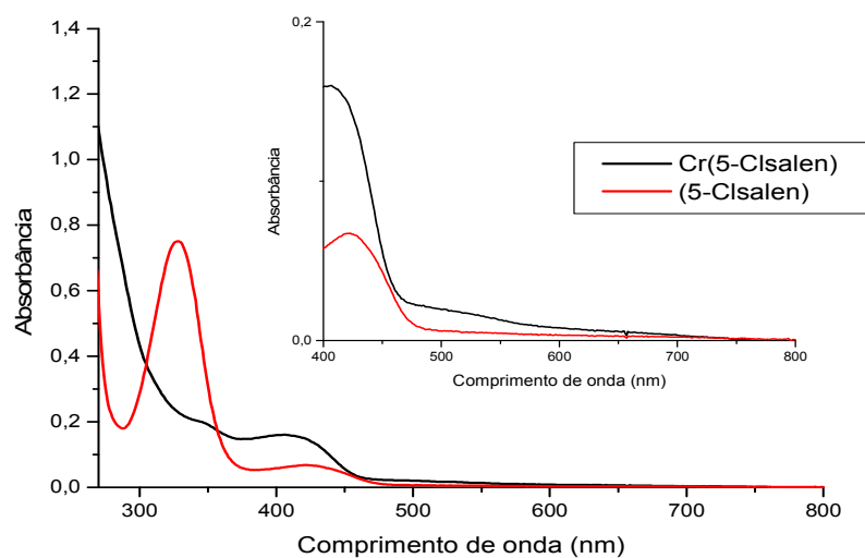
FIGURA B.1. Espectros eletrônicos na região do ultravioleta-visível para o ligante (5-Clisalen) e complexo Cr(5-Clisalen) em solvente DMSO concentração 1 \times 10^{-4} \text{ mol L}^{-1} , com expansão na região acima de 400 nm.
