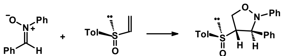
FIGURA 1.3. Reações de adição 1,3-dipolar com vinil sulfóxidos [47] .
