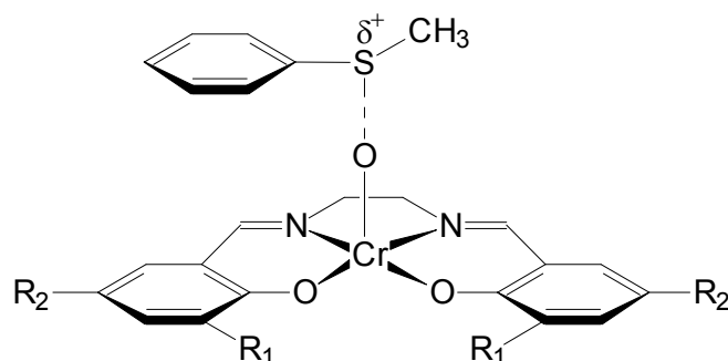
FIGURA 4.15. Estado de transição proposto para o ataque eletrofilico do oxigênio do catalisador ao enxofre nucleófilo do substrato [11,81] , R 1 e R 2 são os grupos substituintes no anel.
