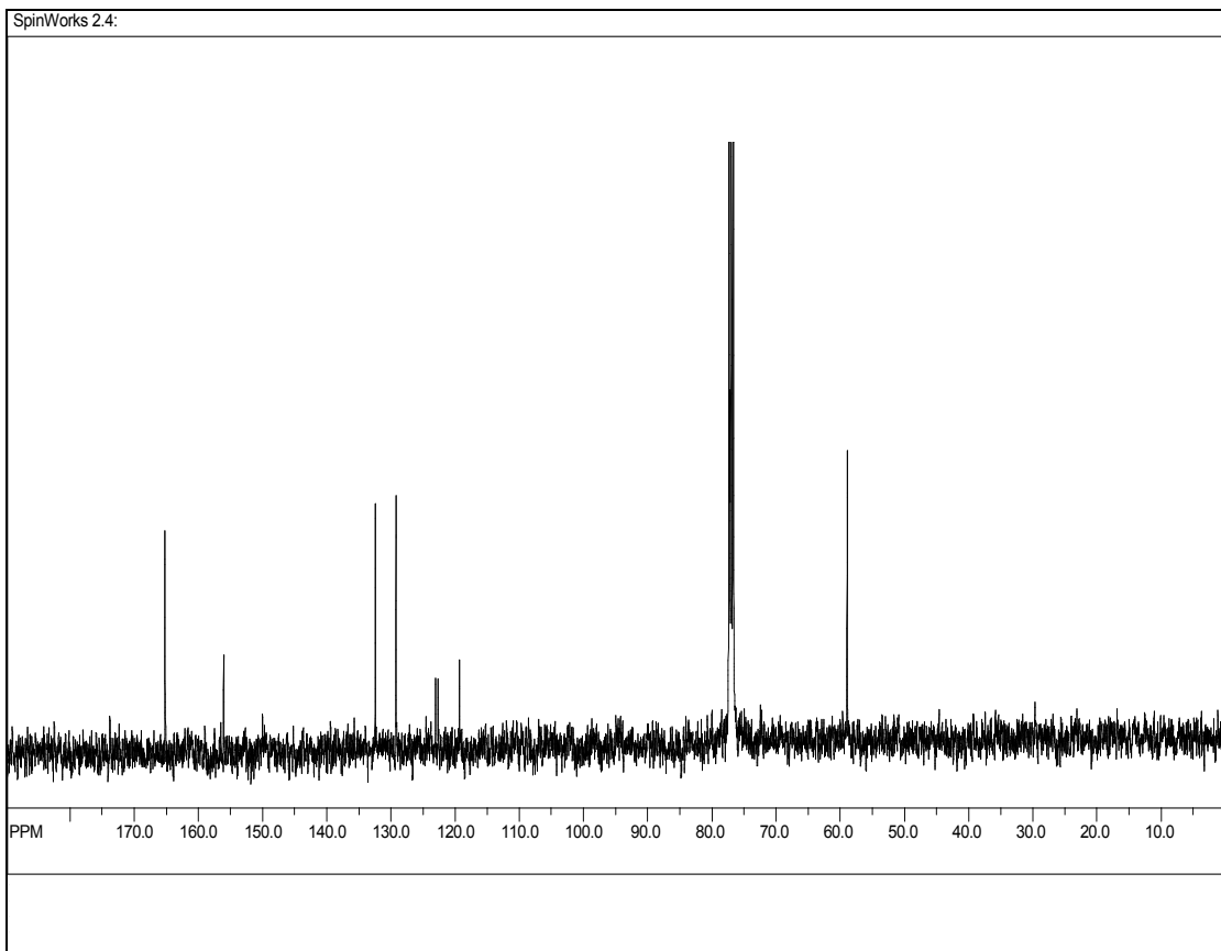
FIGURA E.4. Espectro ^{13}\text{C} RMN do ligante (3,5-Cl 2 salen) utilizando como solvente \text{CDCl}_3 e como padrão interno TMS.
