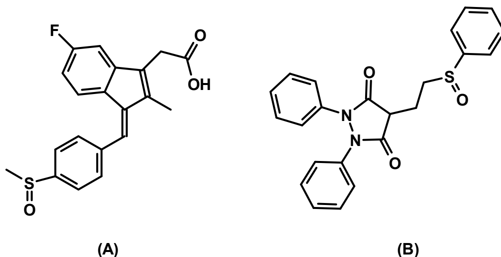
FIGURA 1.2. Exemplos de sulfóxidos utilizados como drogas (Sulindac- (A) e Sulfinpirazona –(B) ) [54] .
