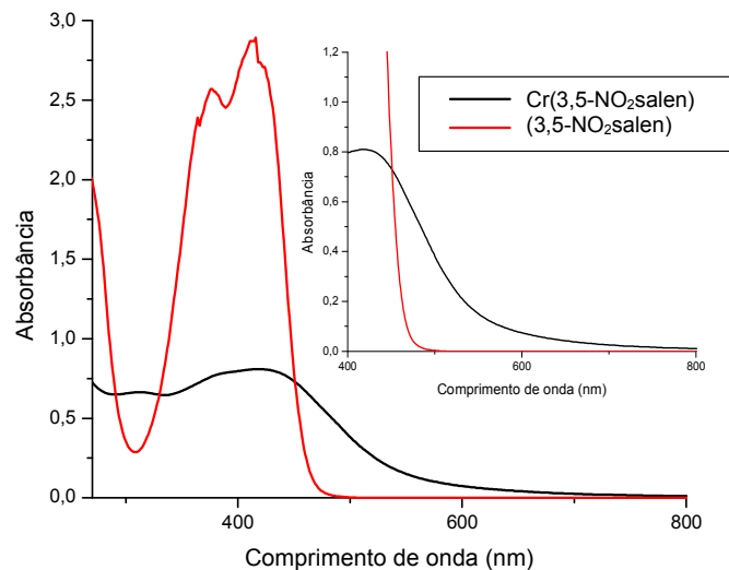
FIGURA B.9. Espectros eletrônicos na região do ultravioleta-visível para o ligante (3,5-NO 2 salen) e complexo Cr(3,5-NO 2 salen) em solvente DMSO concentração 1x 10 -4 mol L -1 , com expansão na região acima de 400 nm.
