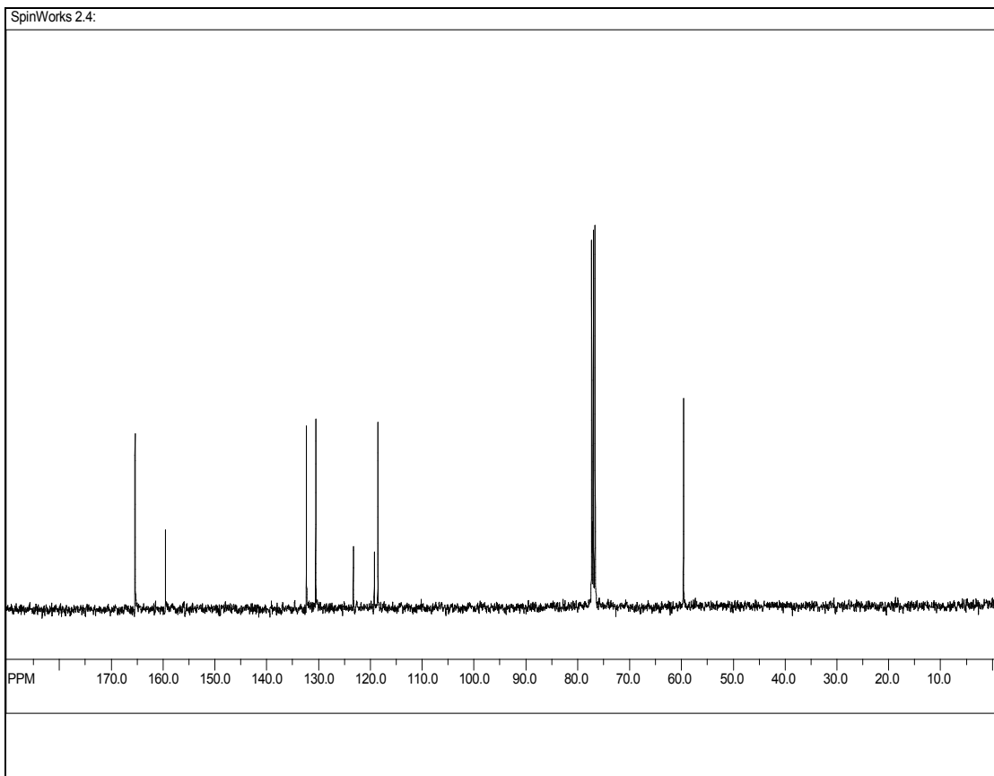
FIGURA E.1. Espectro ^{13}\text{C} RMN do ligante (5-Clisalén) utilizando como solvente \text{CDCl}_3 e como padrão interno TMS.
