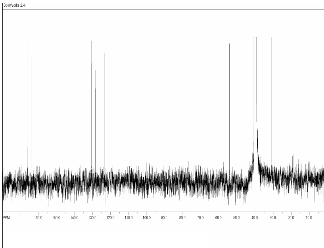
FIGURA E.6. Espectro ^{13}\text{C} RMN do ligante (5-NO 2 salen) utilizando como solvente DMSO deuterado e como padrão interno TMS.
