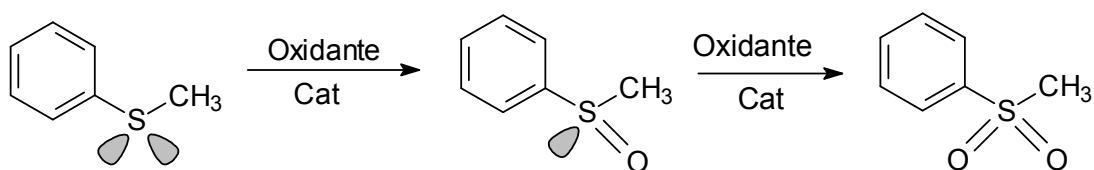
FIGURA 3.3. Reação proposta da oxidação de fenilmetilsulfeto [51] .
