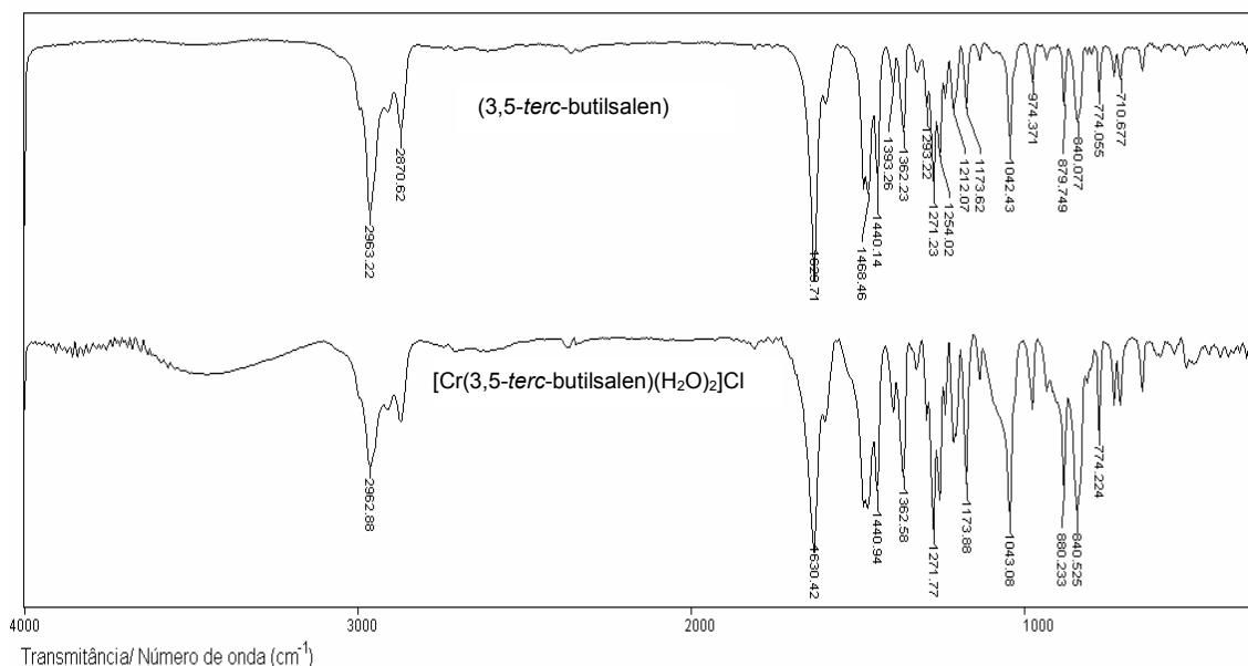
FIGURA A.7. Espectro na região do infravermelho do ligante (3,5- tert -butilsalen) e do complexo [\text{Cr}(3,5\text{-}i\text{tert-butilsalen})(\text{H}_2\text{O})_2]\text{Cl} , na região compreendida entre 4000 e 250 \text{cm}^{-1} , com resolução 4 \text{cm}^{-1} utilizando pastilhas de KBr (1 mg do composto para 100 mg de KBr) com as amostras do ligante e do complexo.
