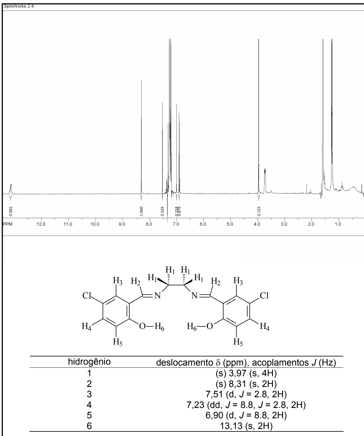
FIGURA D.2. Espectro ^1\text{H} RMN do ligante (5-Cl-salen) utilizando como solvente \text{CDCl}_3 e como padrão interno TMS.
