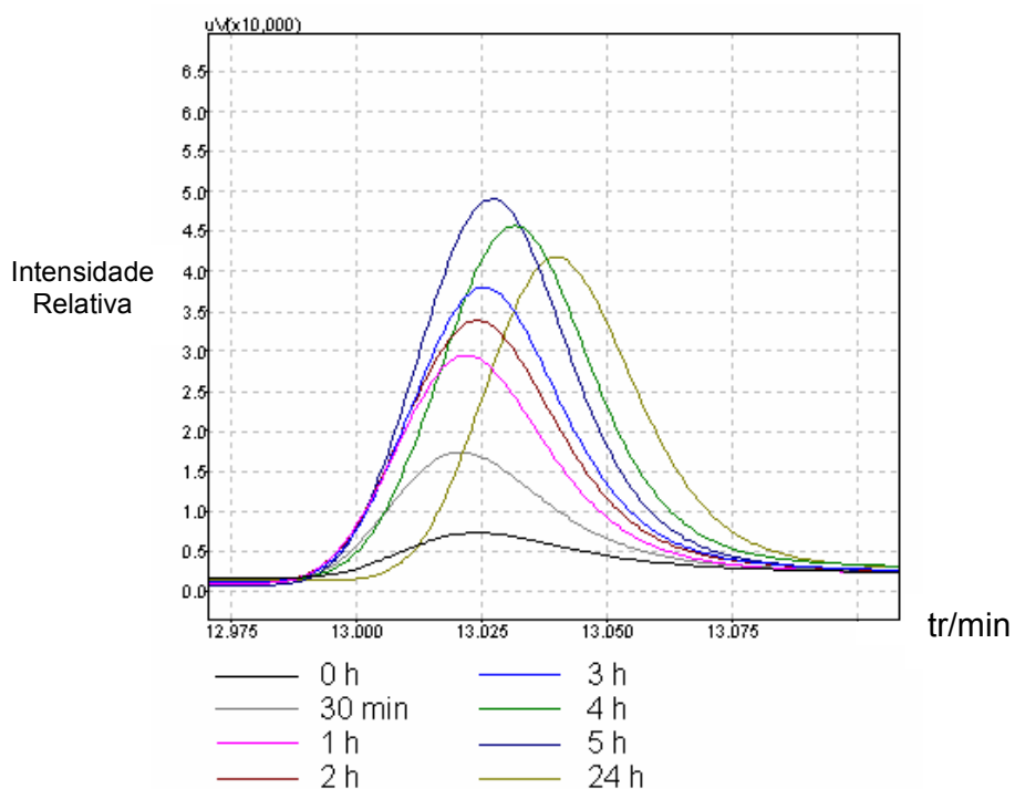
FIGURA 4.13. Cromatograma das alíquotas de 1\mu\text{L} retiradas das reações de oxidação do fenilmetilsulfeto utilizando como oxidante o PhIO e como catalisador o complexo [\text{Cr}(\text{salen})(\text{OH})(\text{H}_2\text{O})] , os sinais mostrados são referentes ao produto fenilmetilsulfóxido.
