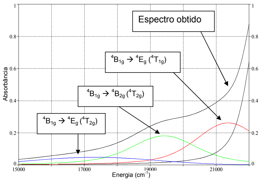
FIGURA C.2. Análise por deconvolução para o complexo Cr(3,5-Brsalen) 1 \times 10^{-3} \text{ mol L}^{-1} para o espectro eletrônico em DMSO.
