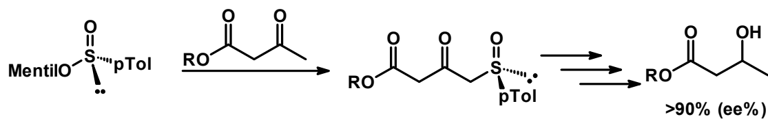
FIGURA 1.5. Redução seletiva de compostos \beta -dicarbonílicos [49] .
