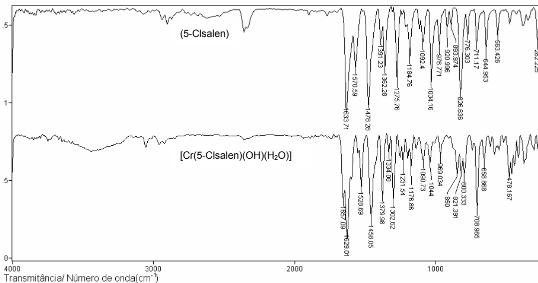
FIGURA A.3. Espectro na região do infravermelho do ligante (5-Clisalen) e do complexo [Cr(5-Clisalen)(OH)(H 2 O)], na região compreendida entre 4000 e 250 cm -1 , com resolução 4 cm -1 utilizando pastilhas de KBr (1 mg do composto para 100 mg de KBr) com as amostras do ligante e do complexo.
