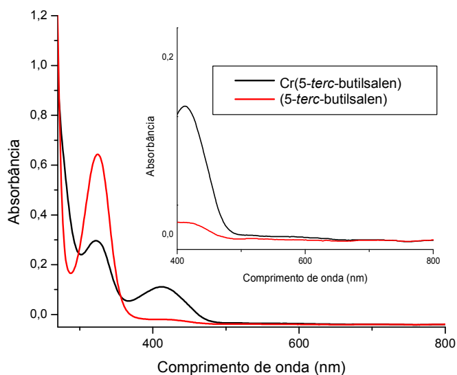
FIGURA B.4. Espectros eletrônicos na região do ultravioleta-visível para o ligante (5- tert -butylsalen) e complexo Cr(5- tert -butylsalen) em solvente DMSO concentração 1 \times 10^{-4} \text{ mol L}^{-1} , com expansão na região acima de 400 nm.
