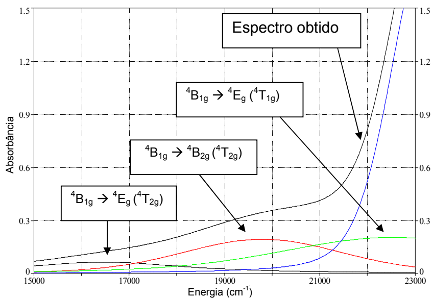
FIGURA C.3. Análise por deconvolução para o complexo \text{Cr}(3,5\text{-Isalen}) 1 \times 10^{-3} \text{ mol L}^{-1} para o espectro eletrônico em DMSO.
