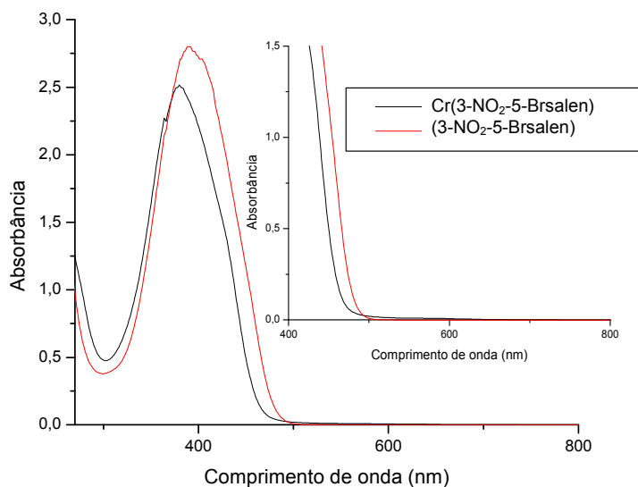
FIGURA B.10. Espectros eletrônicos na região do ultravioleta-visível para o ligante (3-NO 2 -5-Brsalen) e complexo Cr(3-NO 2 -5-Brsalen) em solvente DMSO concentração 1x 10 -4 mol L -1 , com expansão na região acima de 400 nm.
