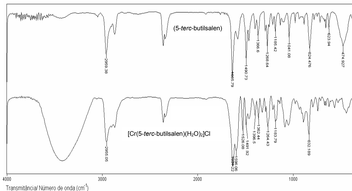
FIGURA A.4. Espectro na região do infravermelho do ligante (5-terc-butilsalen) e do complexo [Cr(5-terc-butilsalen)(H 2 O) 2 ]Cl, na região compreendida entre 4000 e 250 cm -1 , com resolução 4 cm -1 utilizando pastilhas de KBr (1 mg do composto para 100 mg de KBr) com as amostras do ligante e do complexo.
