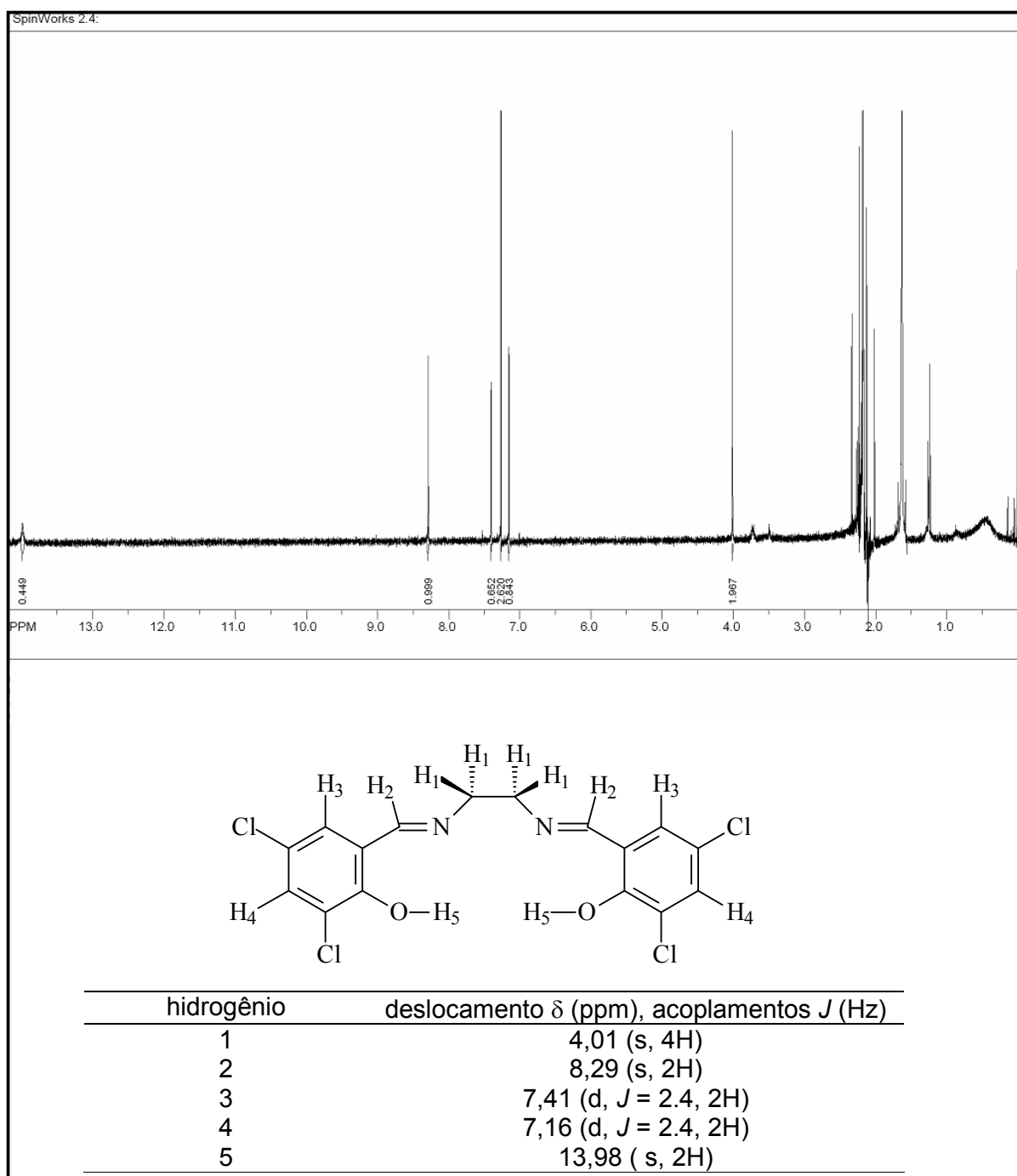
FIGURA D.5. Espectro ^1\text{H} RMN do ligante (3,5-DiClalen) utilizando como solvente \text{CDCl}_3 e como padrão interno TMS
