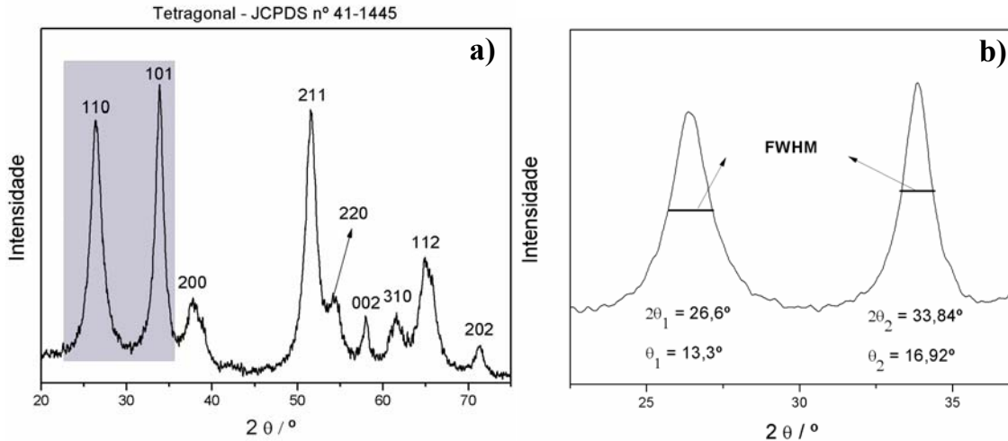
FIGURA 4.4 – (a) Padrão de difração de Raio X das nanopartículas de SnO 2 sintetizadas (área hachurada mostra os picos de difração que foram utilizados para se estimar a medida do tamanho de cristalito); (b) Em detalhe os picos de difração que foram utilizados com seus respectivos valores de \theta .
