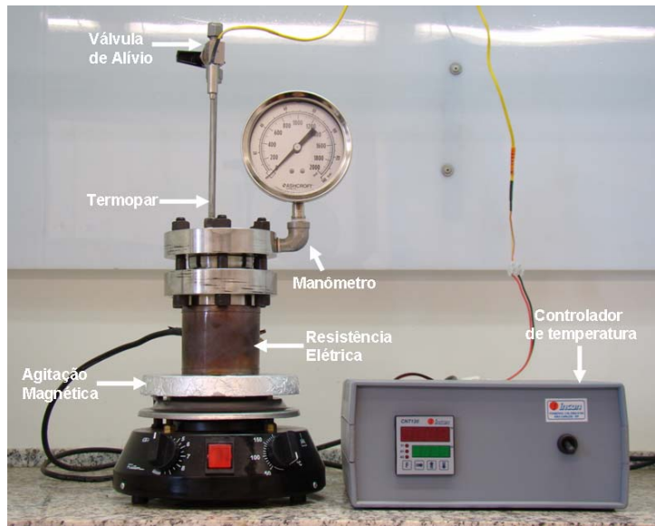
Figura 3.3 – Autoclave confeccionada para realização das sínteses de óxidos metálicos livre de haleto metálico como precursor ( ZrO_2 e In_2O_3:Sn ).
