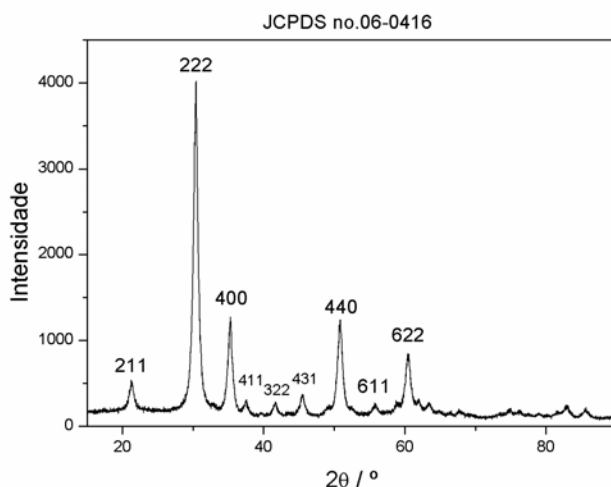
FIGURA 4.7 – Padrão de difração de Raio X das nanopartículas de ITO sintetizadas.
