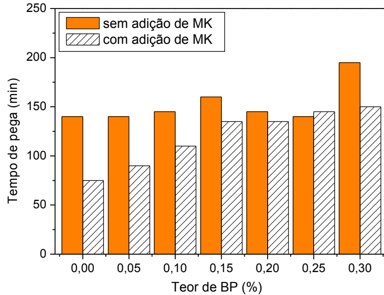
FIGURA 22: TEMPO DE PEGA POR PICO DE MÓDULO.
