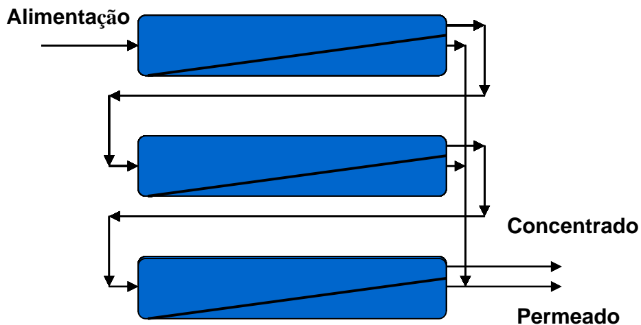
Figura 5.3.1: Arranjo com três elementos de membranas em série.
