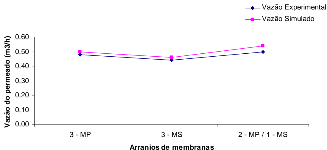
Figura 6.9 – Vazão do permeado em função dos arranjos dos elementos de membranas sem pré-tratamento químico
