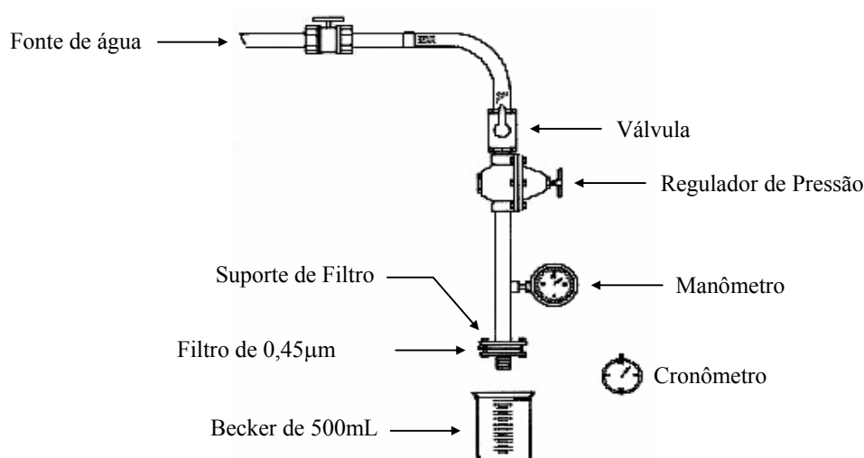
Figura 4.9.1: Equipamento básico para medição do IDS (AMJAD, 1992).
