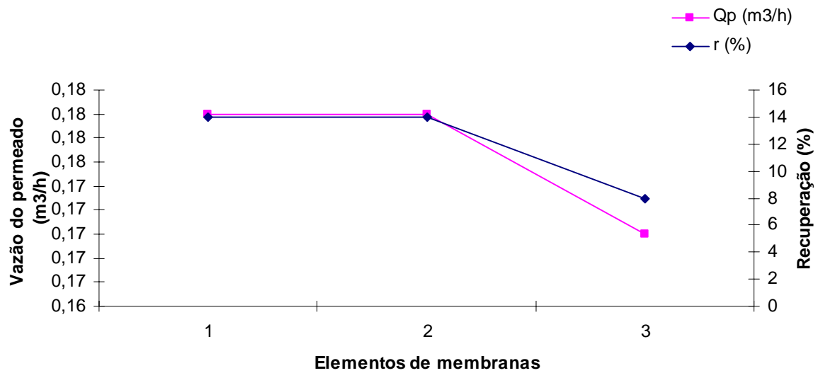
Figura 6.3 – Vazão do permeado e recuperação simulados para os elementos de membranas sem pré-tratamento químico
