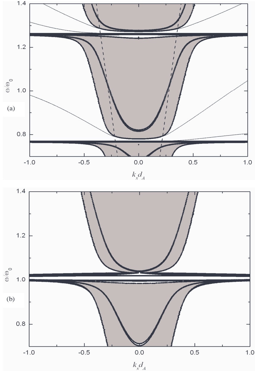
Figura 2.11: (a) Espectro de polariton, frequência reduzida \omega/\omega_0 versus k_x d_A , para a sexta seqüência da super-rede quasi-periódica de Fibonacci com \gamma H_0 = 13.5kG . (b) O mesmo de (a) com \gamma H_0 = 0kG .
