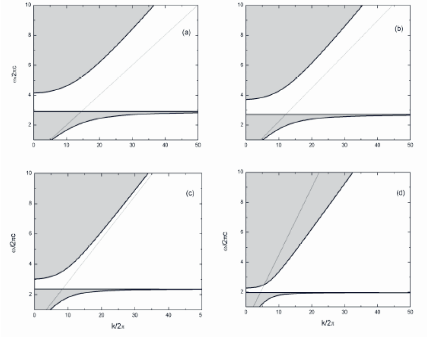
Figura 3.6: O mesmo da Fig. 3.5 para o metamagneto \text{FeCl}_2 .
