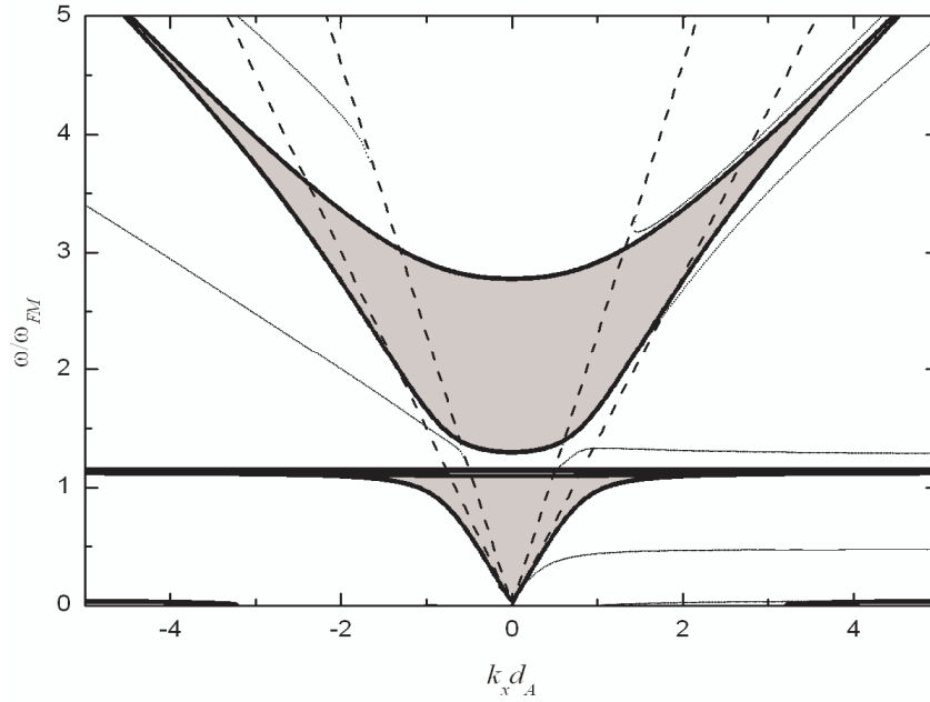
Figura 4.2: Espectro de polariton para o metamagneto \text{FeBr}_2 na sua fase FM (caso periódico).
