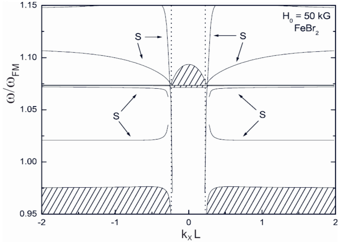
Figura 2.8: Relação de dispersão dos modos de polaritons magnéticos, volume (áreas sombreadas) e superfície (linhas contínuas), para o metamagneto \text{FeBr}_2 na sua fase FM como uma função do vetor de onda adimensional no plano k_x L . Consideramos um campo externo aplicado H_0 = 50kG , que é suficiente para superar o fraco acoplamento antiferromagnético intercamada.
