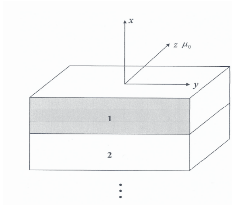
Figura 3.2: Geometria da super-rede periódica utilizada no problema onde o material (1) é ferromagnético e o material (2) não-magnético.
