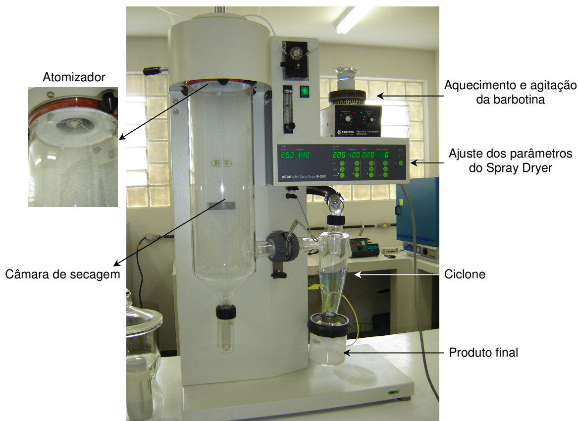
Figura 9 – Mini “Spray Dryer” utilizado para atomizar as suspensões varistoras (LIMAC – UEPG).]
