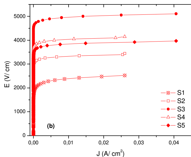
Figura 17 – Curva J \times E dos sistemas varistores de \text{SnO}_2 , sinterizados em 1350^\circ\text{C}/2\text{h} e compactados à verde em (a) 150 e (b) 200 MPa.
