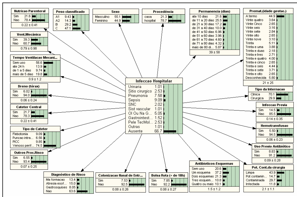
FIGURA 8 – APRESENTAÇÃO FINAL DE REDE BAYESIANA
