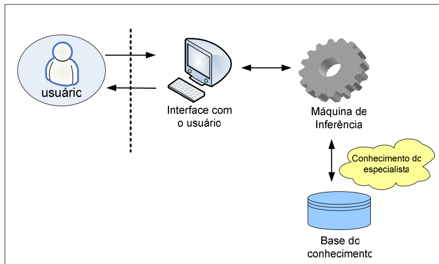
FIGURA 1 – ESTRUTURA CONVENCIONAL DE UM SISTEMA ESPECIALISTA
