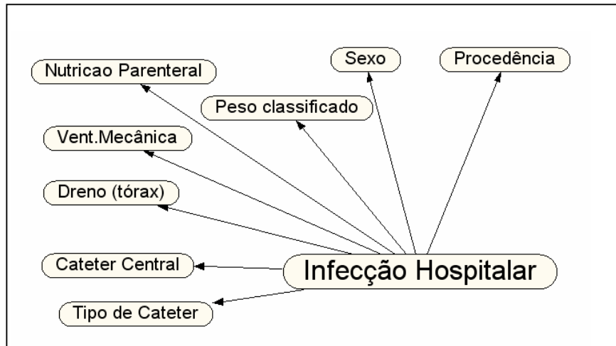
FIGURA 2 – EXEMPLO DA PARTE QUALITATIVA DE UMA REDE BAYESIANA
