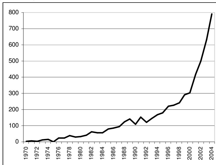
GRÁFICO 1 - NÚMERO DE ARTIGOS SOBRE TEOREMA DE BAYES EM REVISTAS MÉDICAS, PESQUISADOS NO MEDLINE ENTRE 1970 E 2004 (NCBI, 2005)
