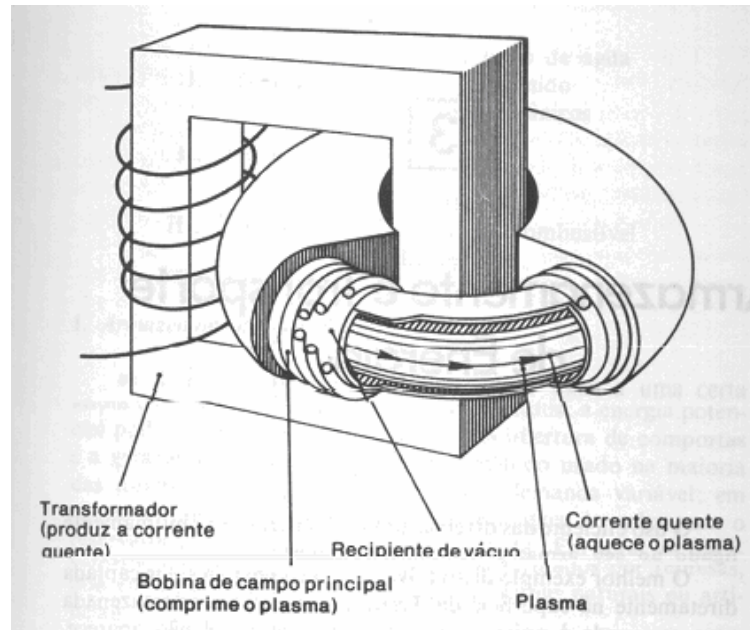
Figura 26: Esquema de um reator Tokamak, Goldemberg, (1979).
