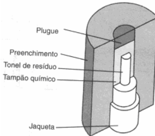
Figura 30: Contêiner para armazenagem de lixo nuclear, Hinrichs (2003).
