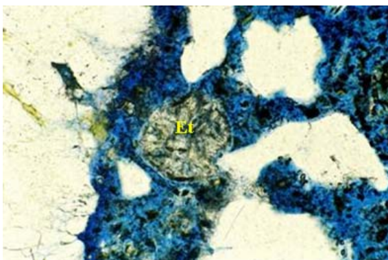
Figura 5.8 – Detalhe de um poro na borda do agregado graúdo preenchido por cristais de etringita (Et). Imagem obtida através de microscópio de luz transmitida com ampliação 100X.
