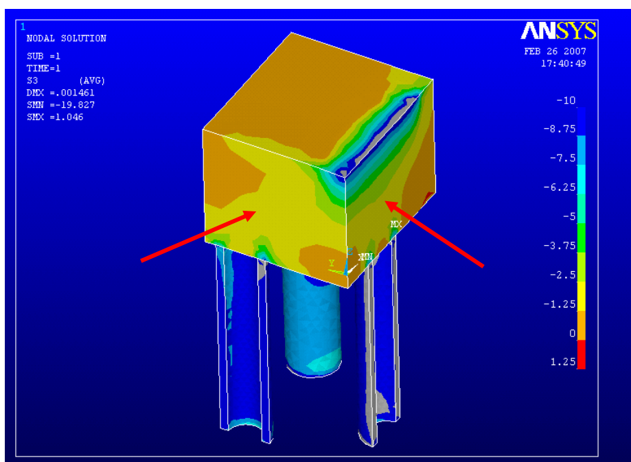
Figura 5.58 – Representação gráfica das tensões internas no bloco.
