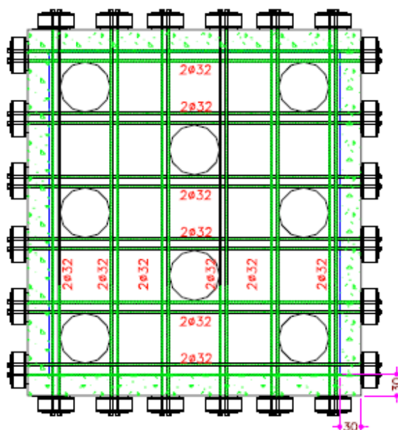
Figura 5.65 – Detalhe das barras DYWIDAG exercendo tensões de compressão no fundo do bloco.
