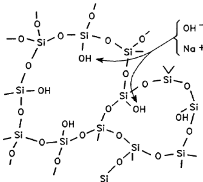
Figura 3.1 – Neutralização das ligações do grupo silanol pelas hidroxilas. Fonte: Hasparyk, 2005
