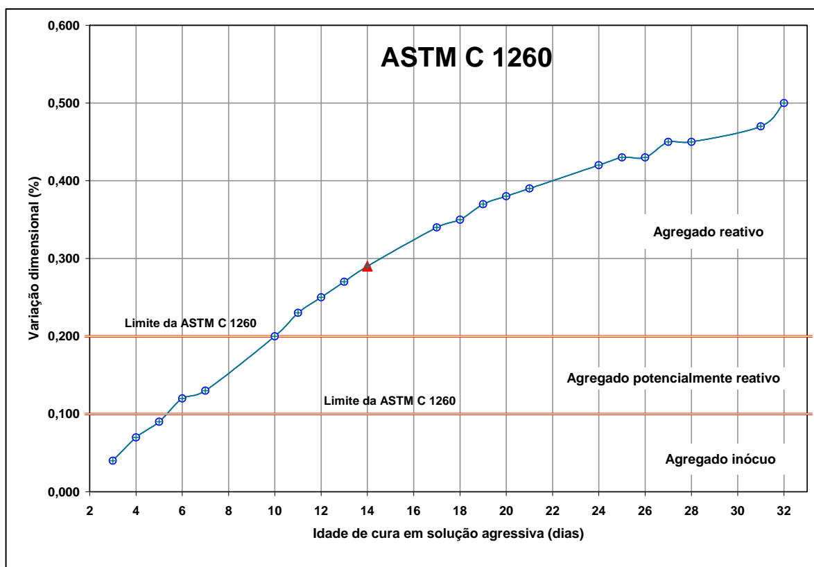
Figura 5.16 – Gráfico de expansão do agregado graúdo utilizado nos blocos de fundação. Fonte: Relatório de ensaio n° 36781 - ABCP
