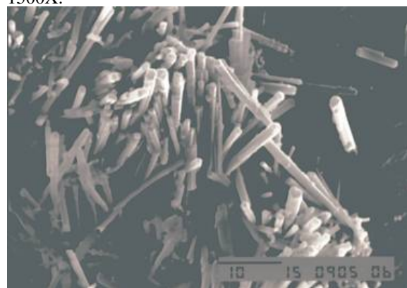
Figura 5.15 – Aspecto de detalhamento do agregado recoberto com cristais aciculares de etringita. Imagem obtida através de Microscópio Eletrônico de varredura.
