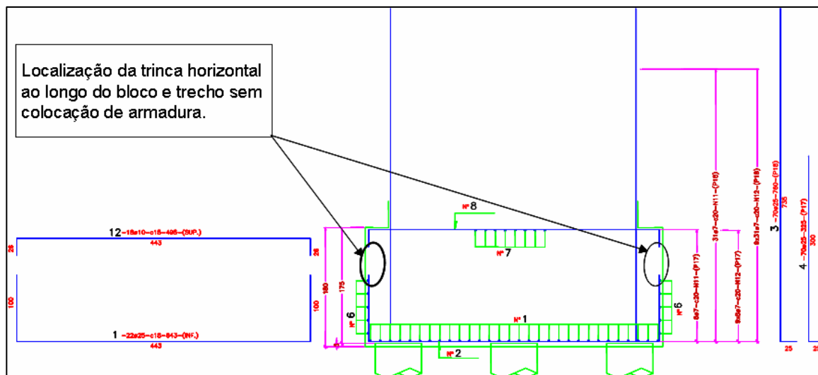
Figura 5.63 – Distribuição, posicionamento da armadura e localização da trinca horizontal de maior espessura.
