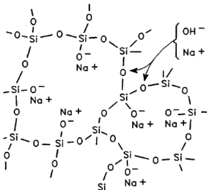
Figura 3.2 – Ruptura das ligações do grupo siloxano pelos íons hidroxilas Fonte: Hasparyk, 2005
