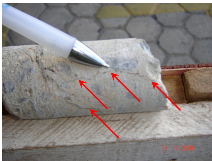
Figura 5.56 – Injeção do microcimento nas trincas finas.
