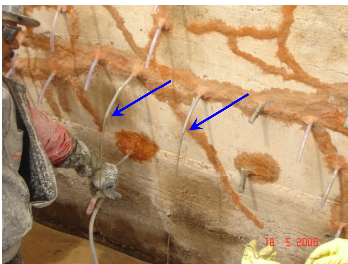
Figura 5.50 – Saída do microcimento pelos purgadores da trinca principal.
