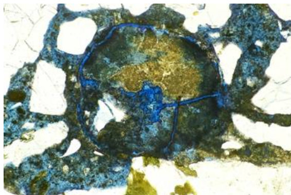
Figura 5.9 – Detalhe de um poro (P) na borda do agregado (A) preenchido por gel típico da RAA. Imagem obtida através de microscópio de luz transmitida com ampliação 100X.
