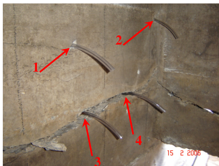
Figura 5.25 – Colocação dos purgadores nas trincas e nos furos.
