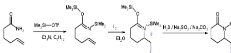
Figura 4.2 – Reação de iodolactamização.
