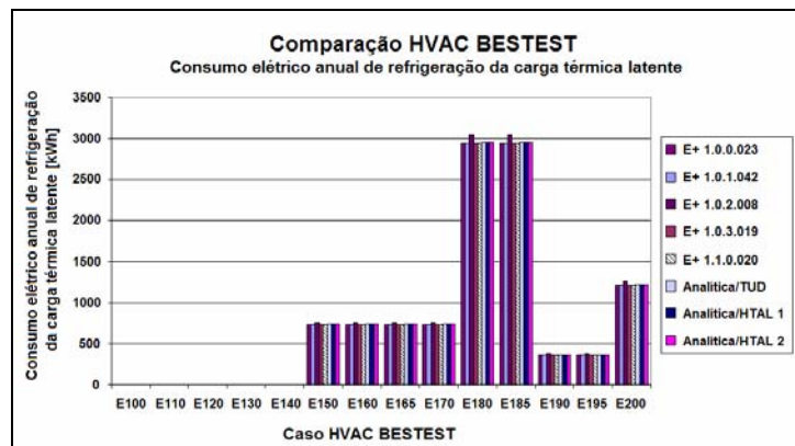
Figura 2.8. HVAC BESTEST – Consumo anual de refrigeração da carga térmica latente.
