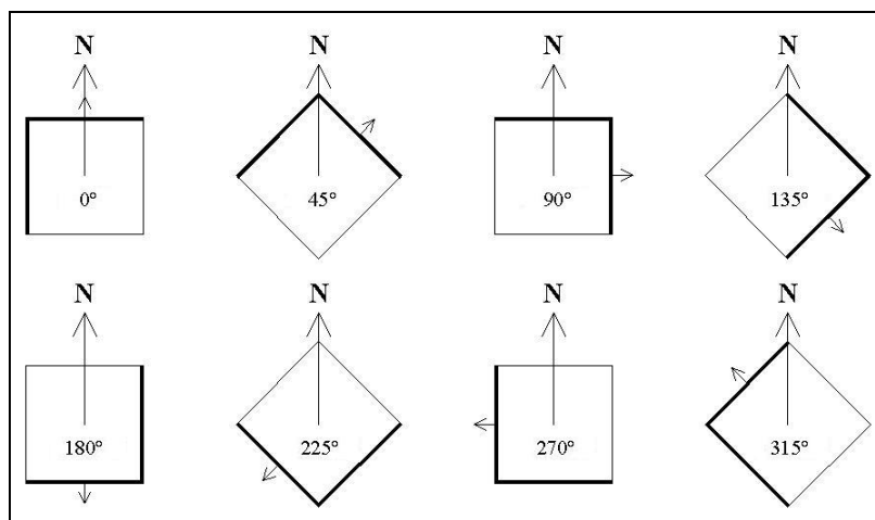
Figura 5.5. Vista superior representando a edificação e mostrando as orientações simuladas.
