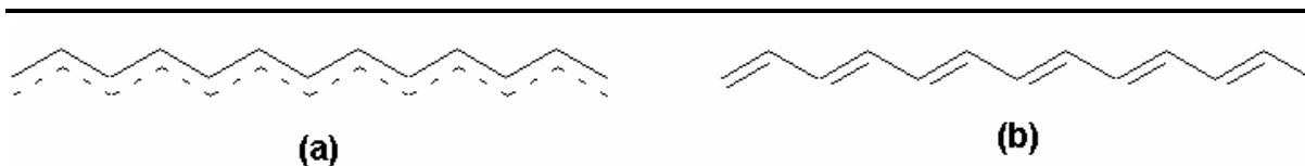
Figura 3 – Poliacetileno. a) estrutura de ressonância; b) estrutura trans “não-ressonante” ou “dimerizada”.
