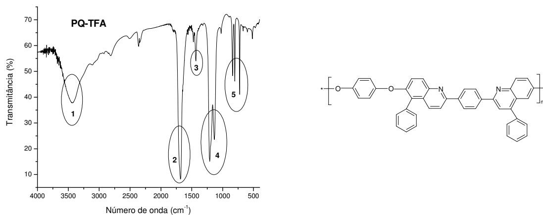
Figura 26 – Espectros de FTIR do copolímero em pastilha de KBr.
