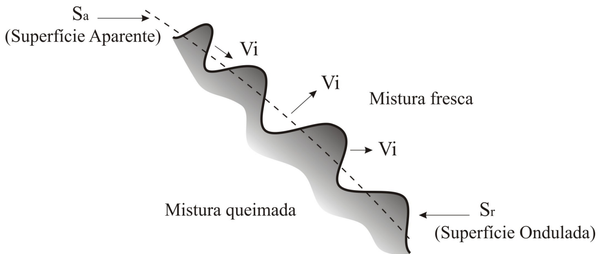
Figura 3.5: Modelo de frente de chama enrugada
