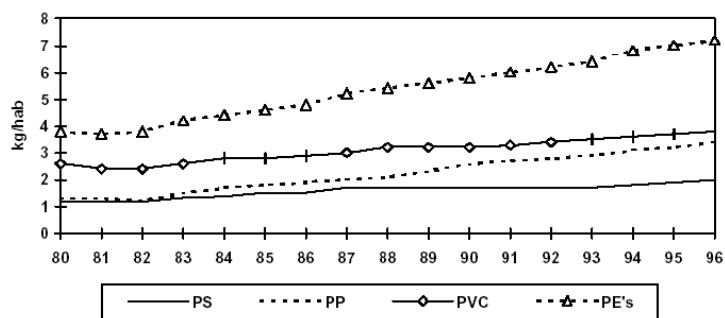
Figura 2.2: Evolução da demanda per capita mundial para o poliestireno, PS, polipropileno, PP, poli(cloreto de vinila), PVC e polietilenos, PE (1980-1996).
