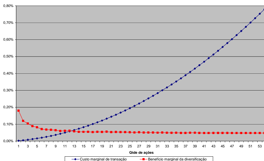
Gráfico 1: Equilíbrio de mercado. Grau ideal de diversificação de uma carteira.
